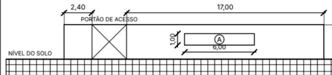
ELEVAÇÃO TAPUME
