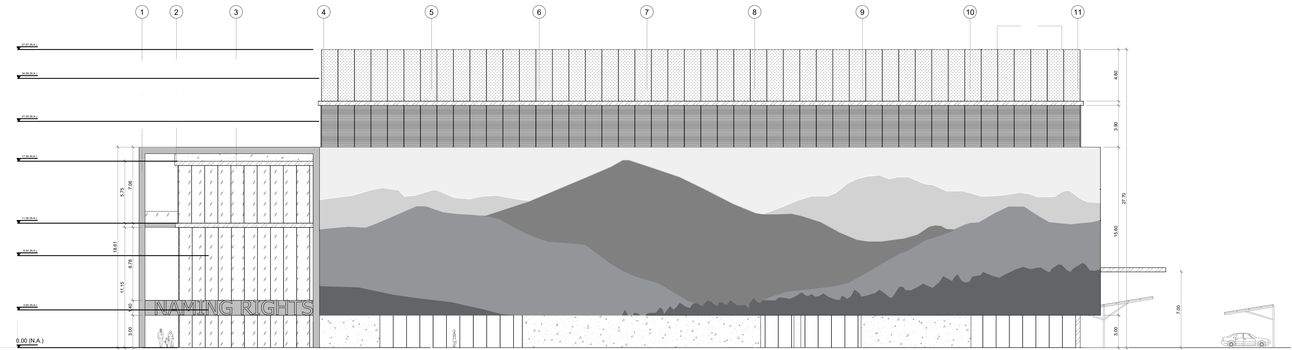
FACHADA PRINCIPAL - AV. EDGAR NELSON MEISTER ESCALA 1:200
