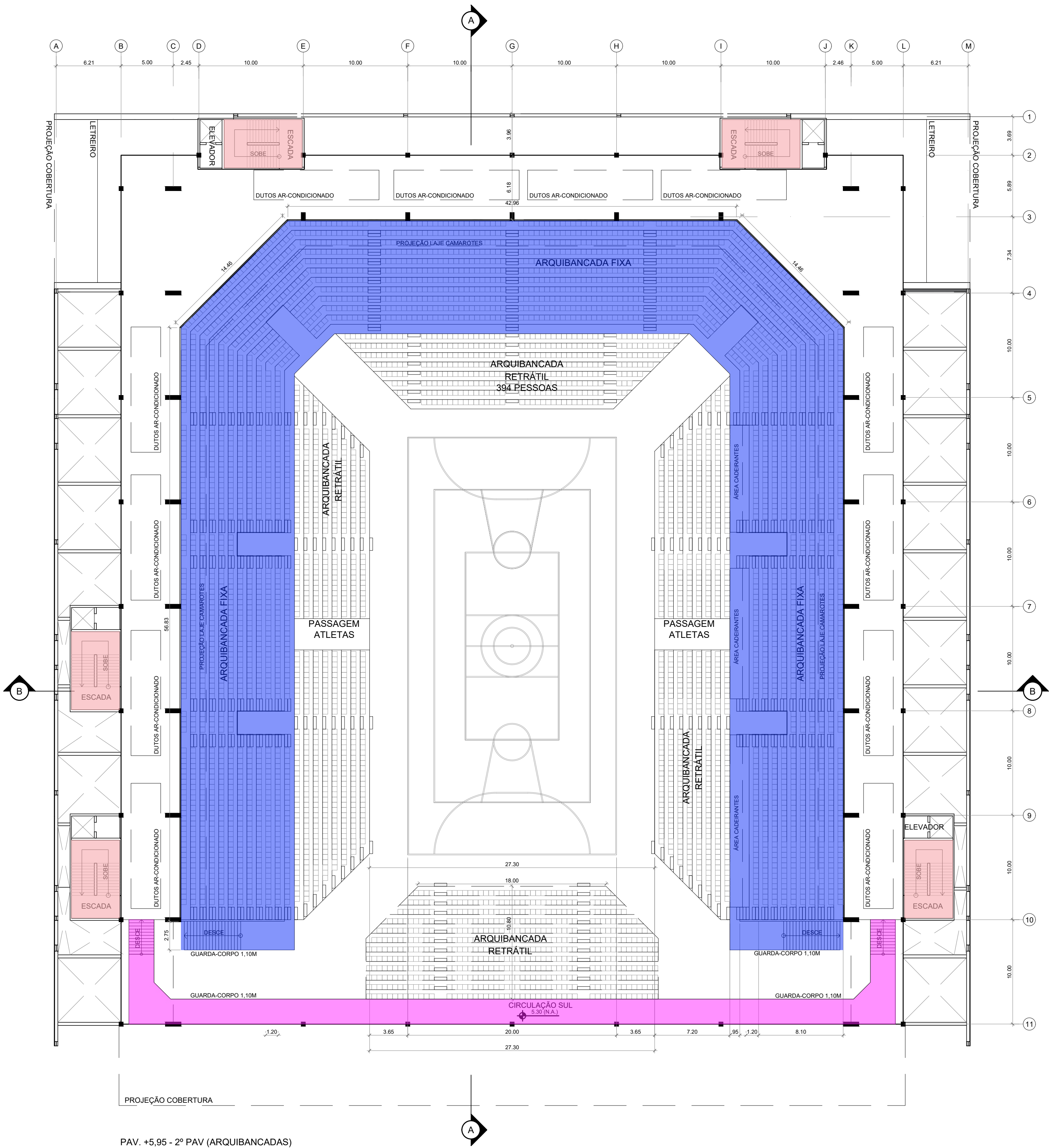
PAV. +5,95 - 2º PAV (ARQUIBANCADAS) ESCALA 1:250
