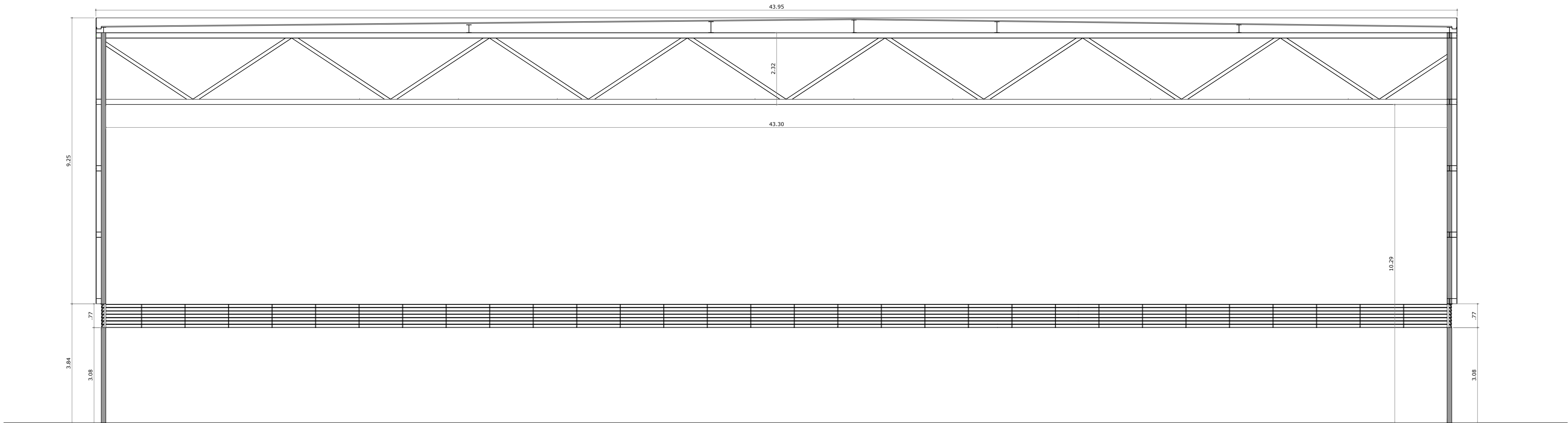
CORTE CC - CENTRO DE TREINAMENTO ESCALA 1:100
