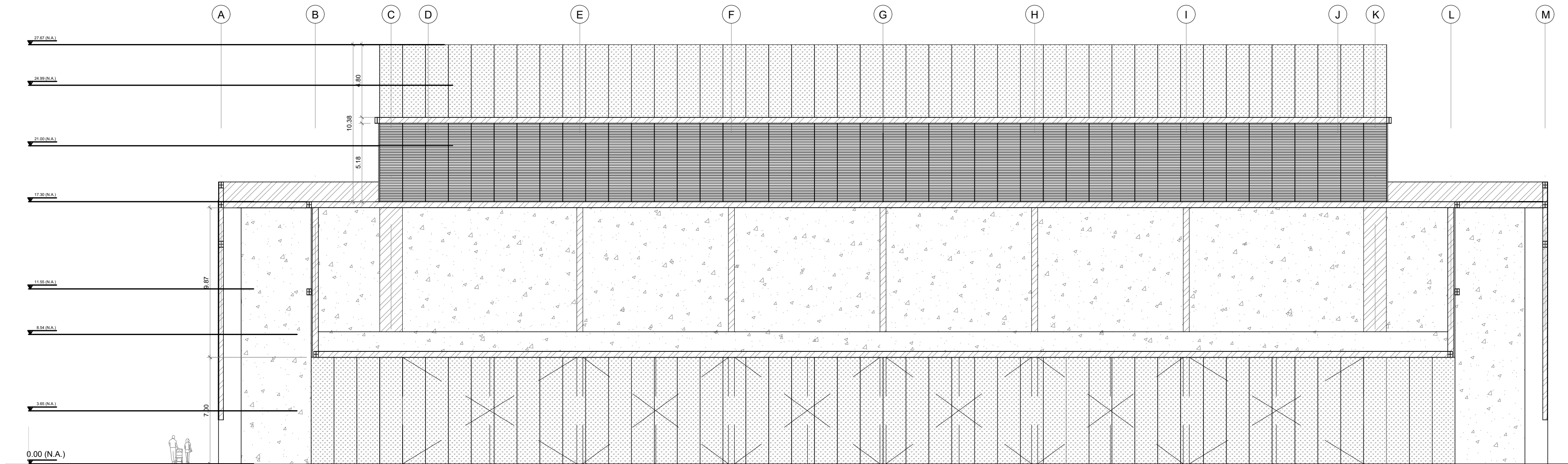
FACHADA LATERAL - SERVIÇO CARGA E DESCARGA ESCALA 1:200
