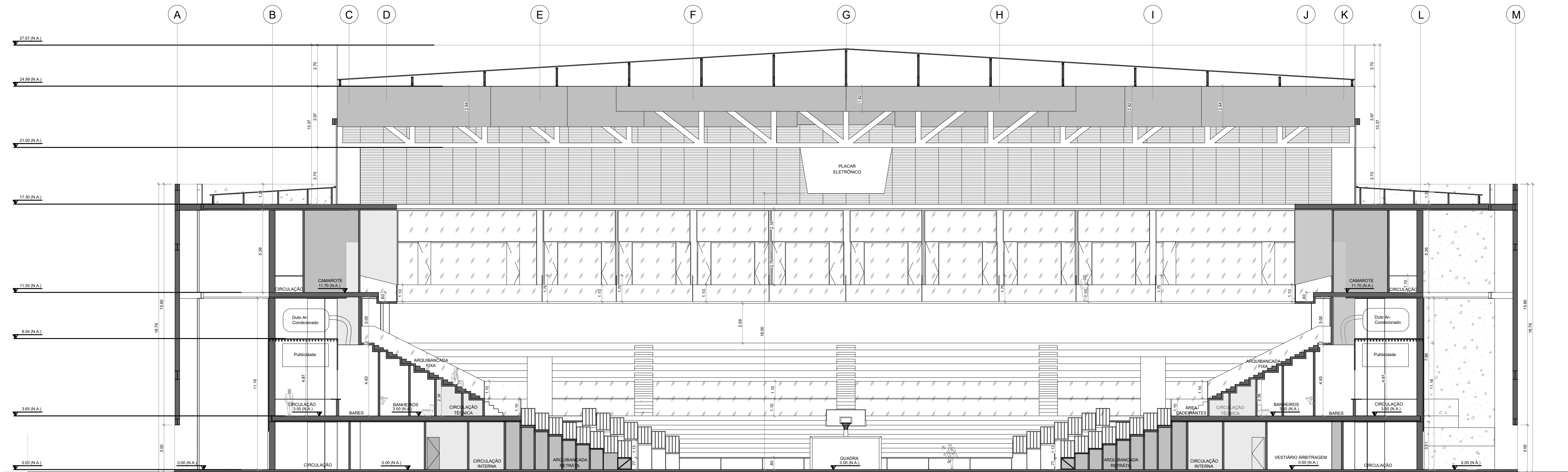
CORTE BB - TRANSVERSAL ESCALA 1:150
