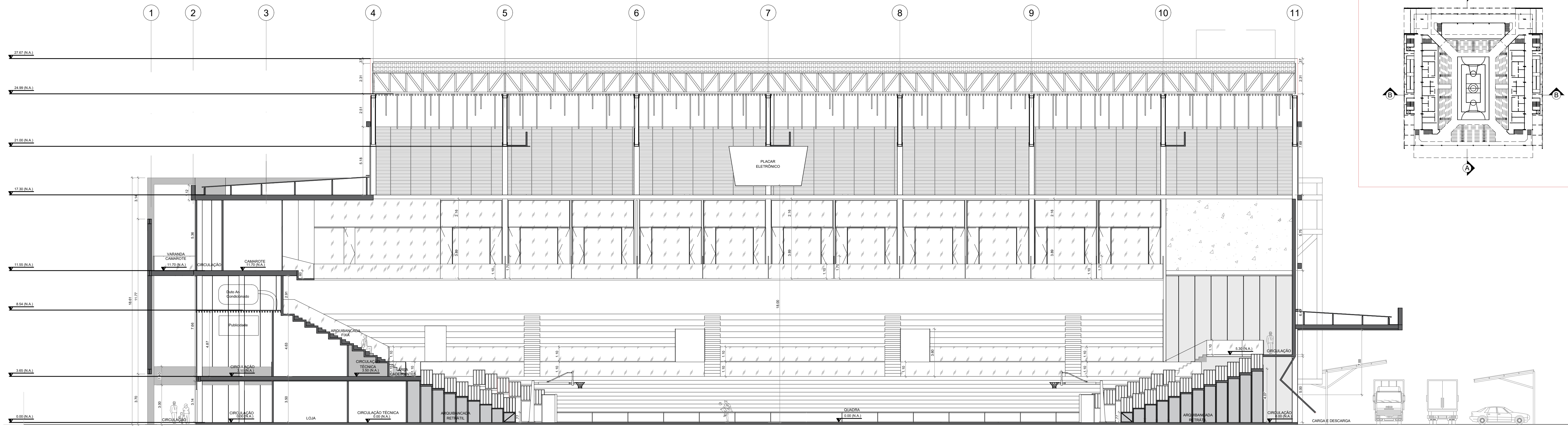
CORTE AA - LONGITUDINAL ESCALA 1:150
