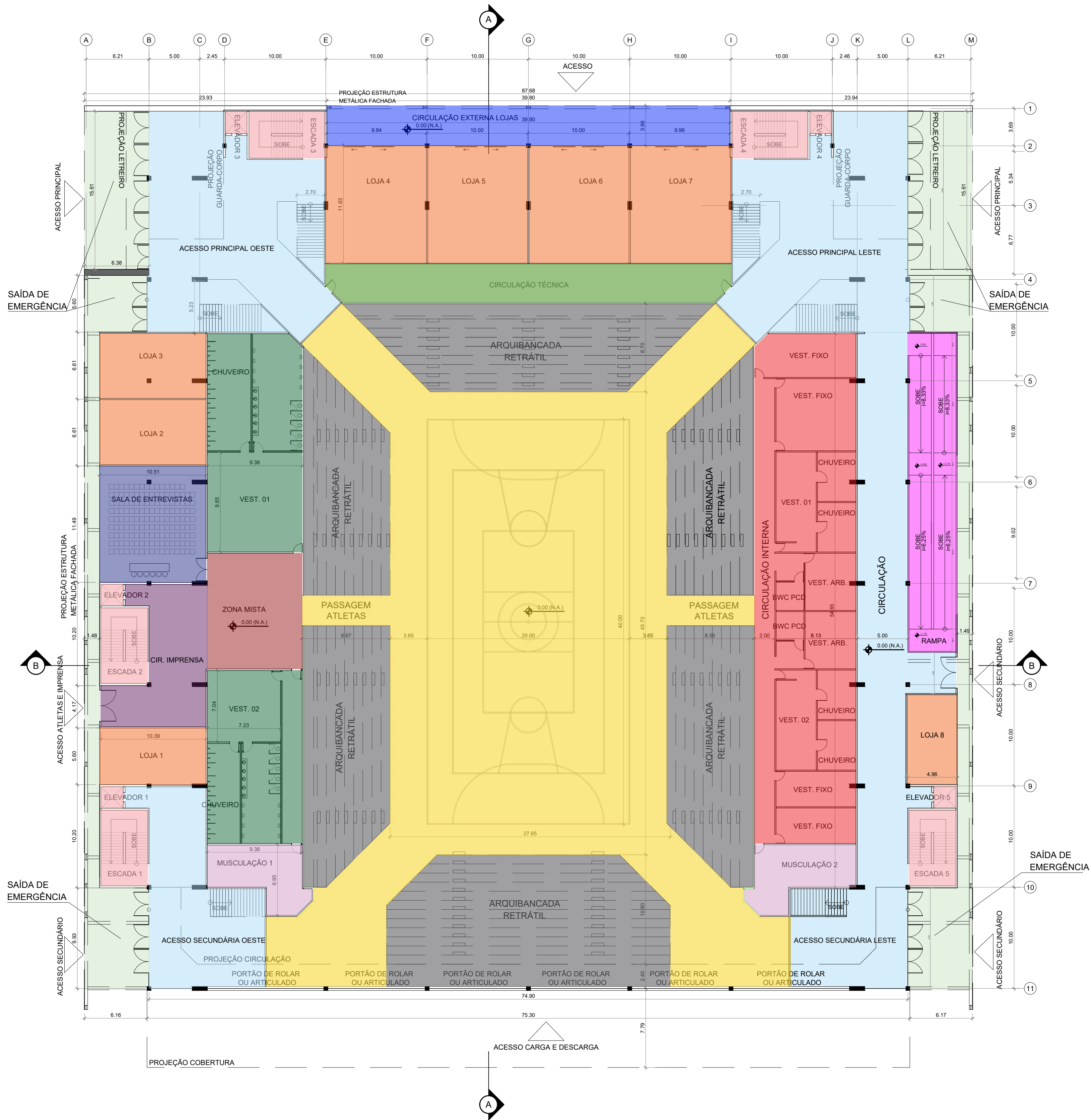
PAV. TÉRREO ESCALA 1:250
