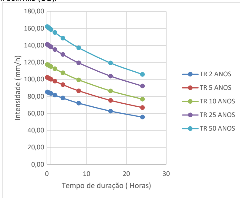
Figura 3.3.2.2-2. Correlação Intensidade-Tempo de duração das chuvas em Joinville (SC).
