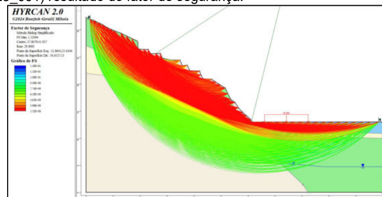
Figura 3.3.1.2-2. Exemplo de modelo de estabilidade de talude (perfil 023_001) resultado do fator de segurança.
