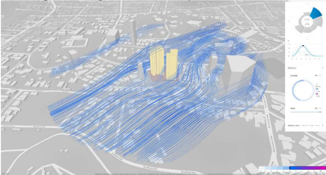
Figura 26 - Modelagem Aerodinâmica com empreendimento - Vento Nordeste
