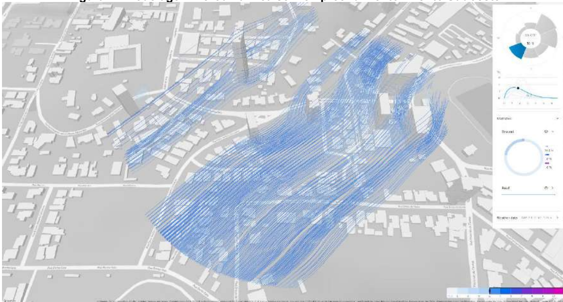
Figura 24 Modelagem Aerodinâmica sem empreendimento - Vento Sudoeste
