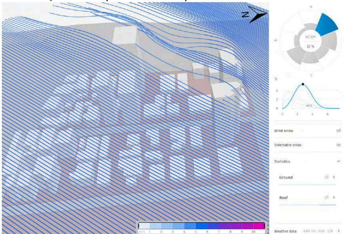
Figura 37. Simulação de ventos predominantes em quadras sentido Nordeste - altura de 35 metros
