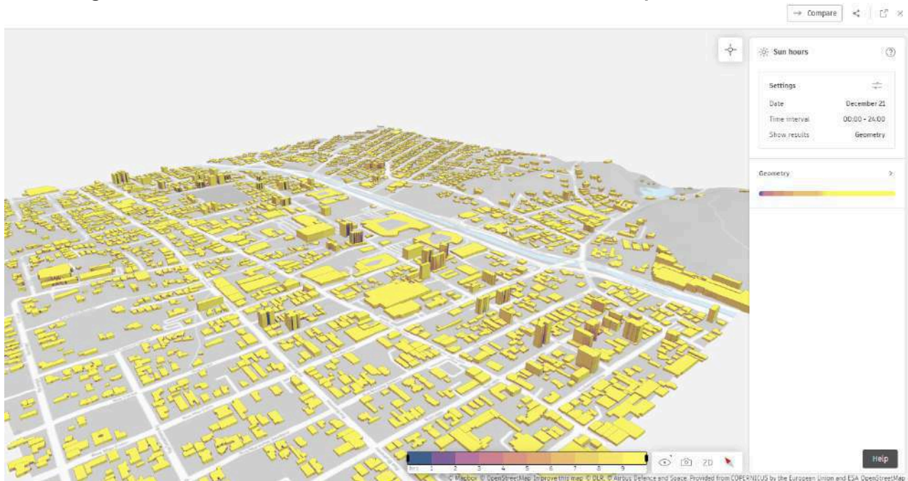
Figura 61. Simulação de incidência solar no solstício de verão, porção norte da OUC
