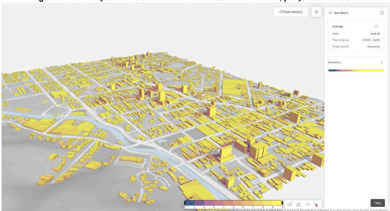
Figura 54. Simulação de incidência solar no solstício de inverno, porção sul da OUC
