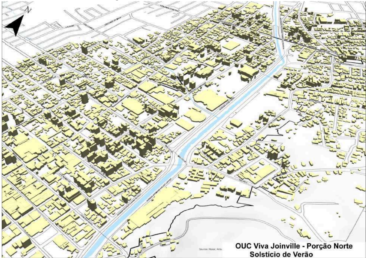
Figura 57. Simulação de sombreamentos
