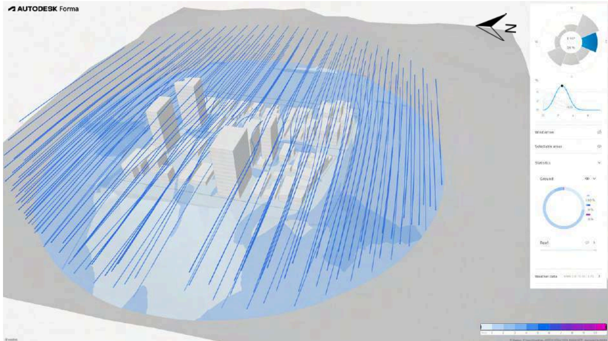
Figura 41. Simulação de ventos predominantes em quadras sentido Leste - altura variada de ventilação
