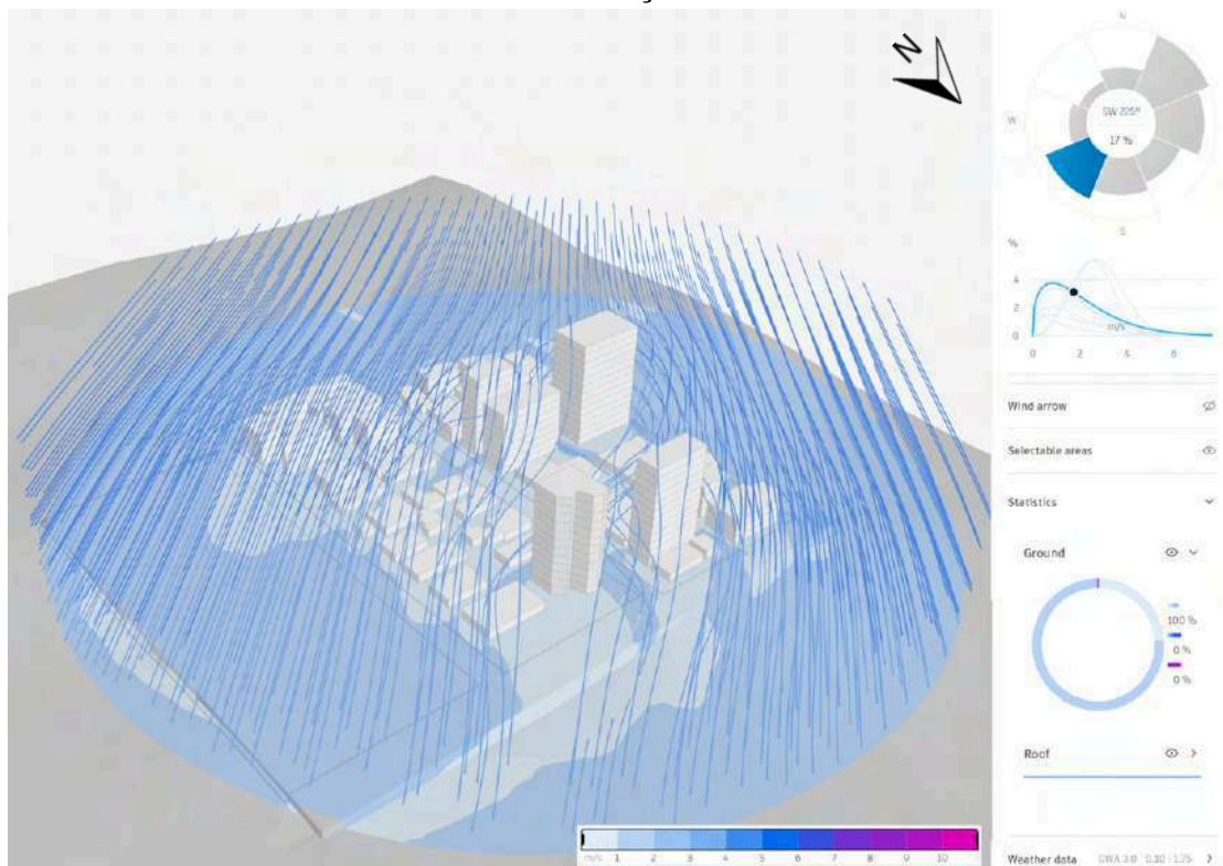
Figura 44. Simulação de ventos predominantes em quadras sentido Sudoeste - altura variada de ventilação
