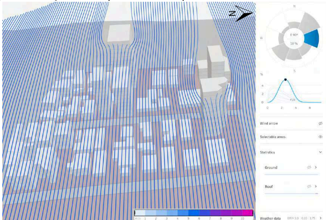
Figura 40. Simulação de ventos predominantes em quadras sentido Leste - altura de 35 metros
