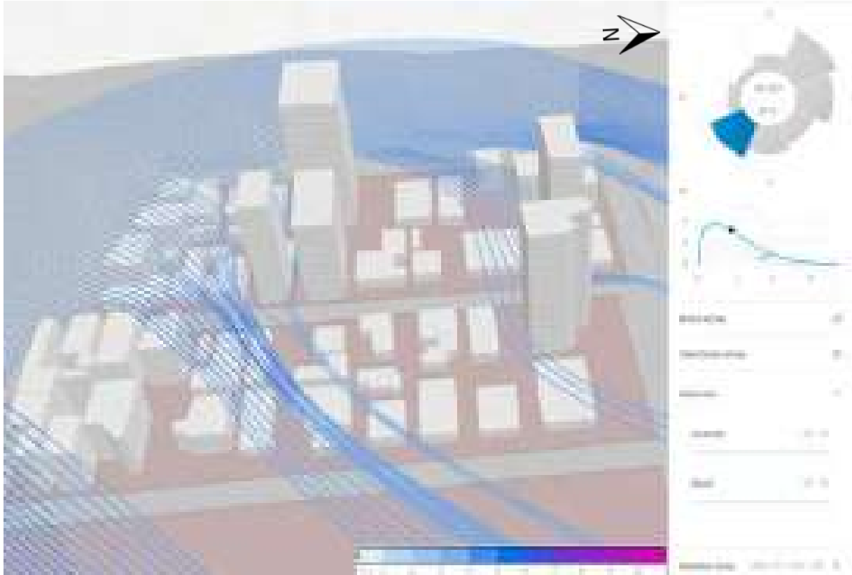
Figura 42. Simulação de ventos predominantes em quadras sentido Sudoeste - altura de 12 metros
