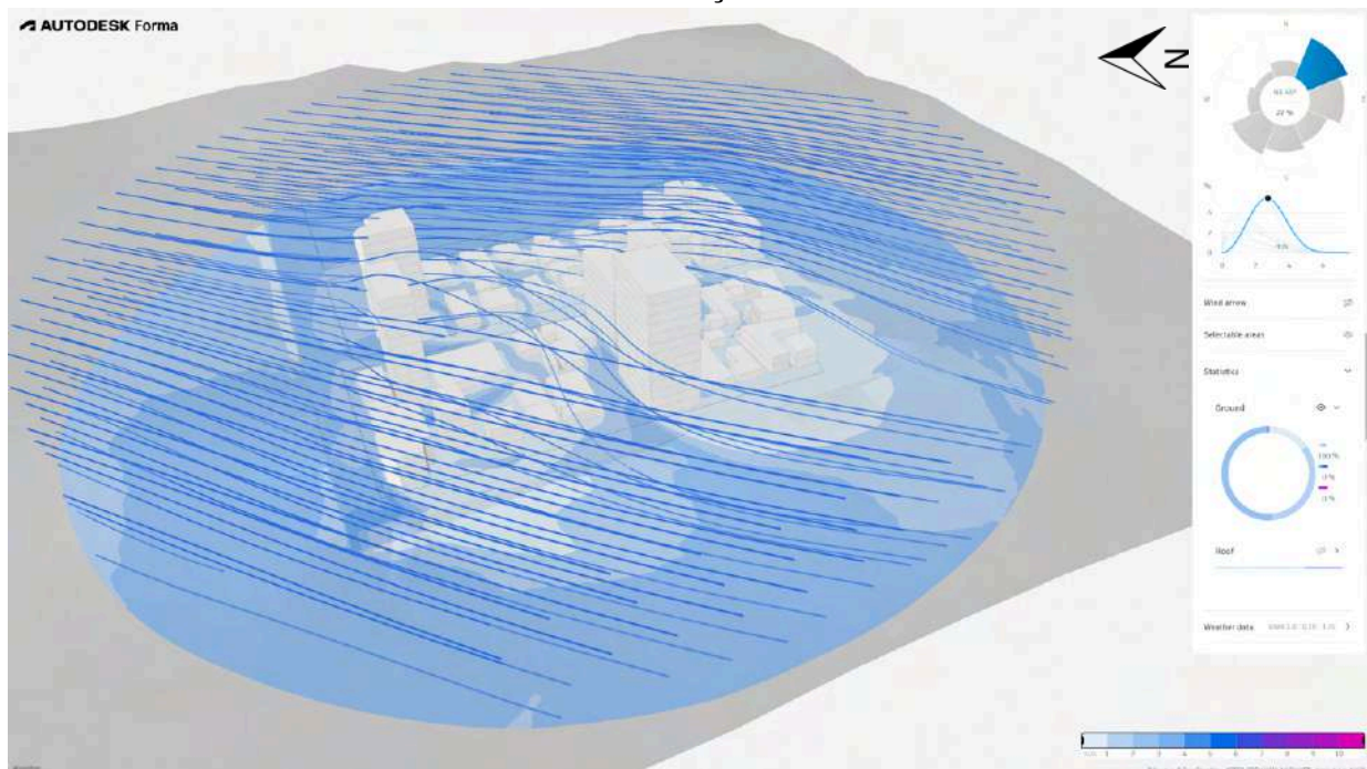
Figura 38. Simulação de ventos predominantes em quadras sentido Nordeste - altura variada de ventilação
