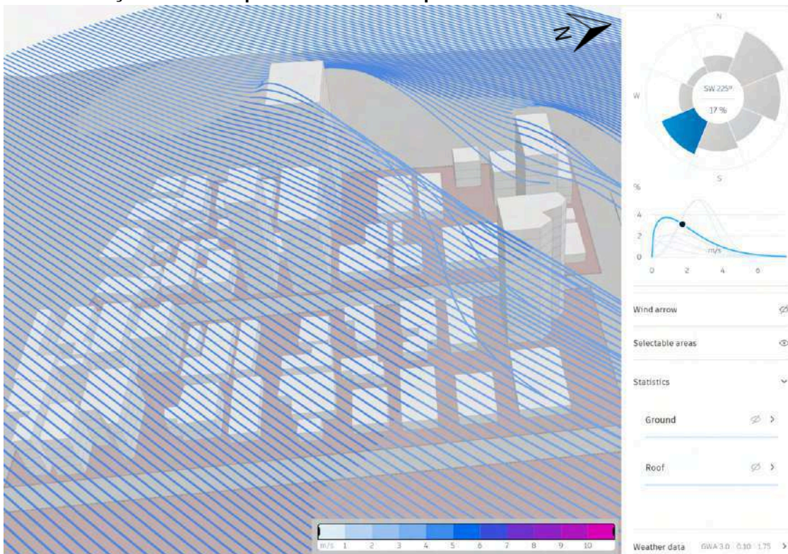
Figura 43. Simulação de ventos predominantes em quadras sentido Sudoeste - altura de 35 metros
