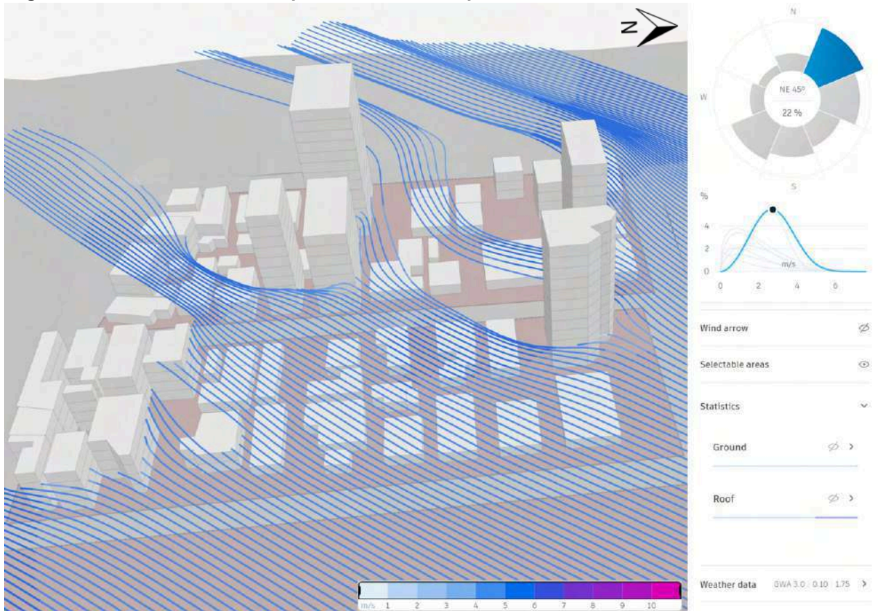
Figura 36. Simulação de ventos predominantes em quadras sentido Nordeste - altura de 12 metros
