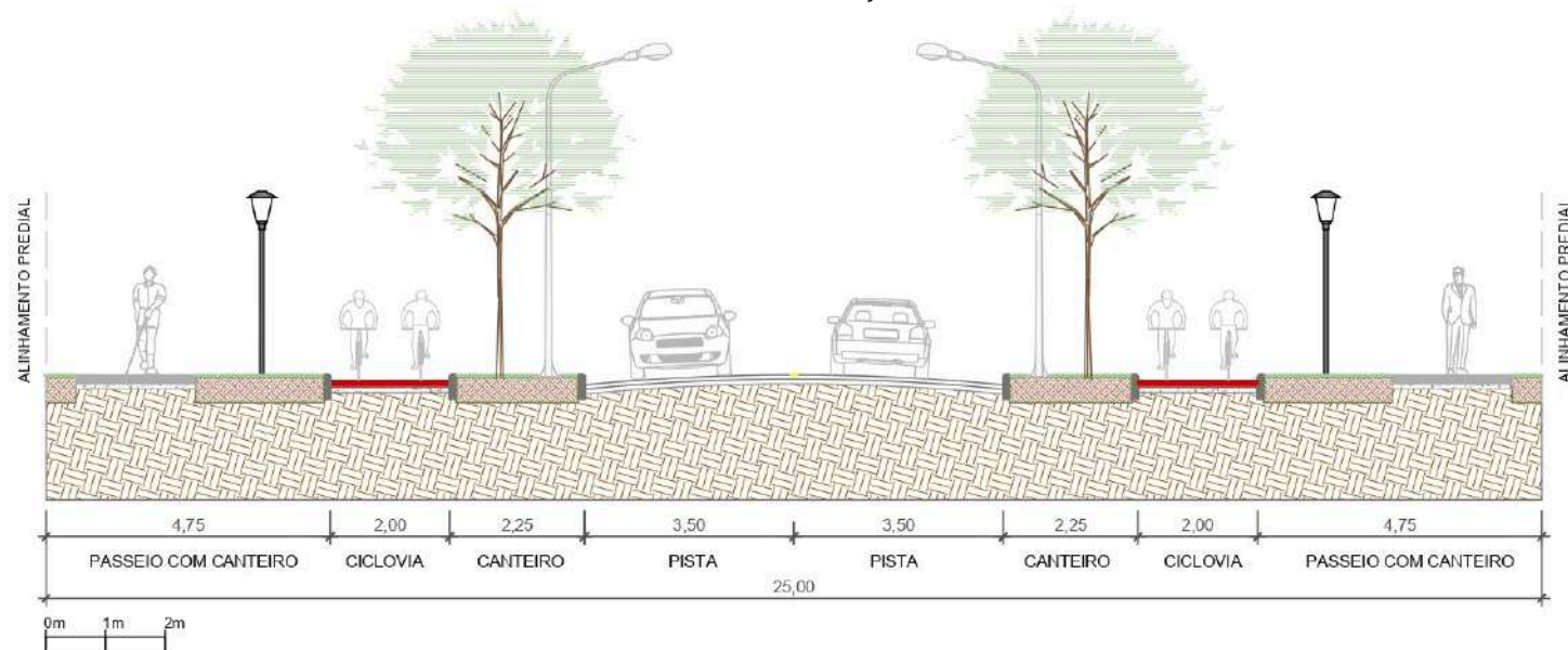
Boulevard Vale Verde - Seção de 25 m
