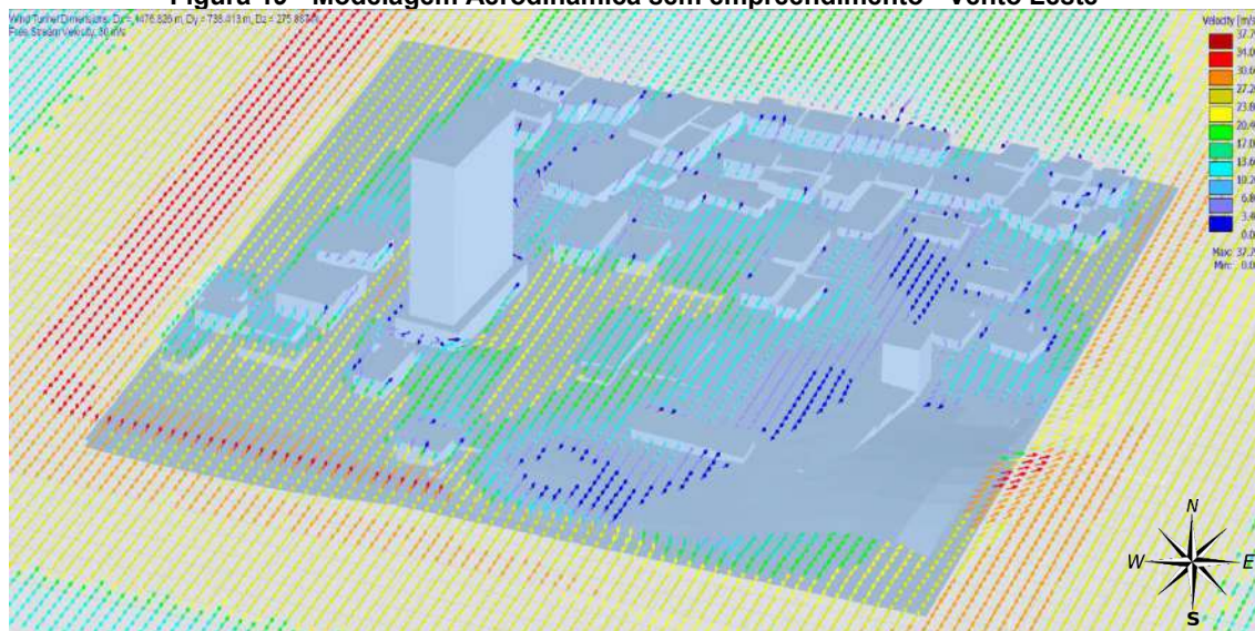
Figura 19 - Modelagem Aerodinâmica sem empreendimento - Vento Leste
