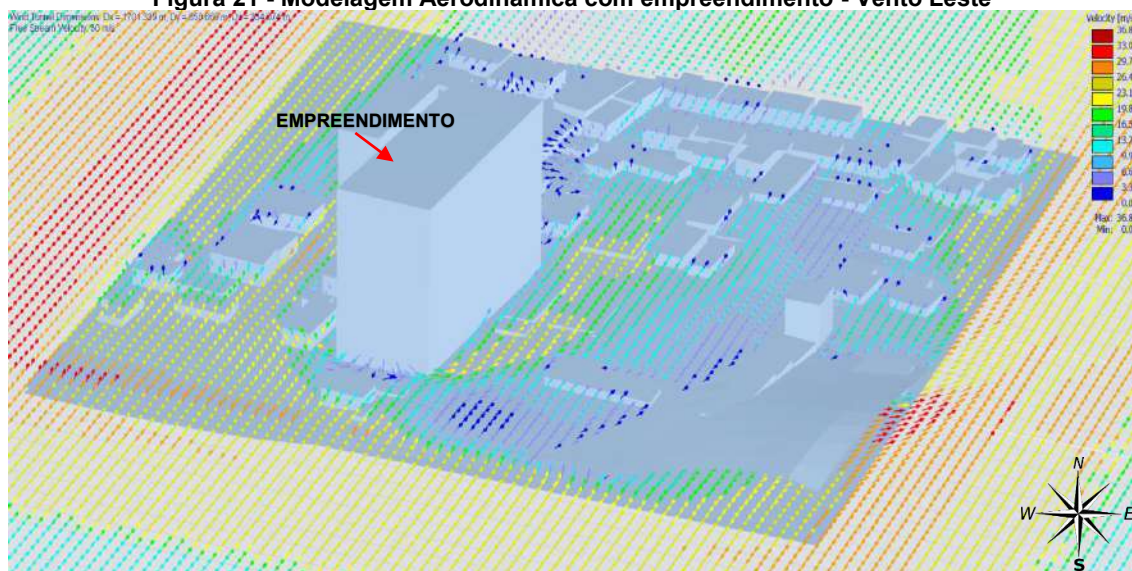
Figura 21 - Modelagem Aerodinâmica com empreendimento - Vento Leste
