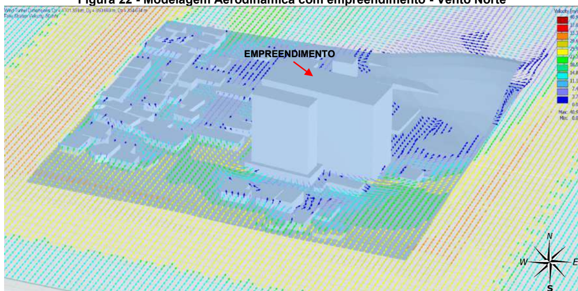
Figura 22 - Modelagem Aerodinâmica com empreendimento - Vento Norte
