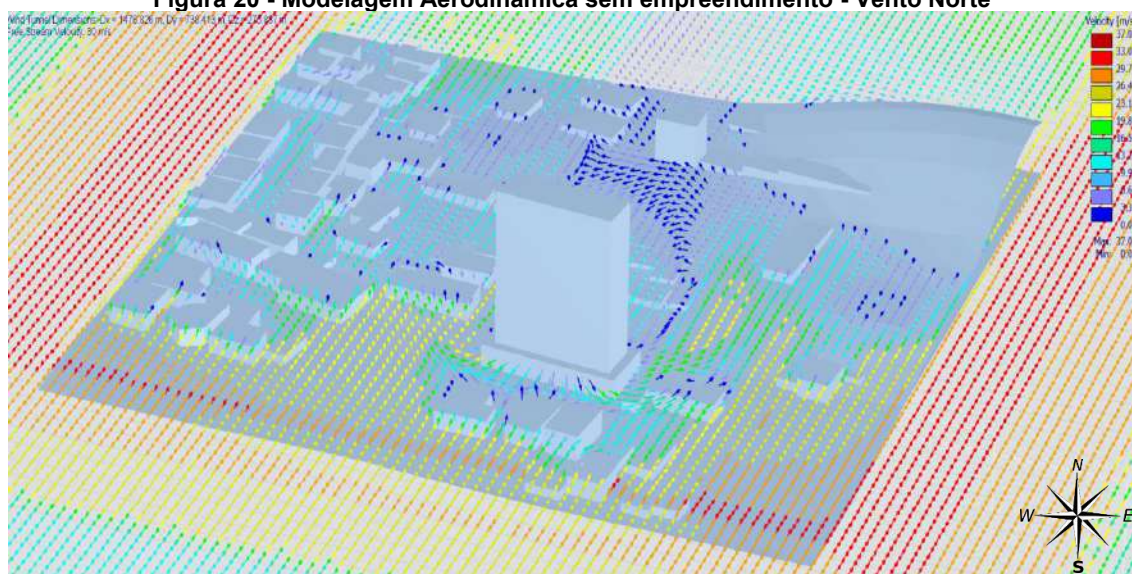
Figura 20 - Modelagem Aerodinâmica sem empreendimento - Vento Norte
