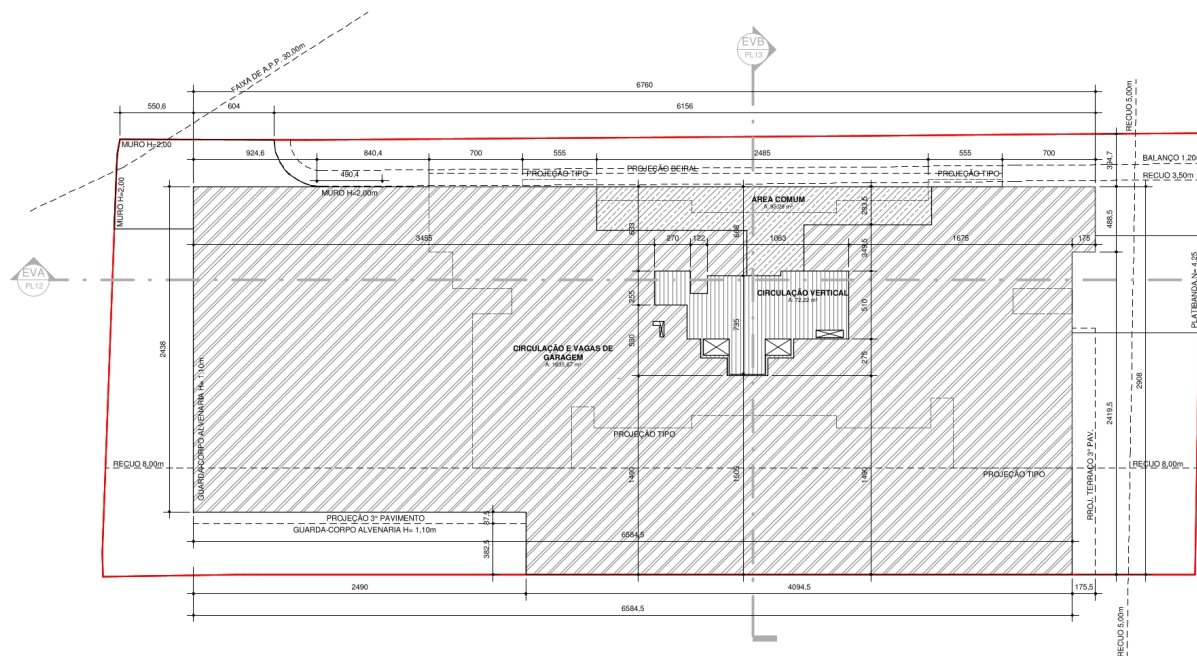
PLANTA ESQUEMÁTICA 2º PAVIMENTO
