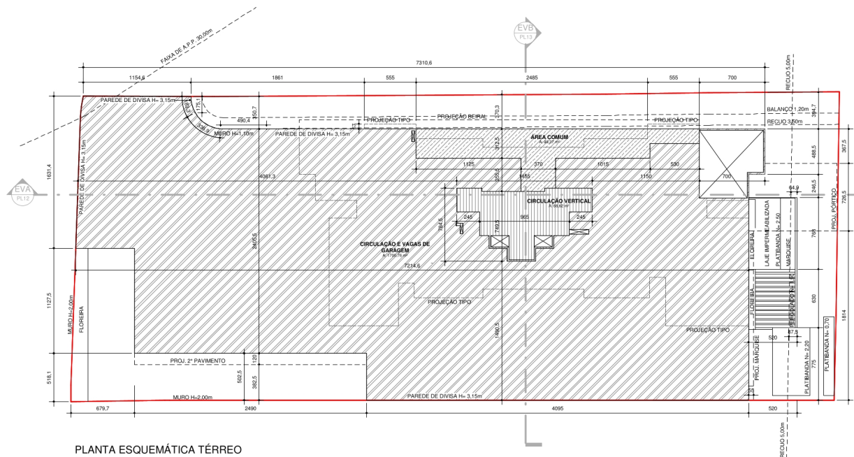
PLANTA ESQUEMÁTICA TÉRREO
