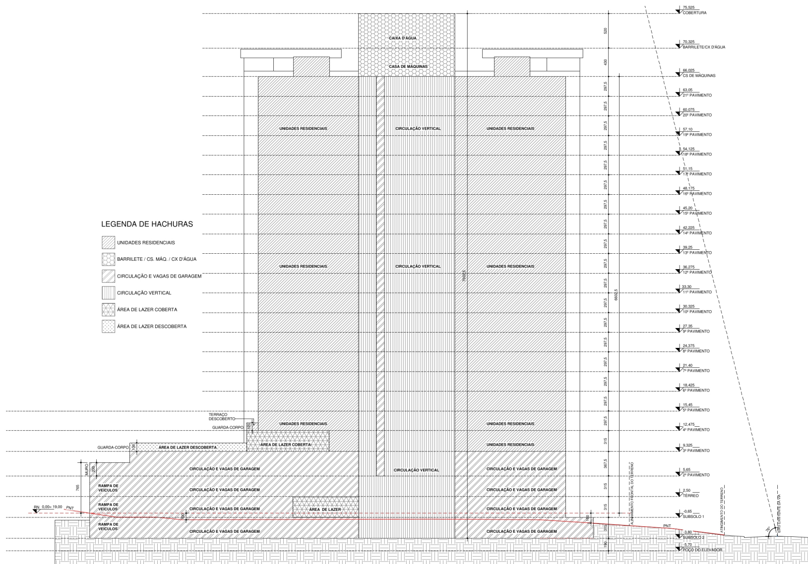
ESQUEMA VERTICAL AA ESCALA 1 : 200
