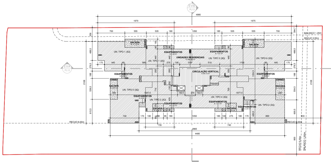
PLANTA ESQUEMÁTICA PAVIMENTO TIPO A (5º - 17º) ESCALA 1:200
