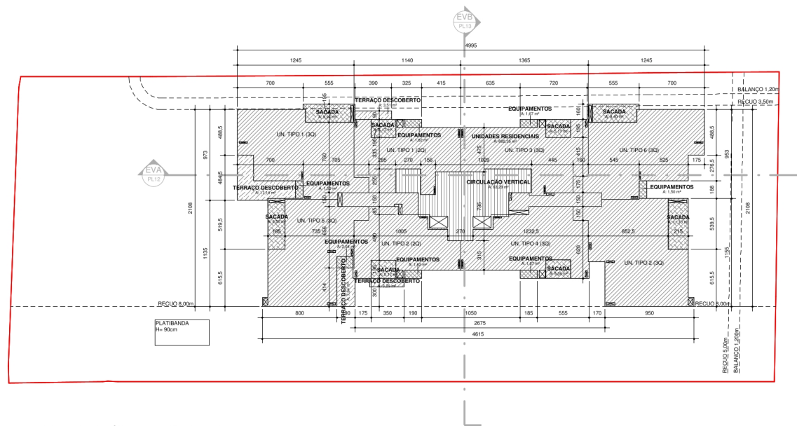
PLANTA ESQUEMÁTICA 4º PAVIMENTO ESCALA 1 : 200
