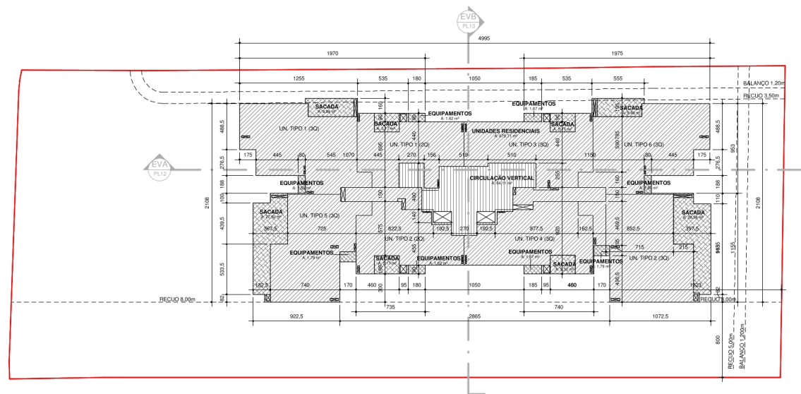
PLANTA ESQUEMÁTICA PAVIMENTO TIPO B (18° - 21°) ESCALA 1:200
