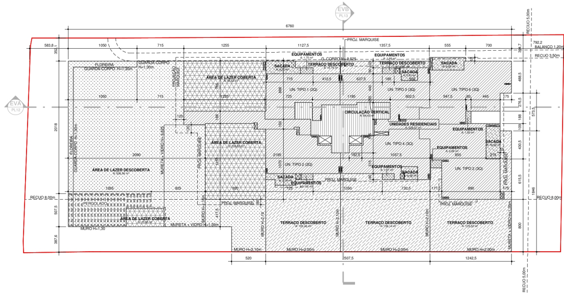
PLANTA ESQUEMÁTICA 3º PAVIMENTO ESCALA 1 : 200
