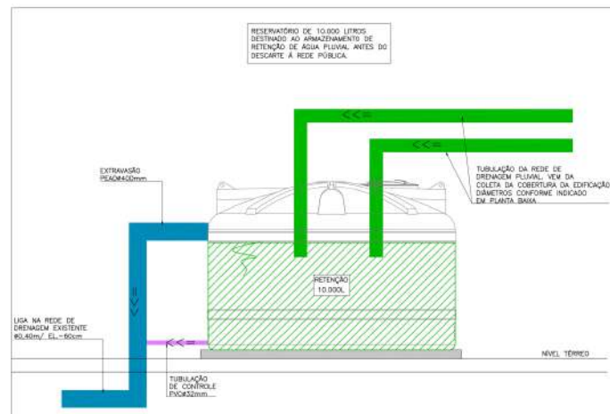
DETALHE CONJUNTO 02 DE RESERVATÓRIOS DE RETENÇÃO PLUVIAL (10.000 LITROS) SEM ESCALA
