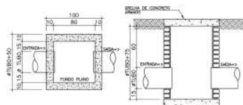
DETALHE CAIXA DE AREIA - CA SEM ESCALA
