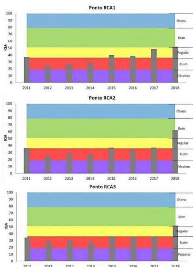
Figura 31: IQA médio de 2011 até 2018 nos pontos de monitoramento do Rio Cachoeira. Fonte: CCJ, 2022.
