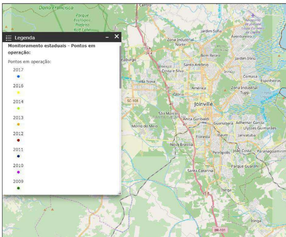
Figura 29: Mapa de Joinville disponibilizado pela Agência Nacional de Águas (ANA), com relação as estações de monitoramento da qualidade da água. A ausência dos pontos informados na legenda demonstra a inexistência deste monitoramento até 2017. Fonte: Agência Nacional de Águas (ANA), 2021.
