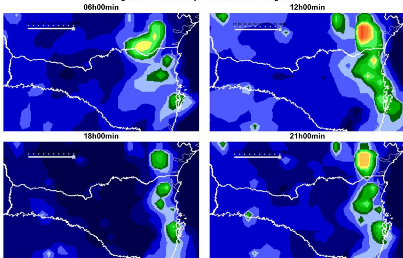
Figura 20 - Concentração de óxidos de nitrogênio
