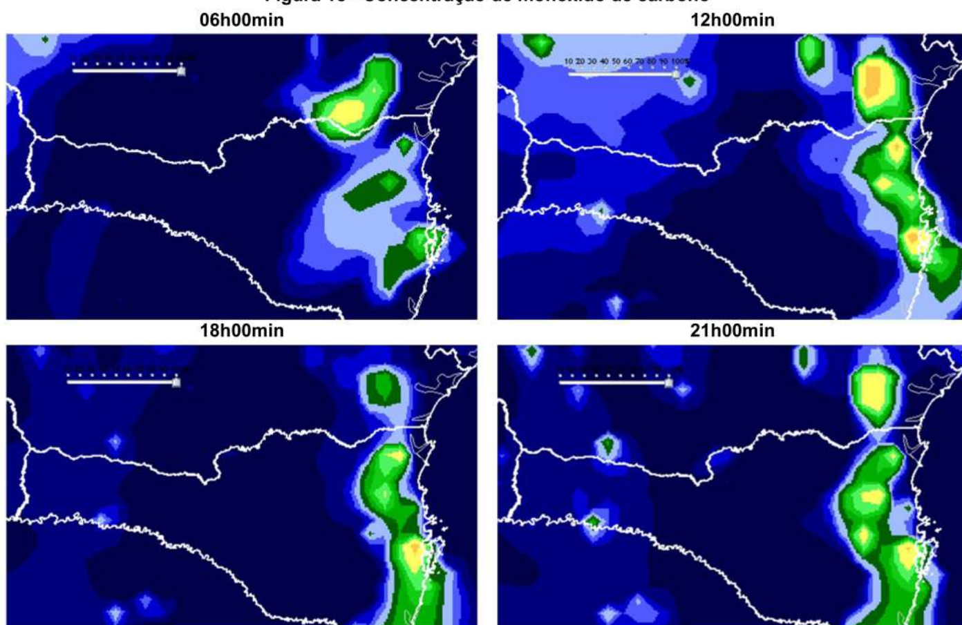
Figura 18 - Concentração de monóxido de carbono
