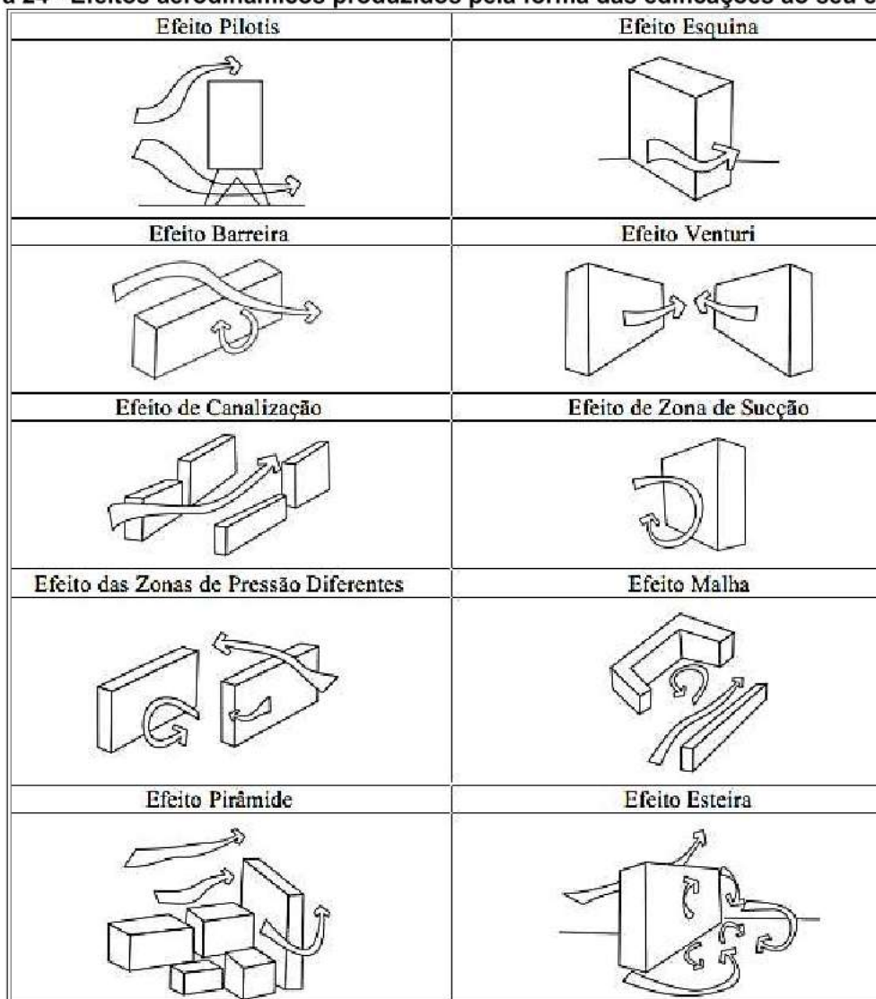
Figura 24 - Efeitos aerodinâmicos produzidos pela forma das edificações ao seu entorno
