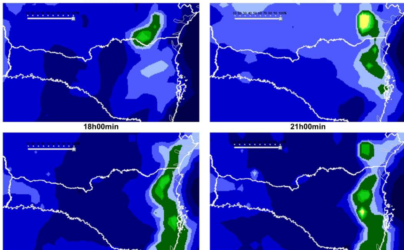
Figura 21 - Concentração de compostos orgânicos voláteis 06h00min 12h00min
