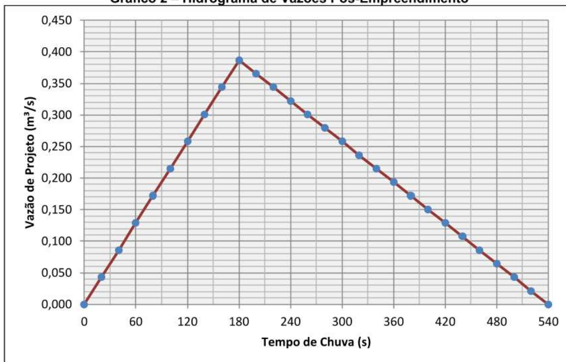
Gráfico 2 – Hidrograma de Vazões Pós-Emprego
