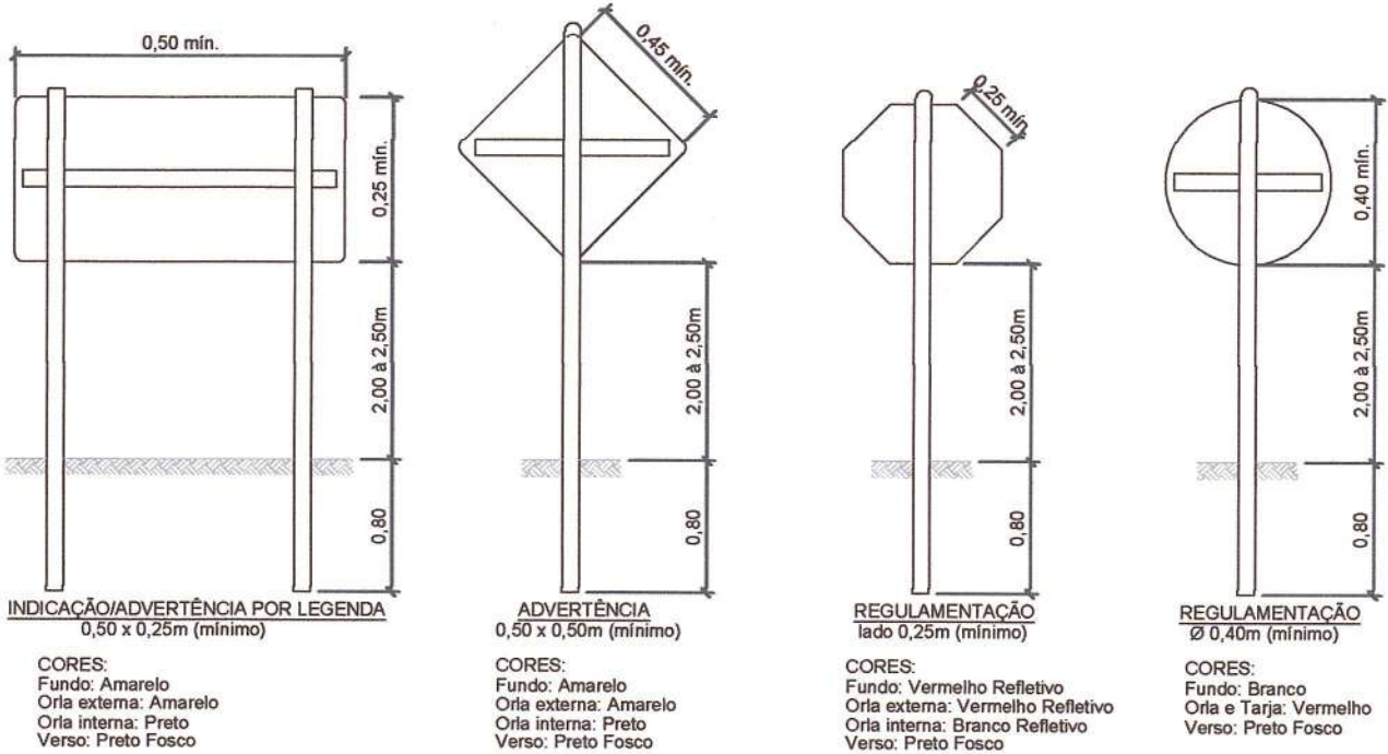
3 DETALHE PLACAS DE SINALIZAÇÃO SEM ESCALA
