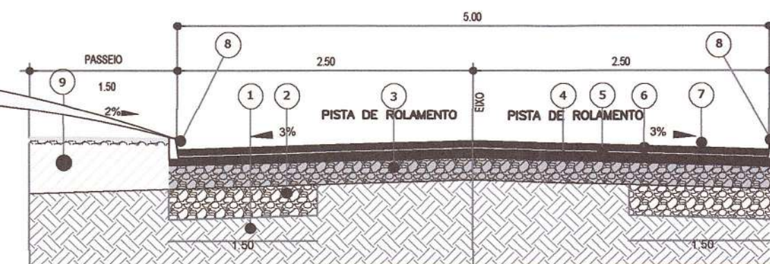
1 SEÇÃO A (VIA 5 METROS) ESCALA: Sem Escala
