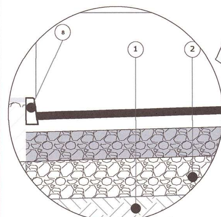
2 DETALHE SARJETA ESCALA: Sem Escala
