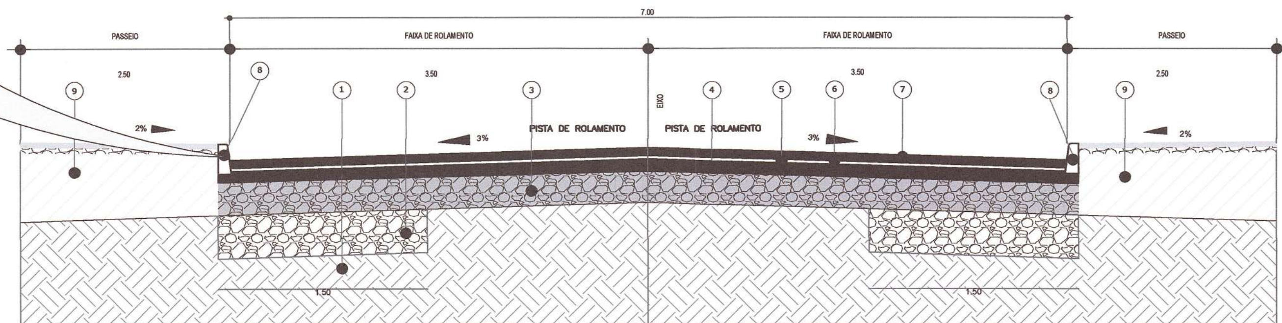
3 SEÇÃO B (VIA 7 METROS) ESCALA: Sem Escala
