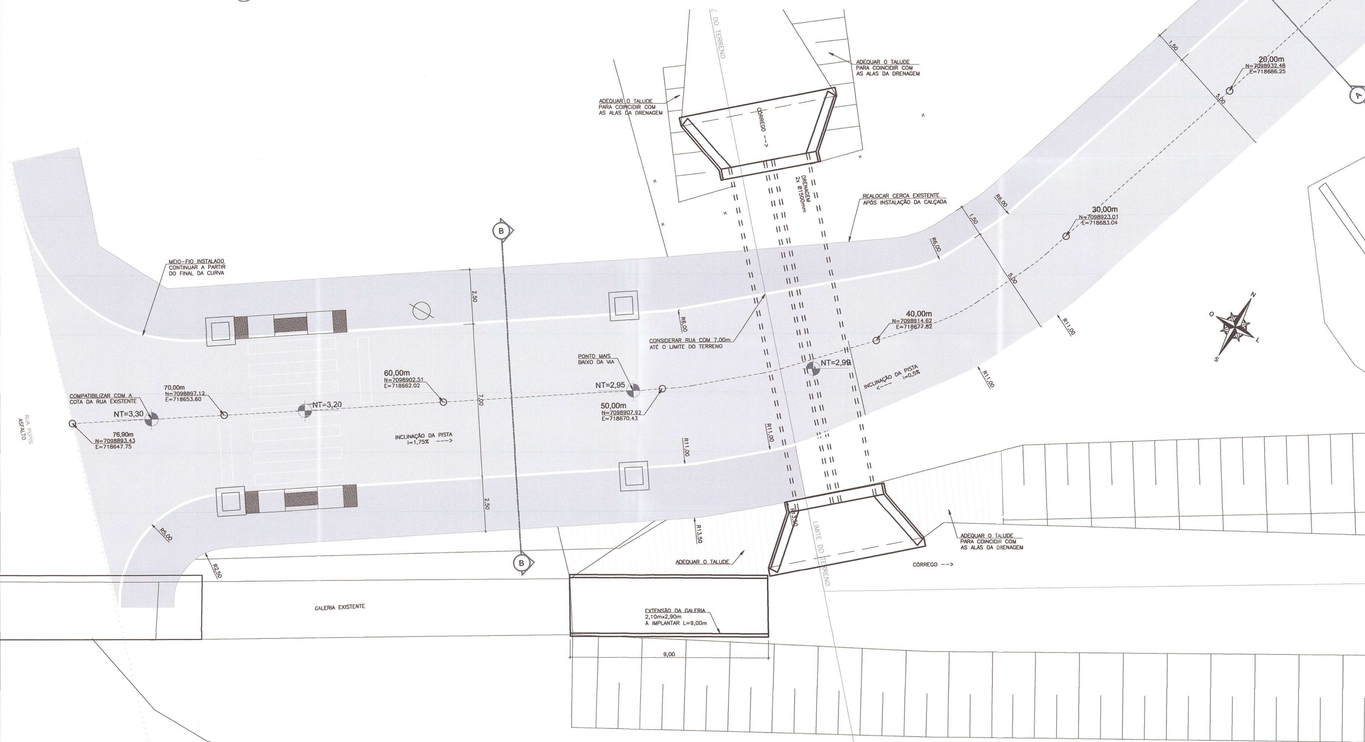
4 PLANTA ESCALA: 1:200
