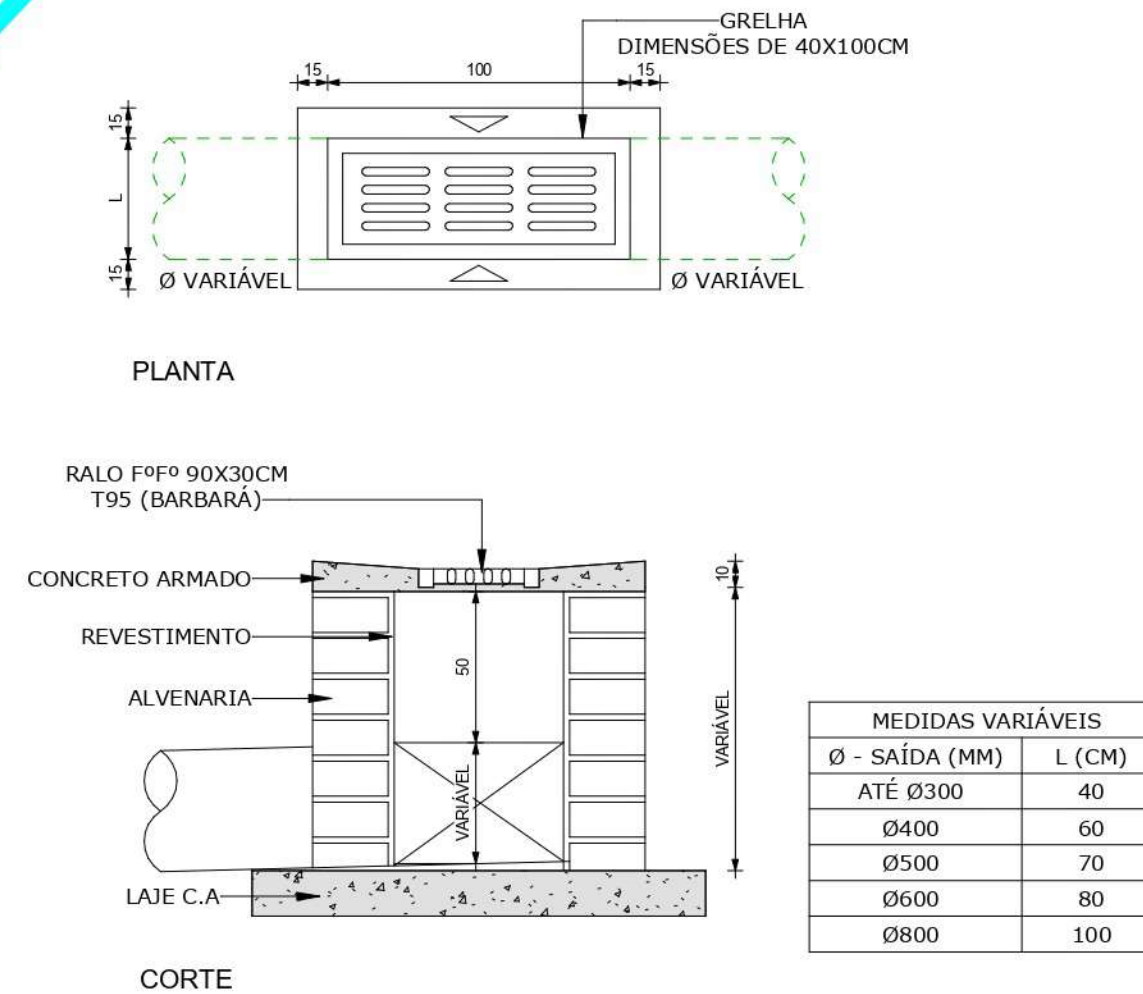
DETALHE BOCA DE LOBO SEM ESCALA BOCA DE LEÃO ÁGUA PLUVIAL COM GRELHA ESC 1 : 25
