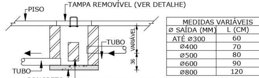
DETALHE CAIXA DE PASSAGEM COM TAMPA DA RAMPA SEM ESCALA
