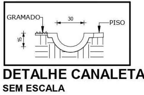
DETALHE CANALETA SEM ESCALA
