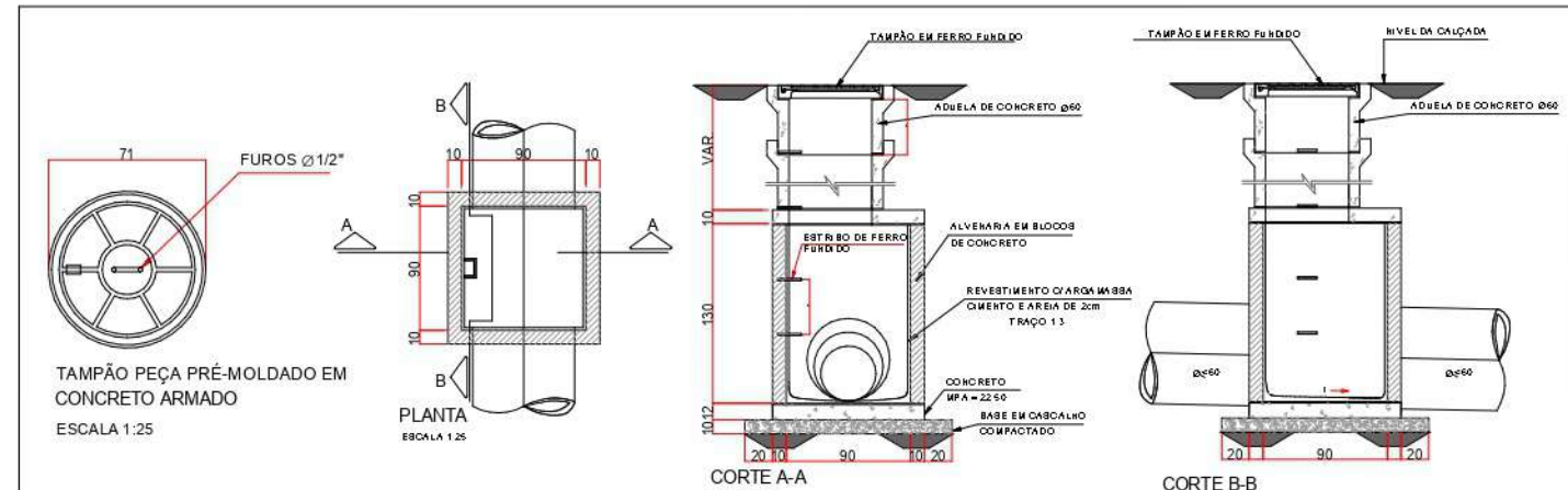
DETALHE POÇO DE VISITA ESC 1 : 15
