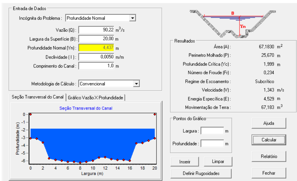
Figura 21 – Programa Canal, com os dados de vazão para 200 anos de tempo de retorno. Fonte: ONE.
