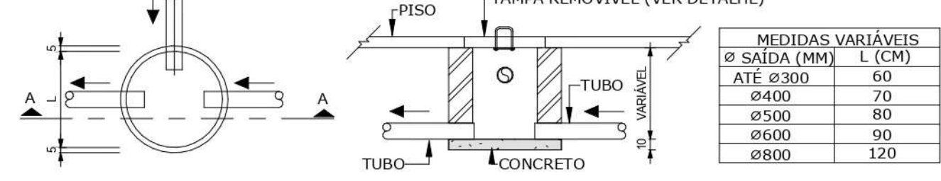
DETALHE CAIXA DE PASSAGEM COM TAMPA SEM ESCALA
