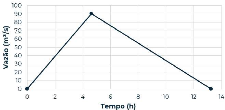
Figura 18 – Hidrograma de Projeto para TR = 200 anos. Fonte: ONE.
