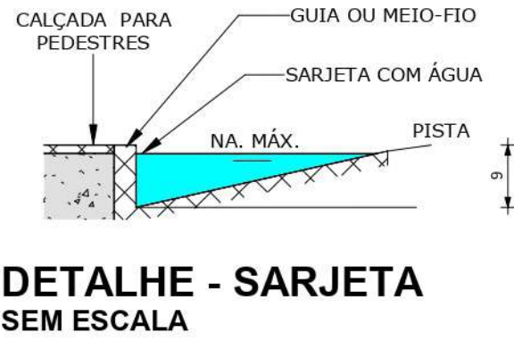
DETALHE - SARJETA SEM ESCALA
