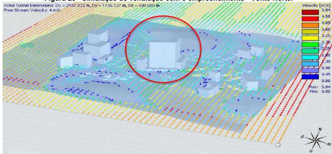
Figura 28 - Simulação de ventilação com o empreendimento - Vento Norte:
