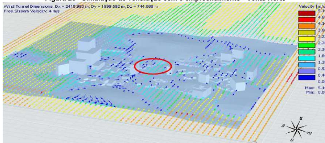
Figura 26 - Simulação de ventilação sem o empreendimento - Vento Norte
