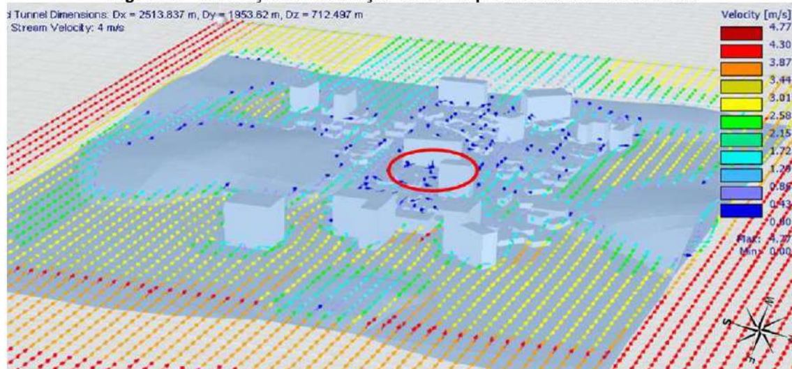
Figura 25 - Simulação de ventilação sem o empreendimento - Vento Leste
