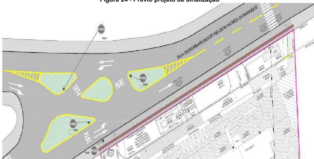
Figura 24 - Prévio projeto de sinalização
