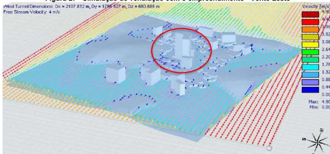
Figura 27 - Simulação de ventilação com o empreendimento - Vento Leste
