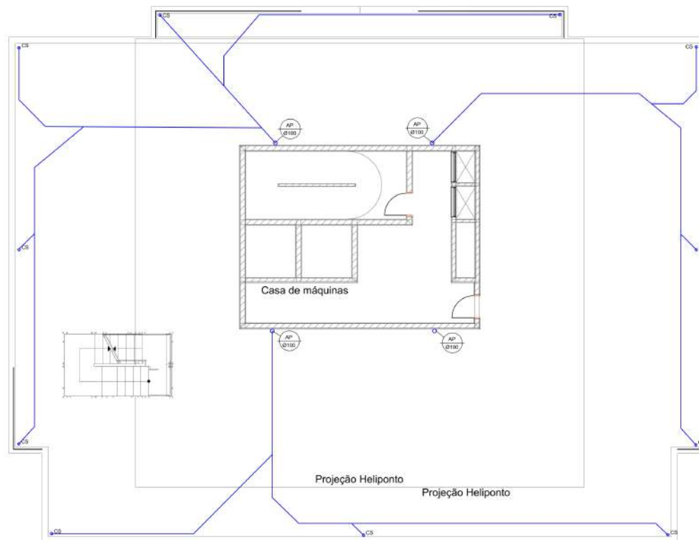
PLANTA DE CAPTAÇÃO DE ÁGUAS PLUVIAIS - COBERTURA ESCALA 1:75
