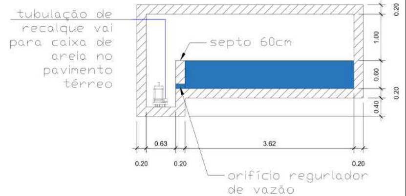
DETALHE - BACIA DE CONTENÇÃO CORTE TRANSVERSAL ESCALA 1:25
