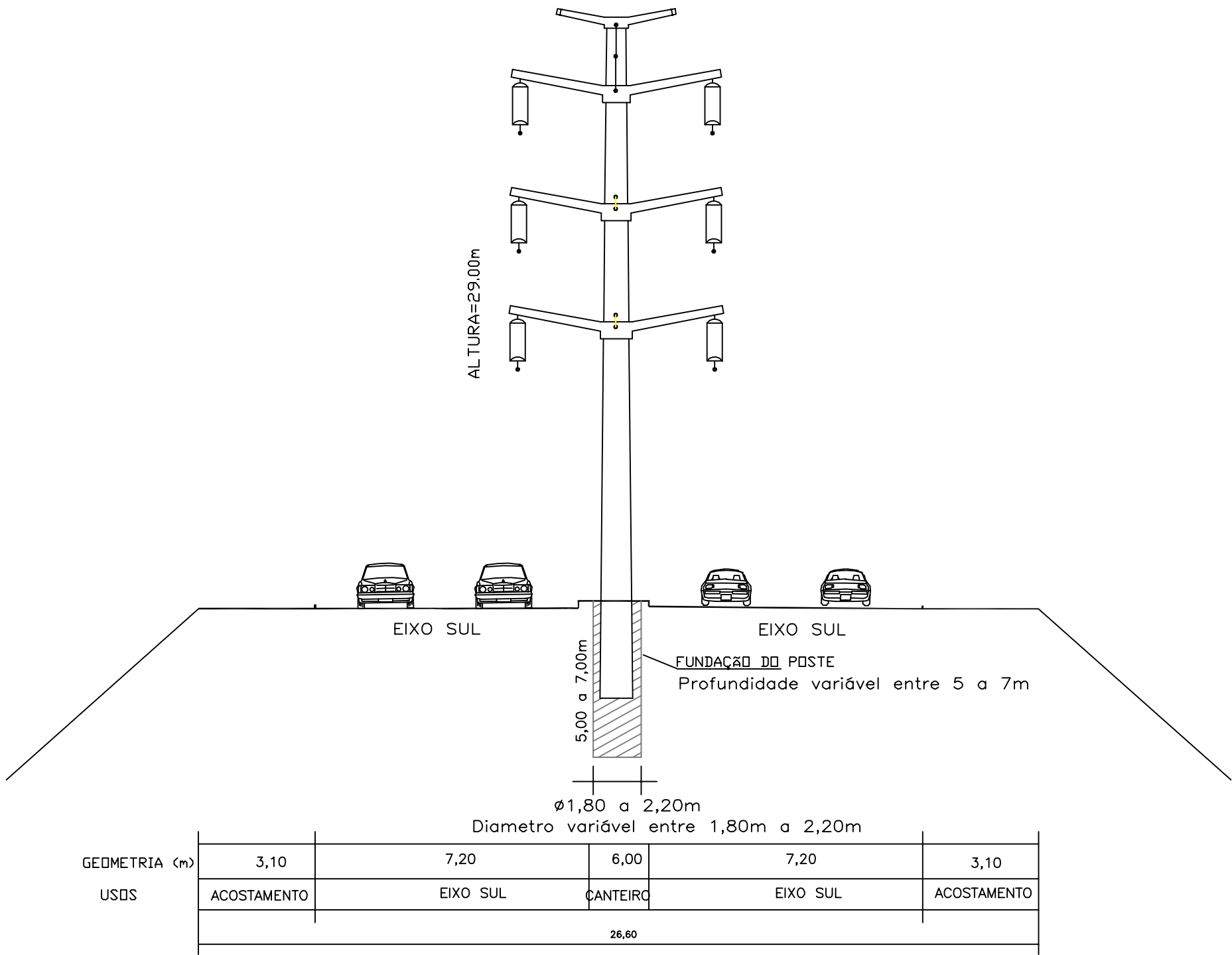
DETALHE EST.17 a 20
