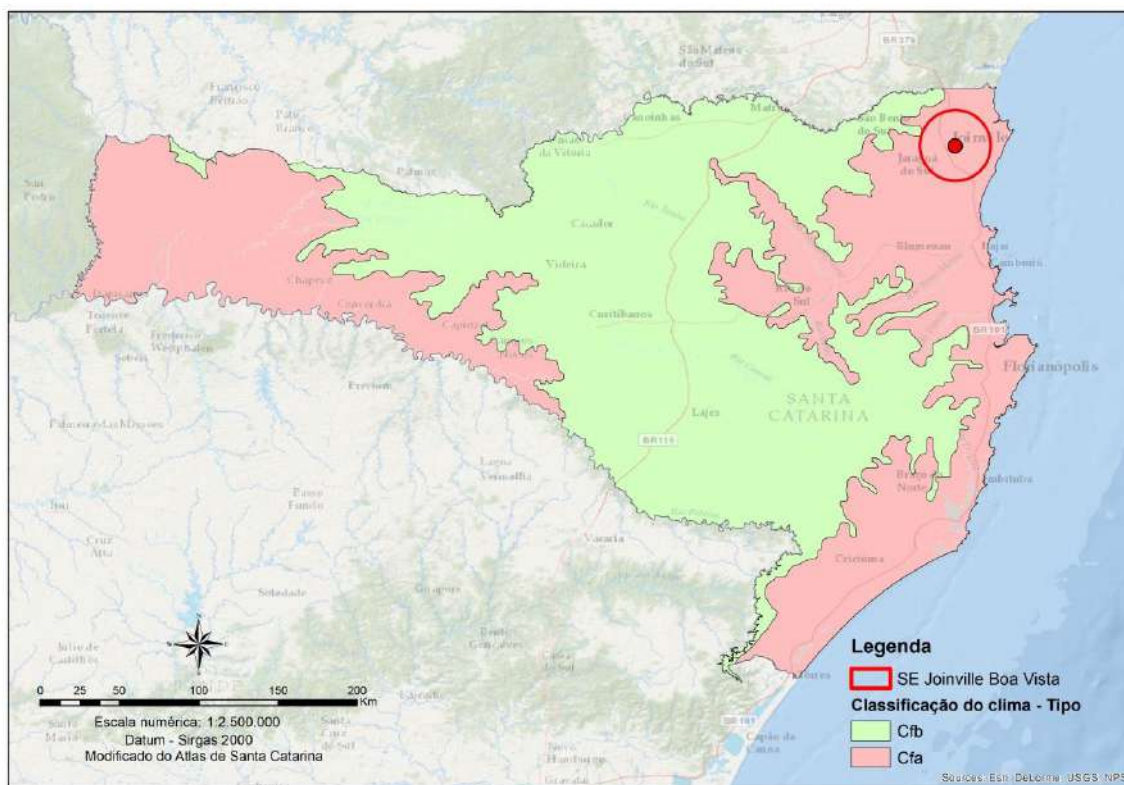
Figura 28: Classificação Climática segundo Köppen para o estado de Santa Catarina com destaque em vermelho para a localização do empreendimento. Fonte: Adaptado do Atlas Climatológico de Santa Catarina (PANDOLFO, 2002).
