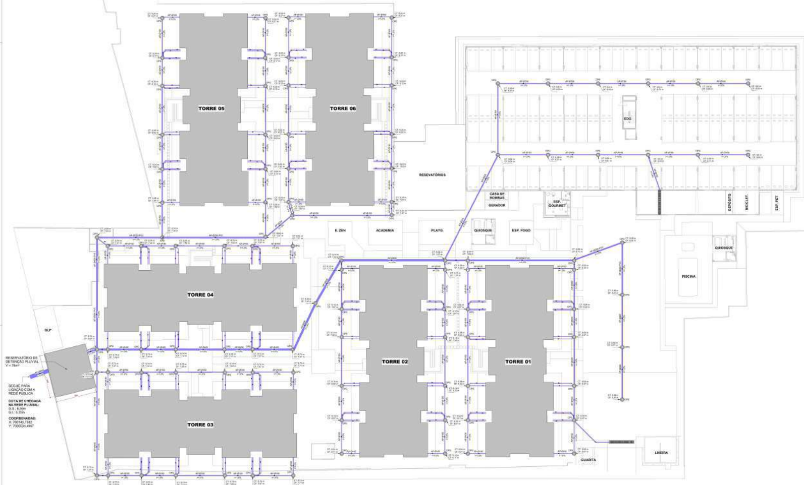
PLANTA BAIXA IMPLANTAÇÃO - DRENAGEM Escala 1:100
