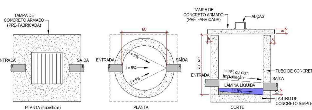
DETALHE - CAIXA DE INSPEÇÃO PLUVIAL COM GRELHA (CIPG) Sem escala
