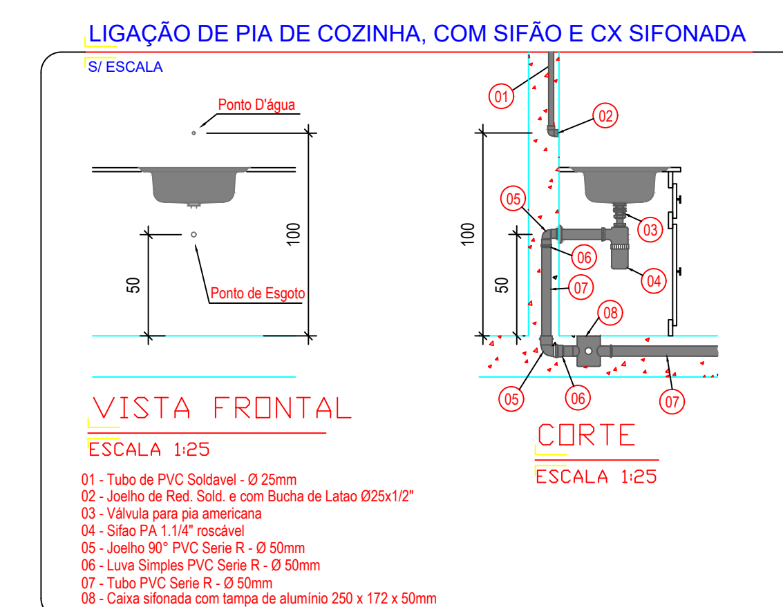
LIGAÇÃO DE PIA DE COZINHA, COM SIFÃO E CX SIFONADA
