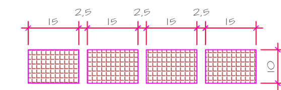
Corte D-D
