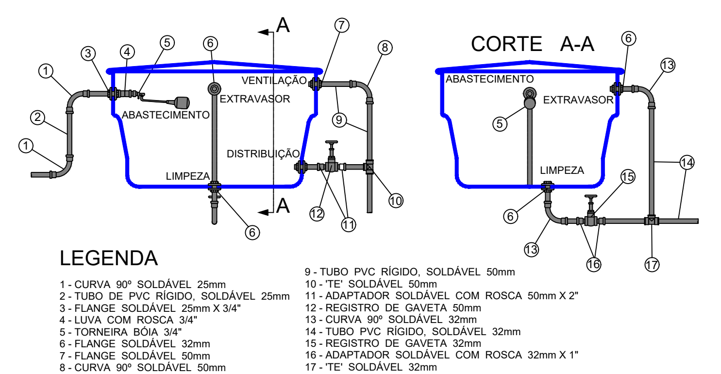
DETALHE CAIXA D'ÁGUA
