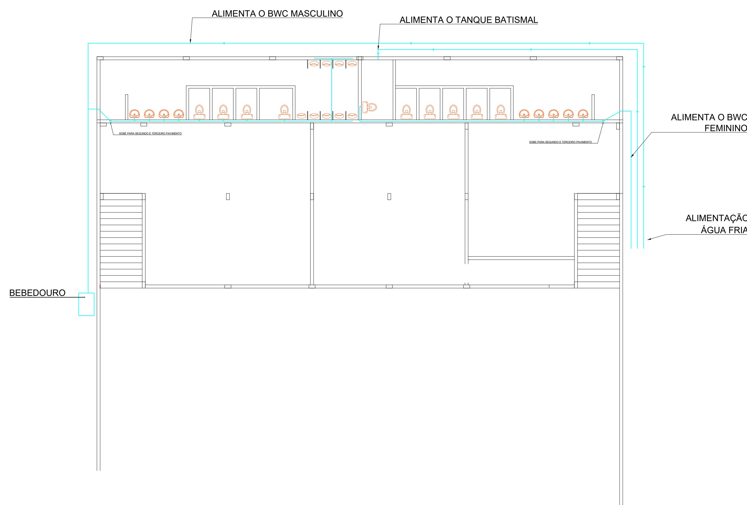
DETALHE 01 - ÁGUA FRIA
