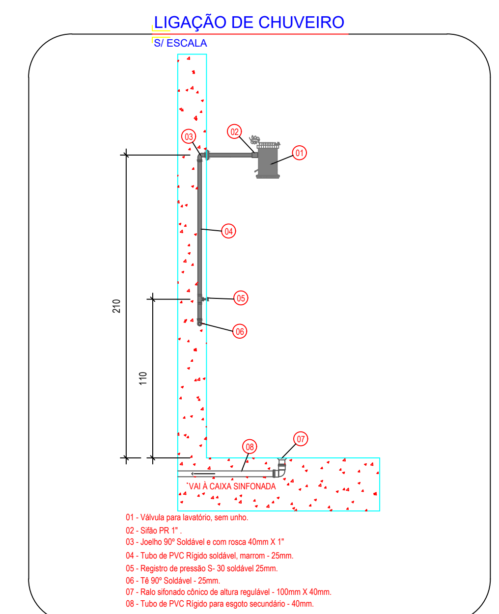
LIGAÇÃO DE CHUIVEIRO
