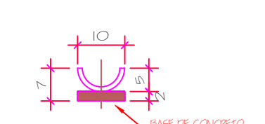
Perfil da Calha Vertedoura
