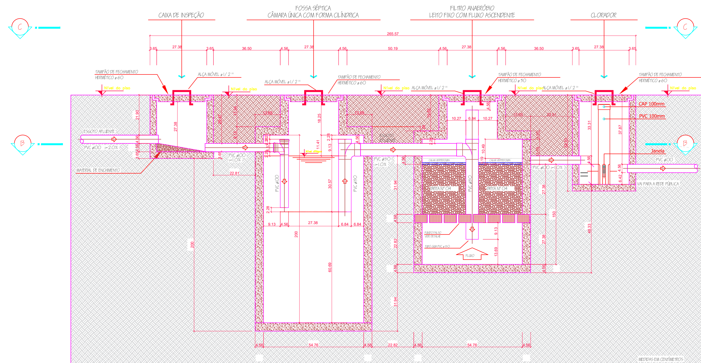
Corte A-A
