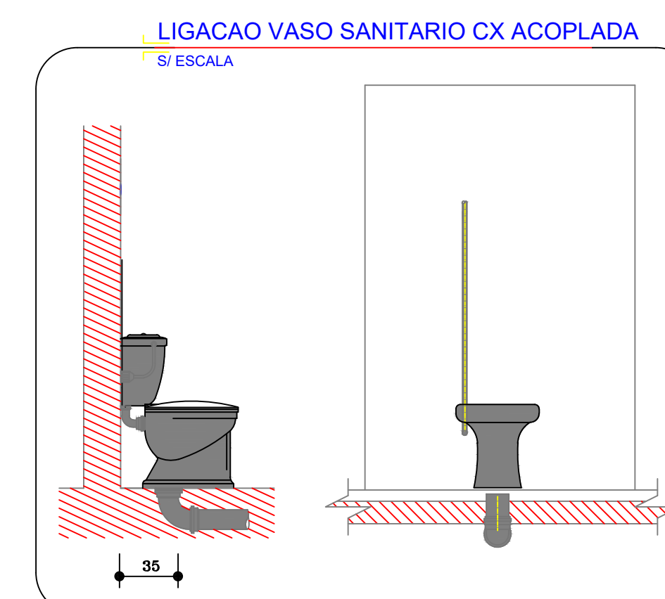
LIGAÇÃO VASO SANITÁRIO CX ACOPLADA
