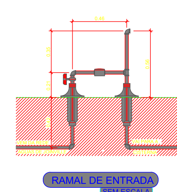
RAMAL DE ENTRADA
