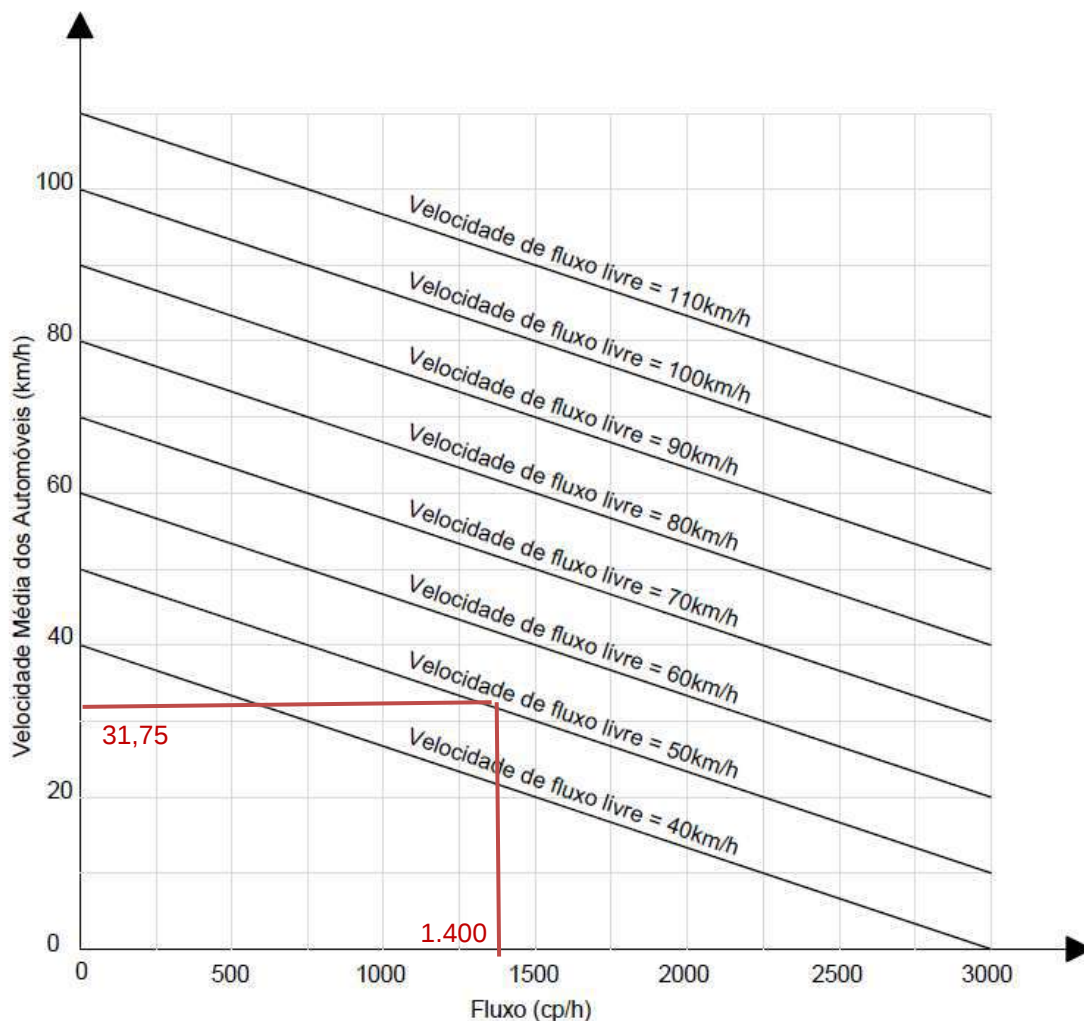
Gráfico 7 - Capacidade de Fluxo Avenida Marquês de Olinda
