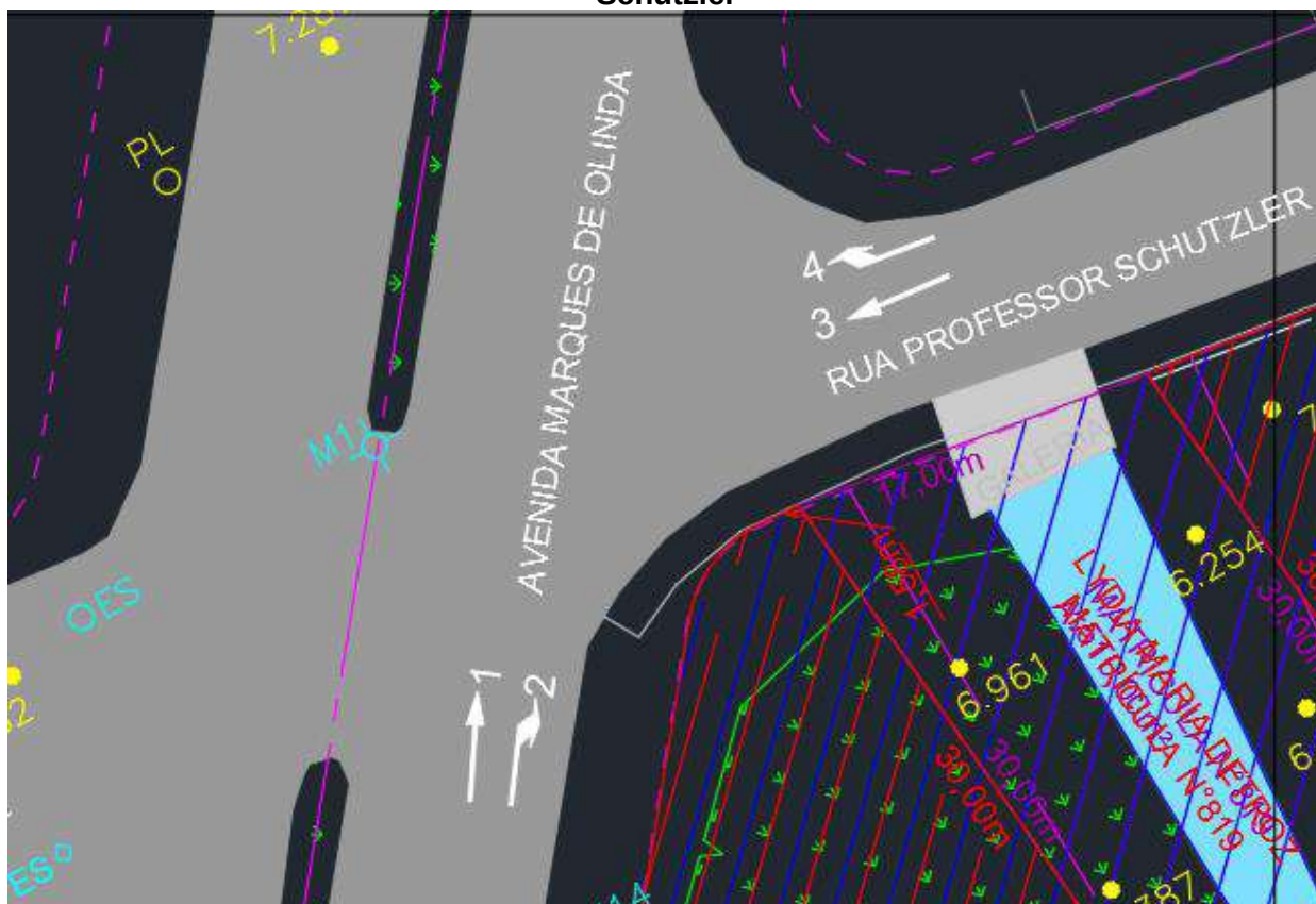
Figura 48 – Esquema de fluxos aferidos – Avenida Marquês de Olinda com Professor Schutzler
