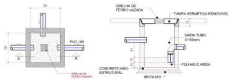
PLANTA BAIXA
