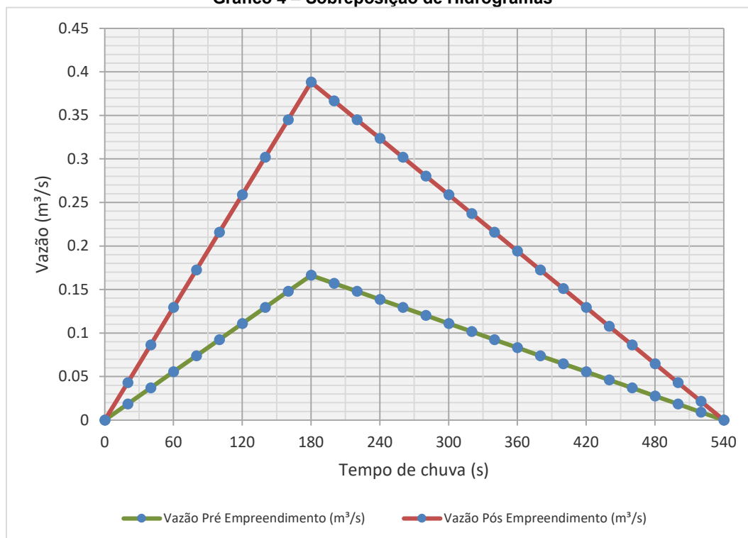
Gráfico 4 – Sobreposição de Hidrogramas
