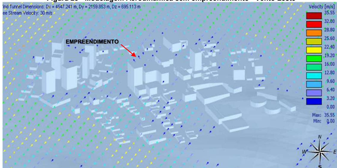
Figura 25 - Modelagem Aerodinâmica sem empreendimento - Vento Leste
