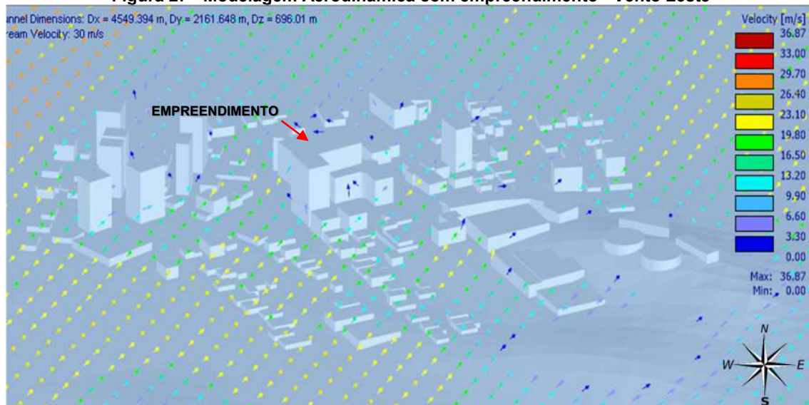
Figura 27 - Modelagem Aerodinâmica com empreendimento - Vento Leste
