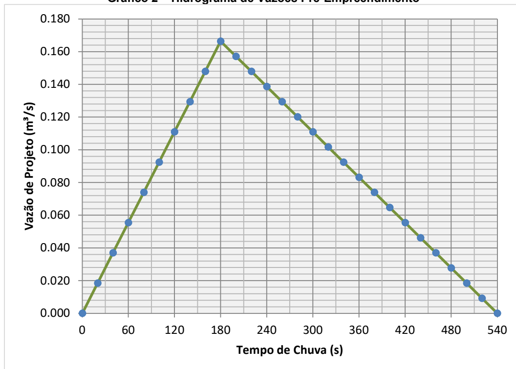
Gráfico 2 – Hidrograma de Vazões Pré-Empreendimento
