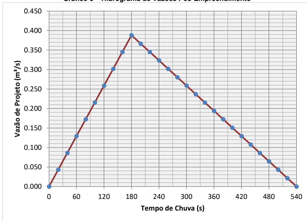
Gráfico 3 – Hidrograma de Vazões Pós-Empreendimento
