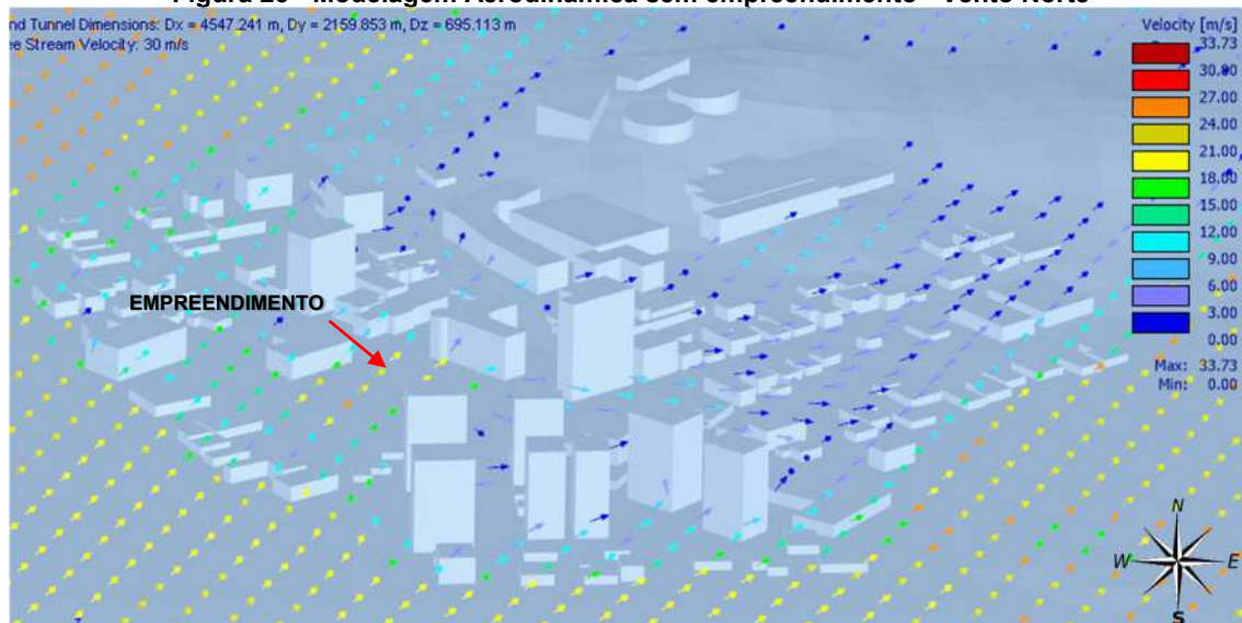
Figura 26 - Modelagem Aerodinâmica sem empreendimento - Vento Norte
