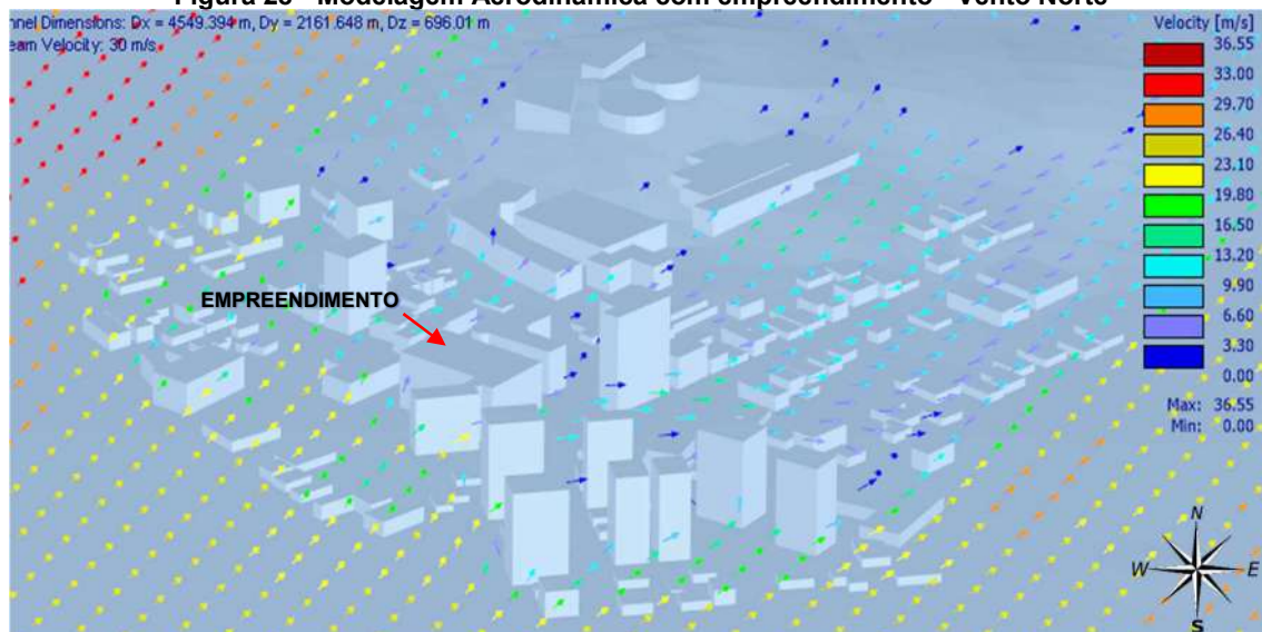
Figura 28 - Modelagem Aerodinâmica com empreendimento - Vento Norte
