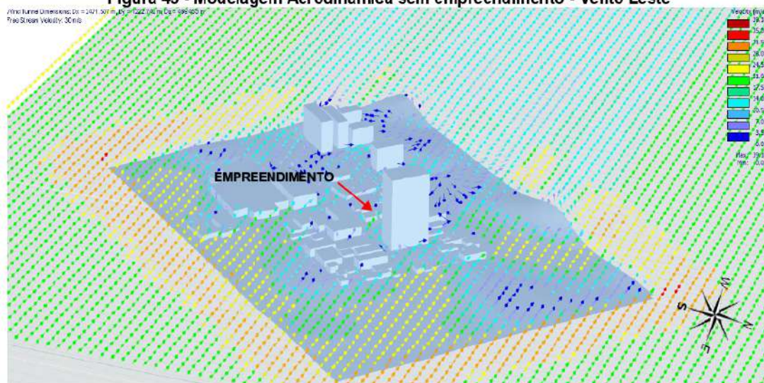
Figura 45 - Modelagem Aerodinâmica sem empreendimento - Vento Leste
