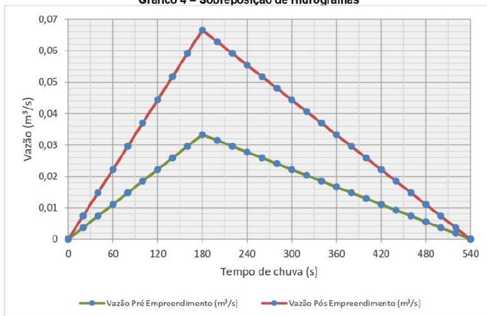
Gráfico 4 – Sobreposição de Hidrogramas
