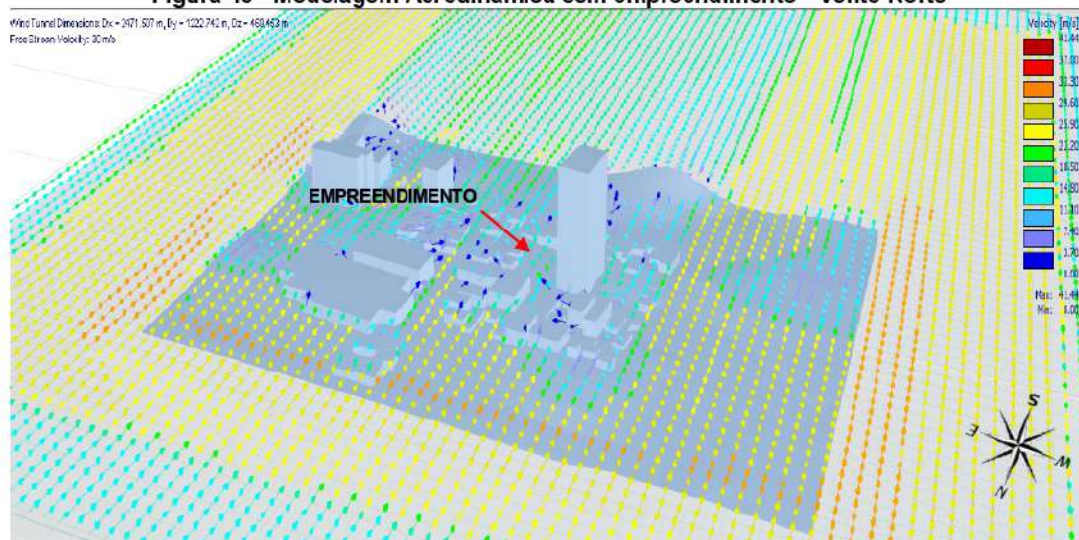
Figura 46 - Modelagem Aerodinâmica sem empreendimento - Vento Norte
