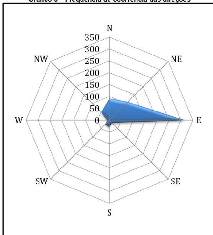
Gráfico 6 – Frequência de ocorrência das direções
