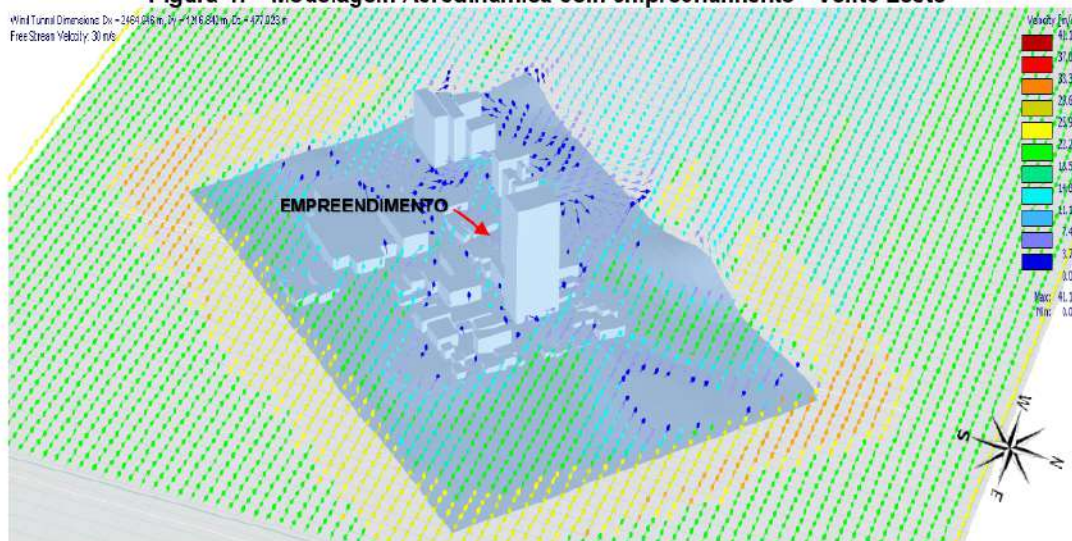
Figura 47 - Modelagem Aerodinâmica com empreendimento - Vento Leste
