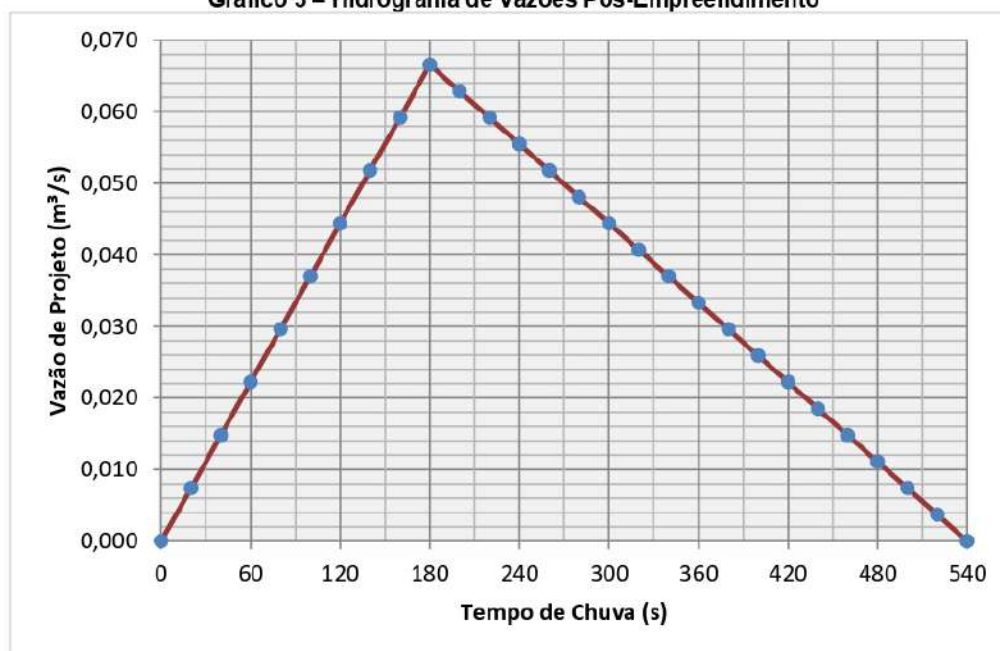
Gráfico 3 – Hidrograma de Vazões Pós-Empreendimento
