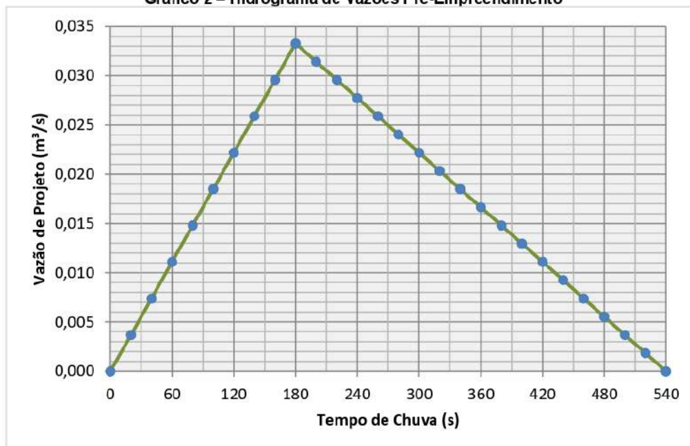
Gráfico 2 – Hidrograma de Vazões Pré-Engrego
