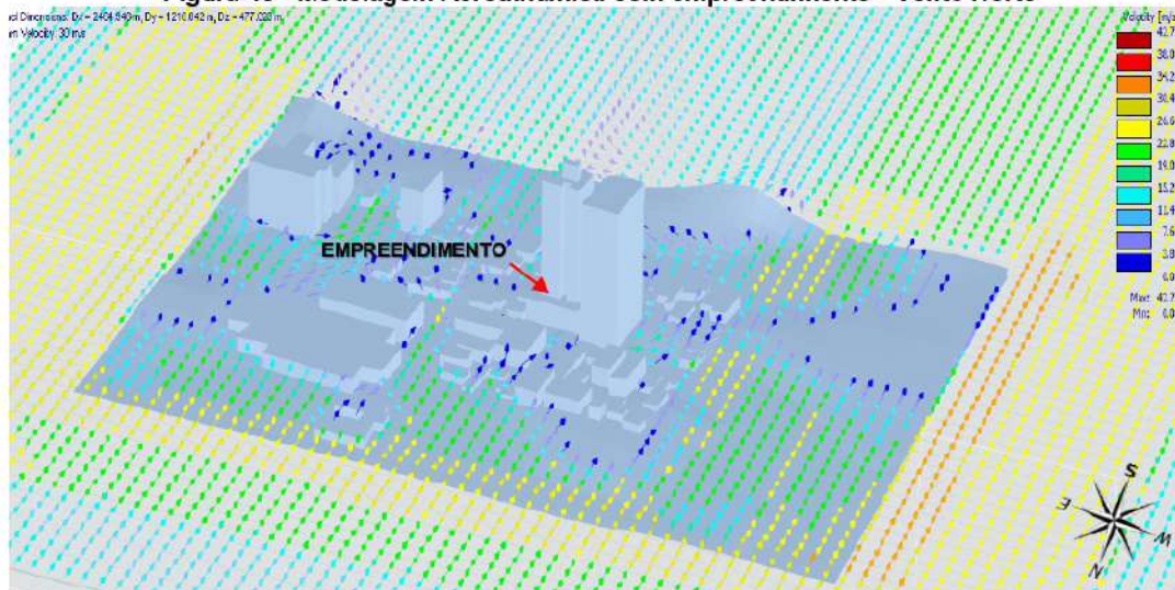
Figura 48 - Modelagem Aerodinâmica com empreendimento - Vento Norte
