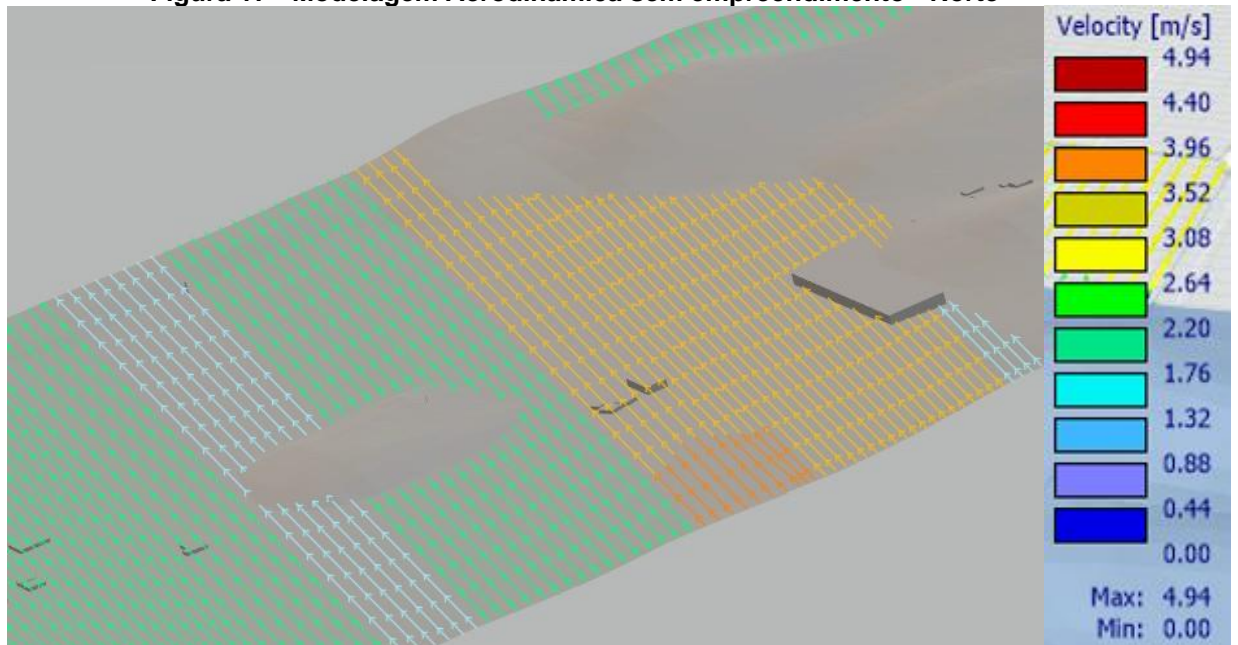
Figura 17 - Modelagem Aerodinâmica sem empreendimento - Norte
