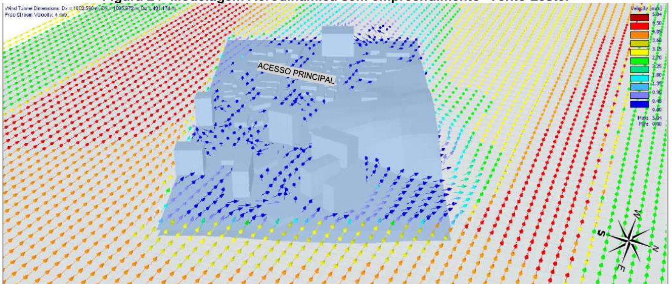
Figura 24- Modelagem Aerodinâmica sem empreendimento- Vento Leste.
