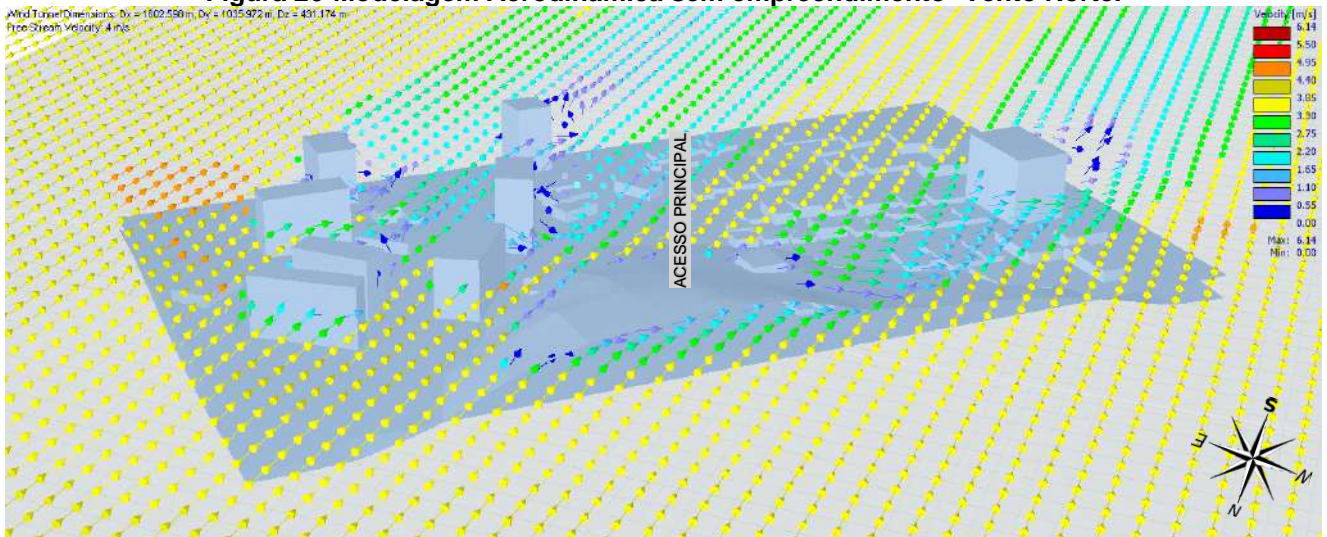
Figura 26-Modelagem Aerodinâmica sem empreendimento- Vento Norte.
