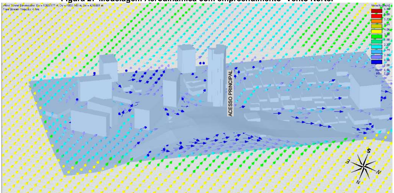
Figura 27-Modelagem Aerodinâmica com empreendimento- Vento Norte.
