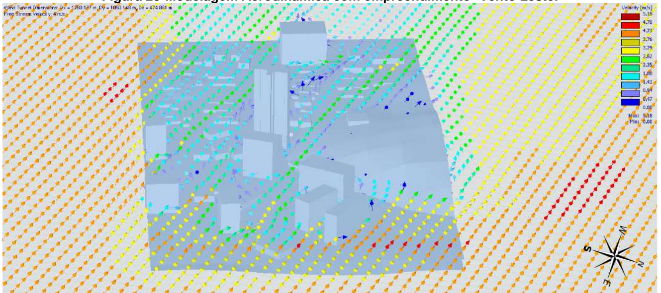
Figura 25-Modelagem Aerodinâmica com empreendimento- Vento Leste.
