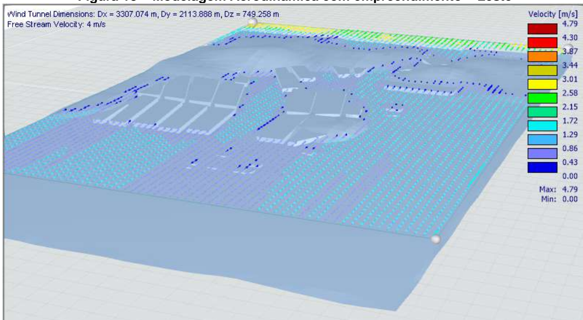
Figura 18 – Modelagem Aerodinâmica com empreendimento – Leste
