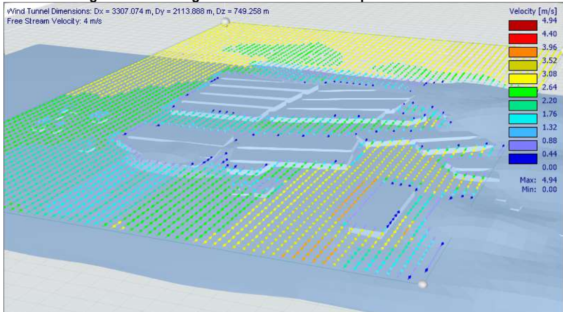
Figura 17 - Modelagem Aerodinâmica com empreendimento - Norte
