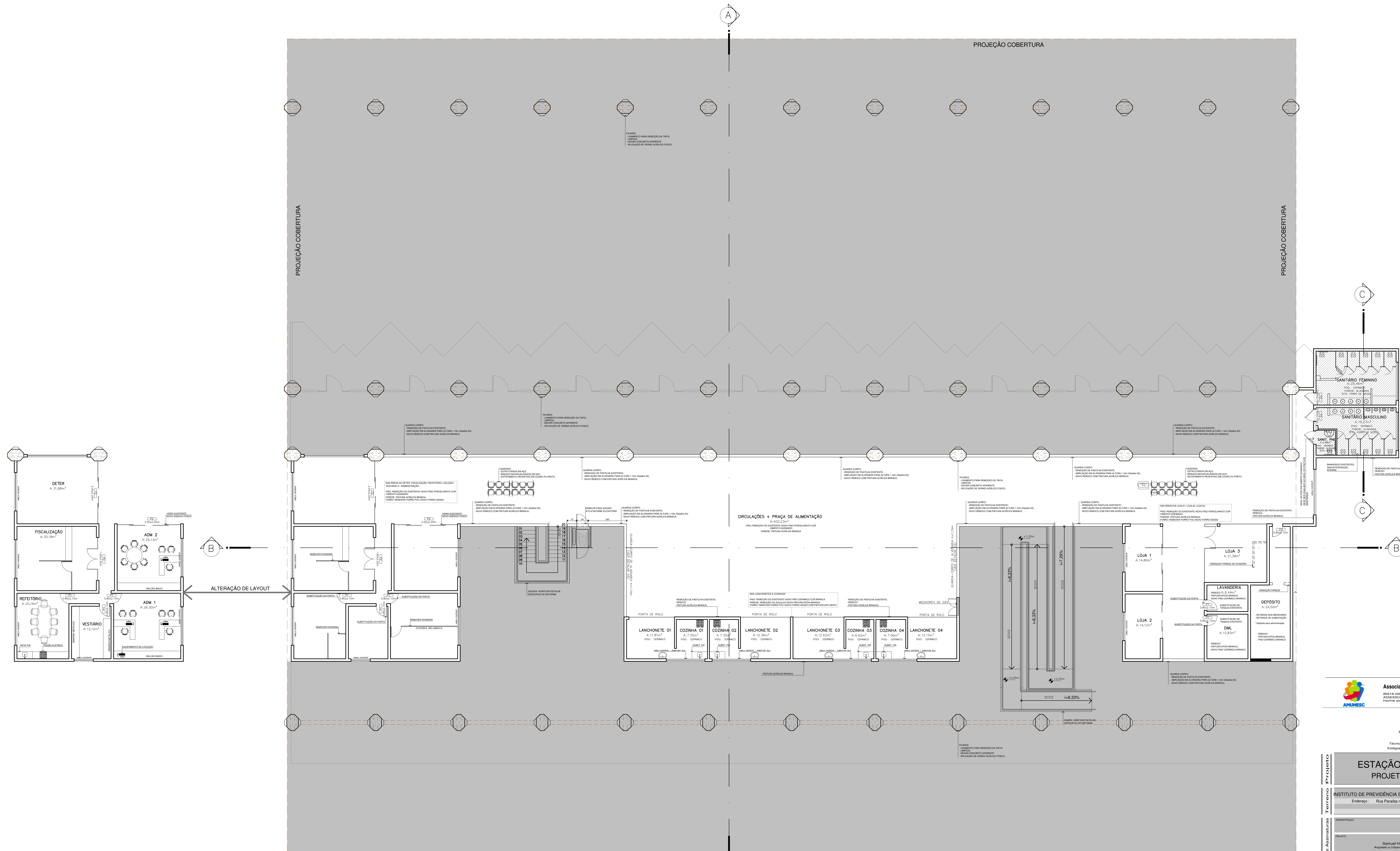
PLANTA BAIXA PAVIMENTO SUPERIOR Escala 1/100
