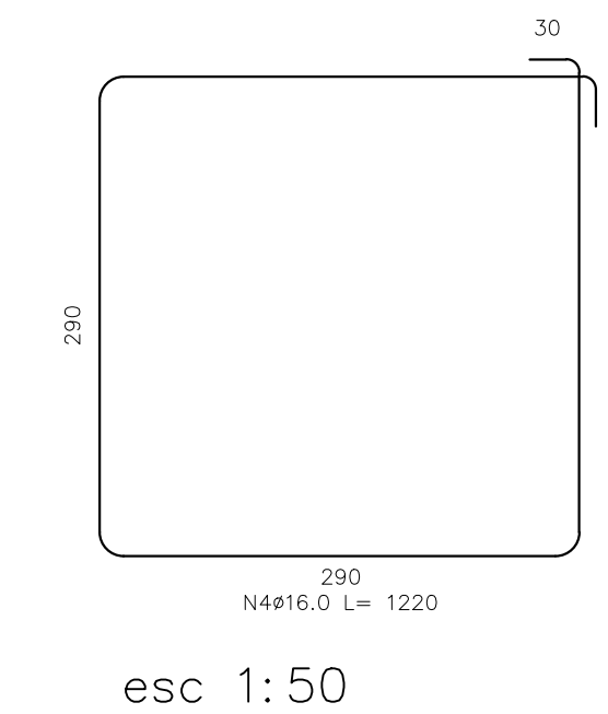
esc 1:50
