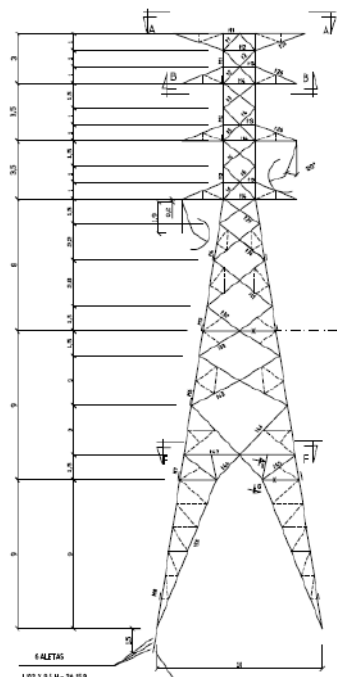
Figura 5: Estrutura Metálica do tipo EAMD.
