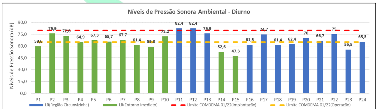
Figura 44: Síntese dos resultados obtidos na campanha de monitoramento dos níveis de pressão sonora ambiental.
