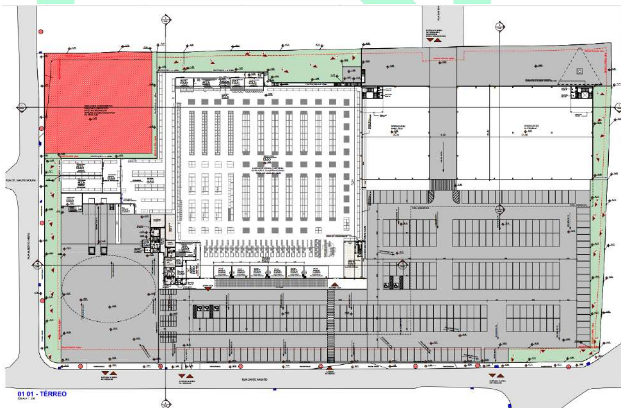
Figura 6: Layout de implantação do empreendimento.
