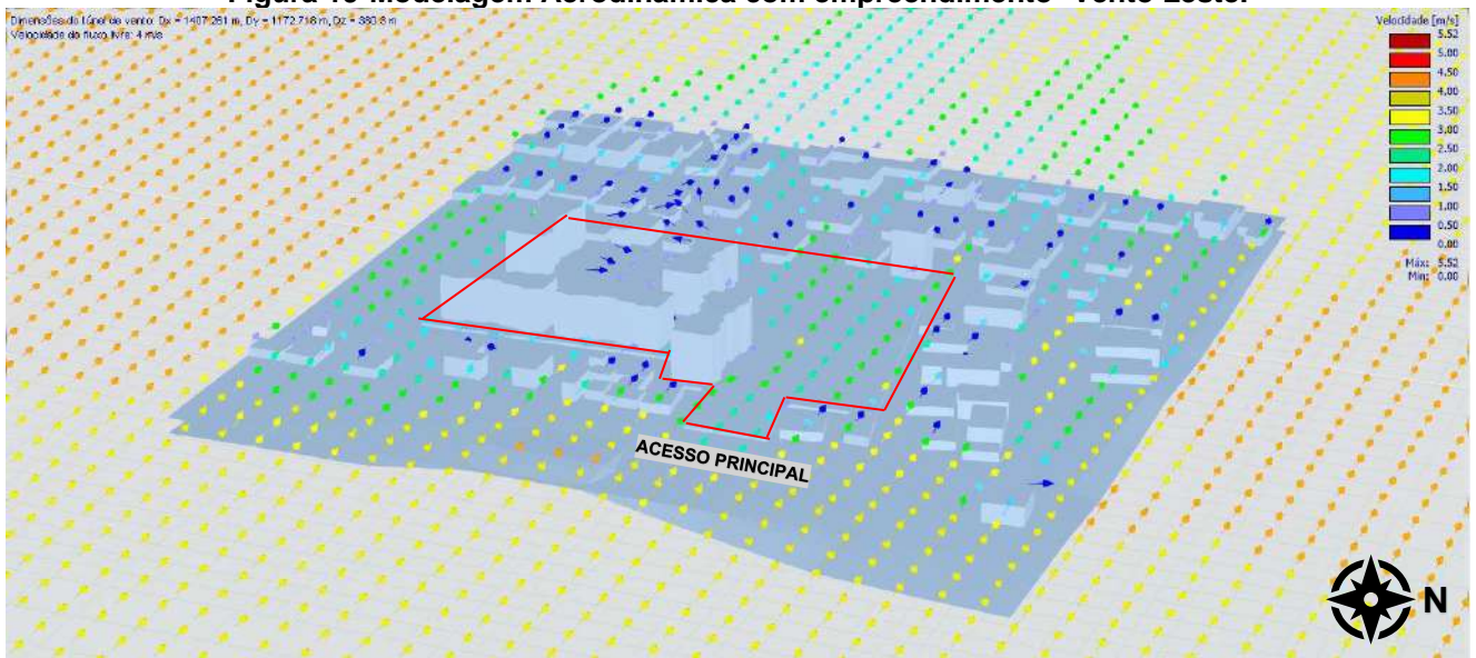
Figura 19- Modelagem Aerodinâmica com empreendimento- Vento Leste.
