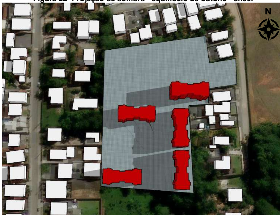
Figura 22- Projeção de sombra - equinócio de outono - 8h00.
