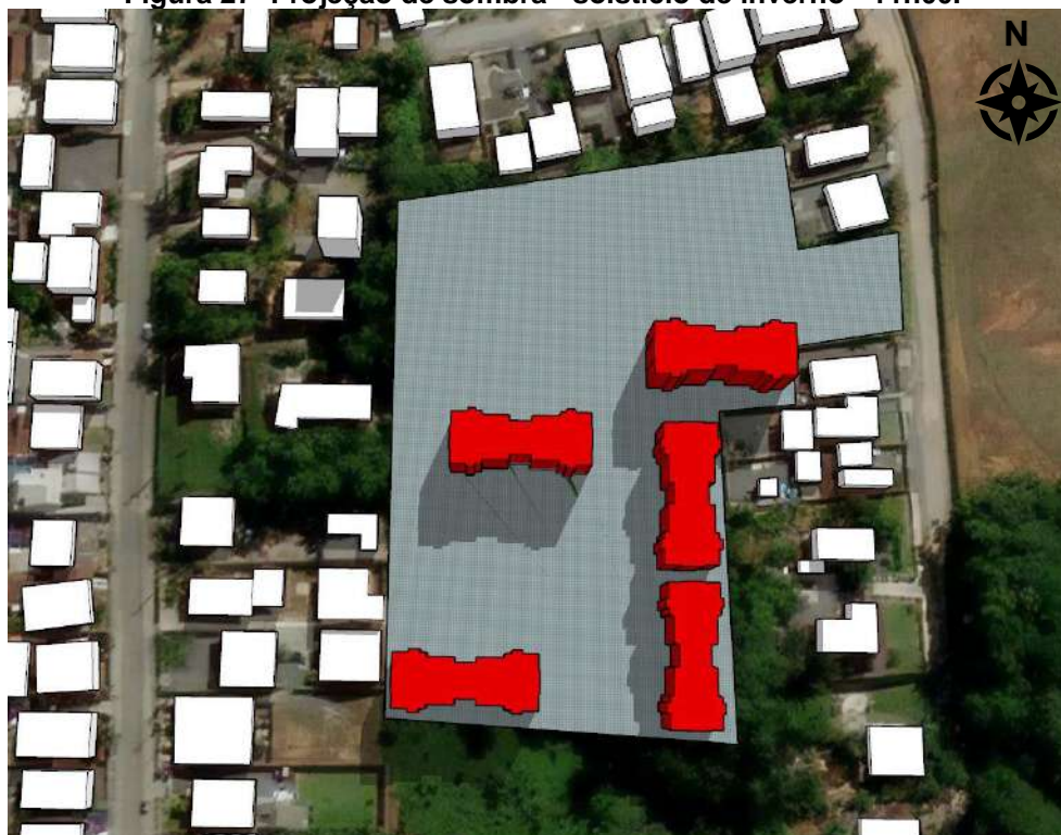
Figura 27- Projeção de sombra - solstício de inverno - 11h00.
