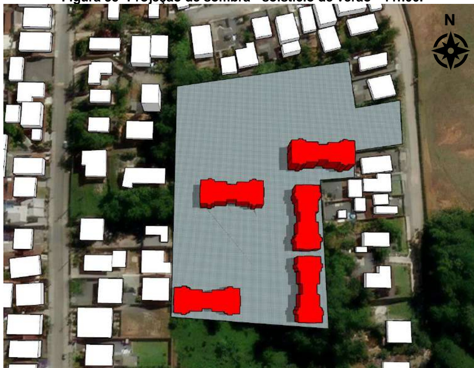
Figura 35- Projeção de sombra - solstício de verão - 11h00.
