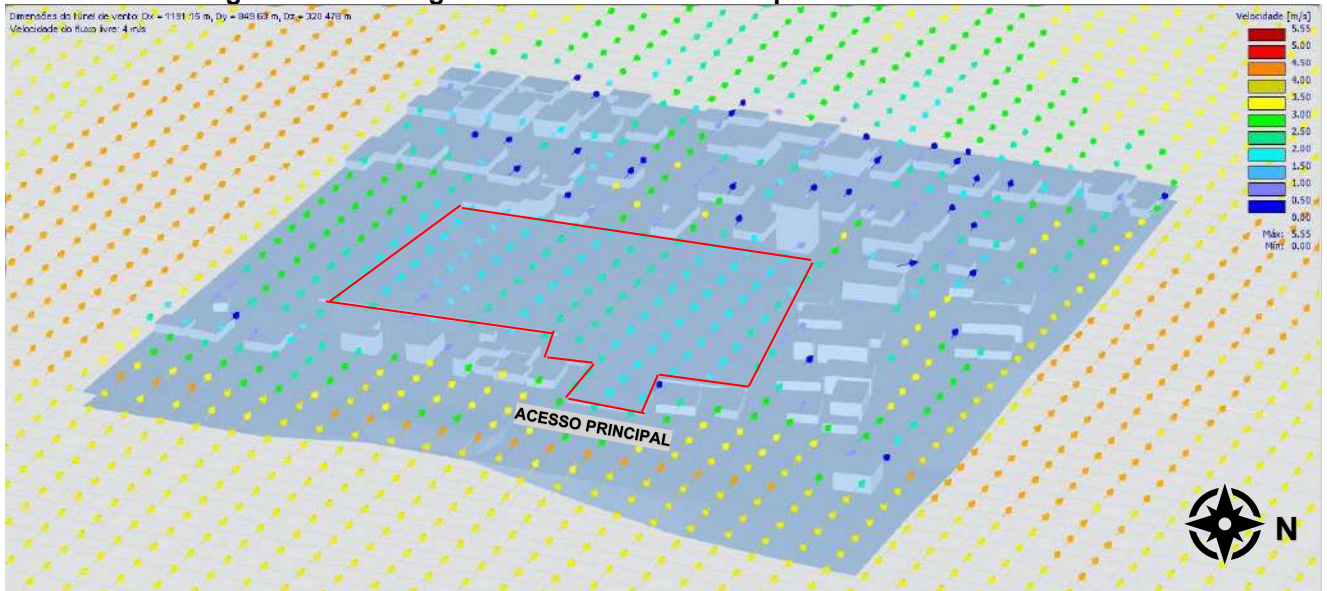
Figura 18- Modelagem Aerodinâmica sem empreendimento- Vento Leste.
