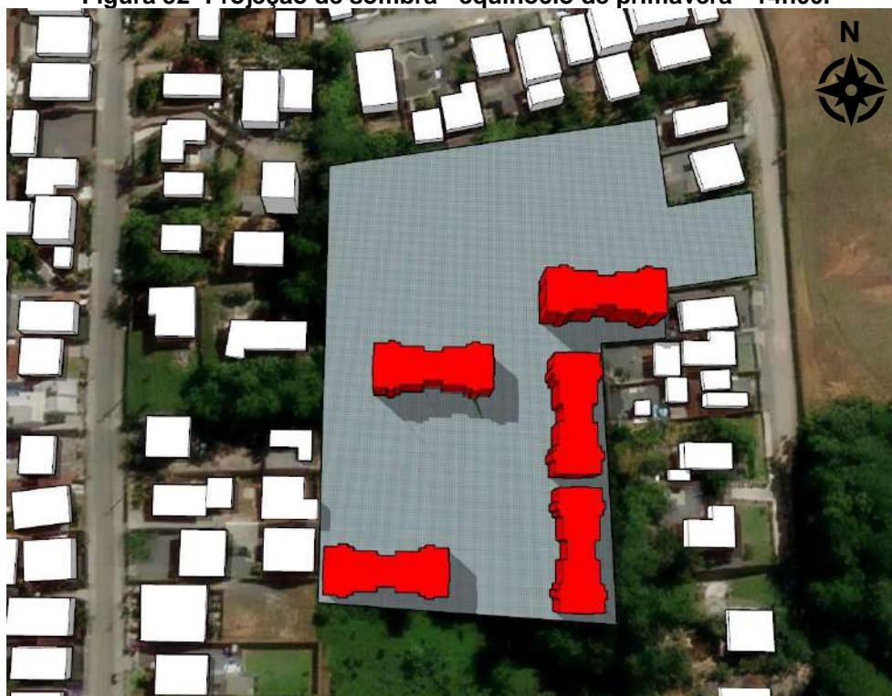
Figura 32- Projeção de sombra - equinócio de primavera - 14h00.
