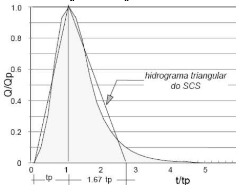
Figura 45- Hidrograma do SCS
