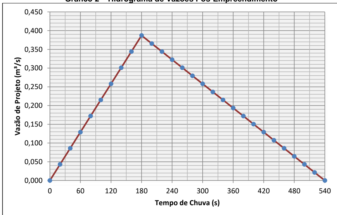
Gráfico 2 – Hidrograma de Vazões Pós-Empredimento
