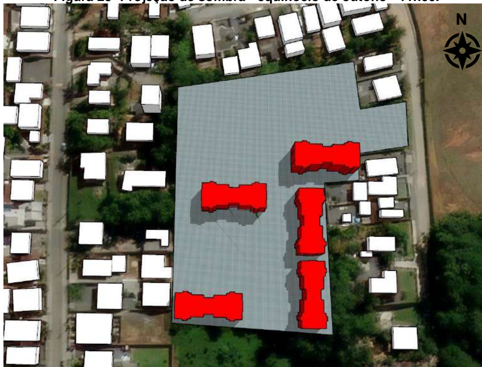
Figura 23- Projeção de sombra - equinócio de outono - 11h00.
