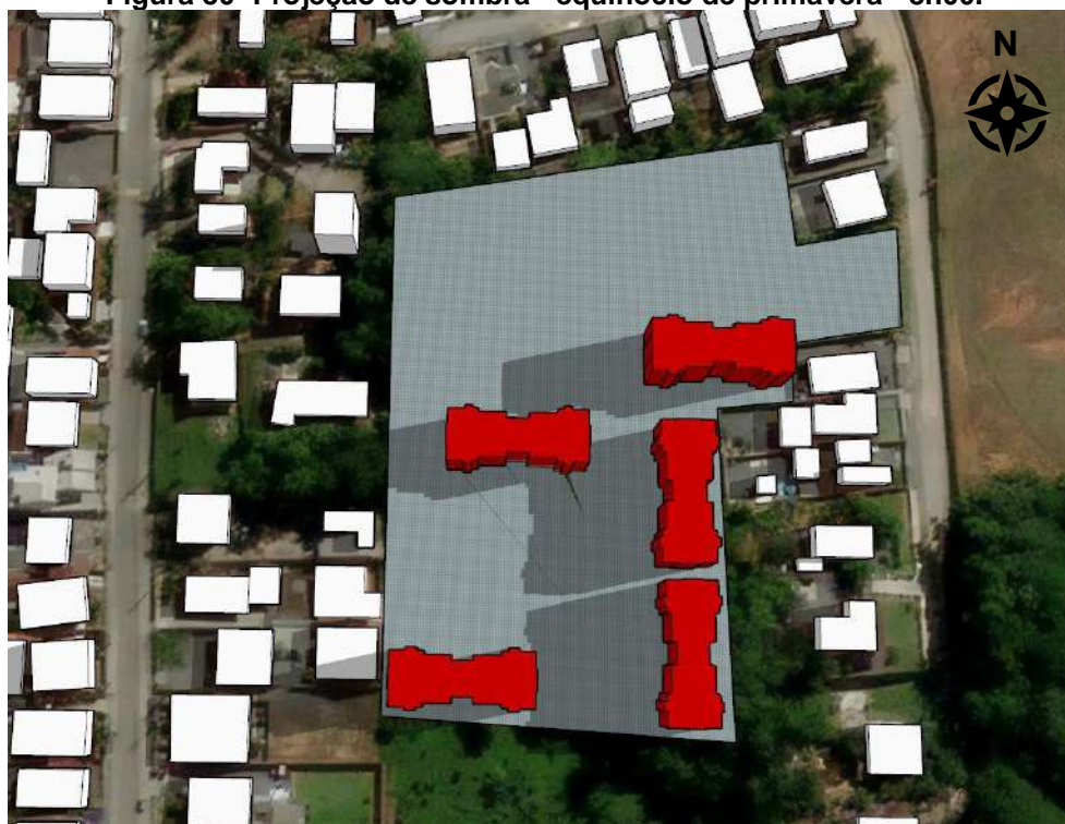
Figura 30- Projeção de sombra - equinócio de primavera - 8h00.
