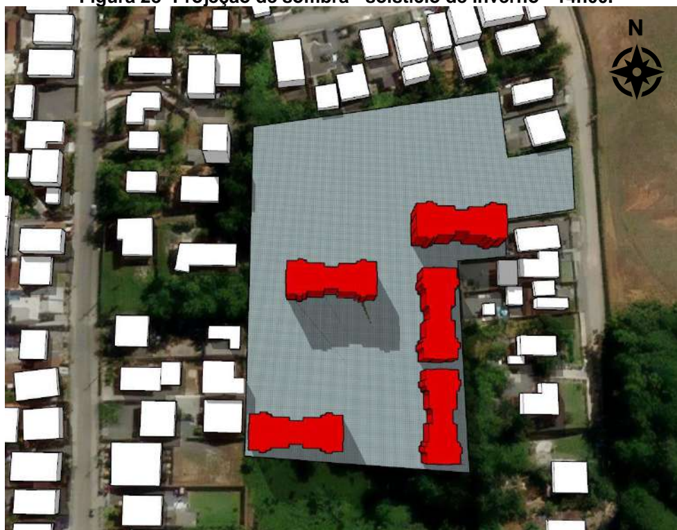
Figura 28- Projeção de sombra - solstício de inverno - 14h00.
