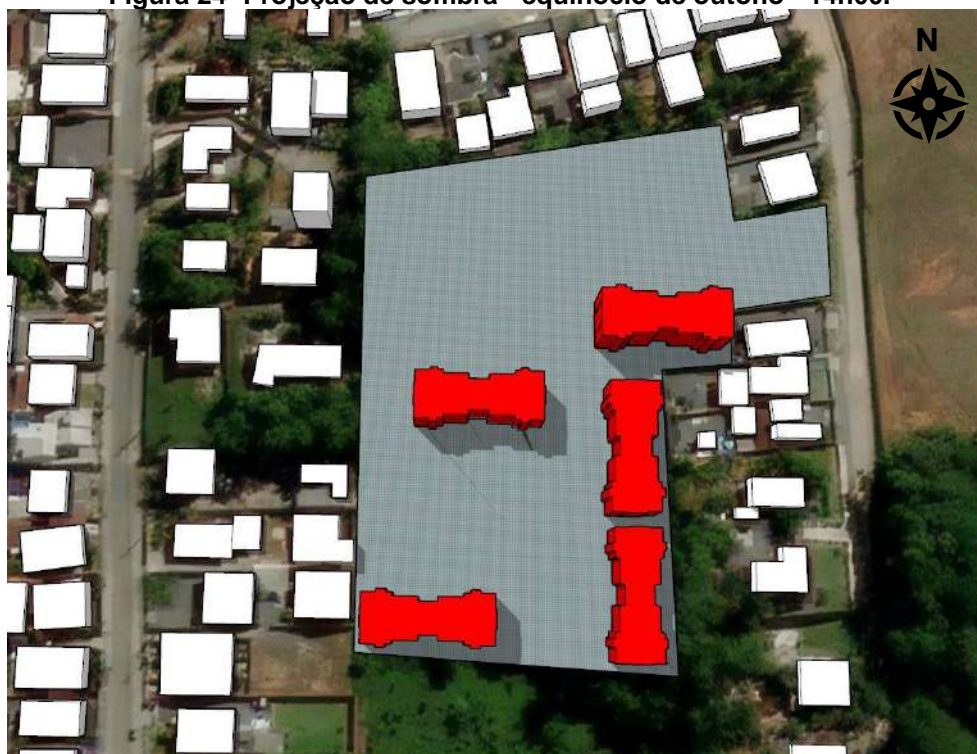
Figura 24- Projeção de sombra - equinócio de outono - 14h00.
