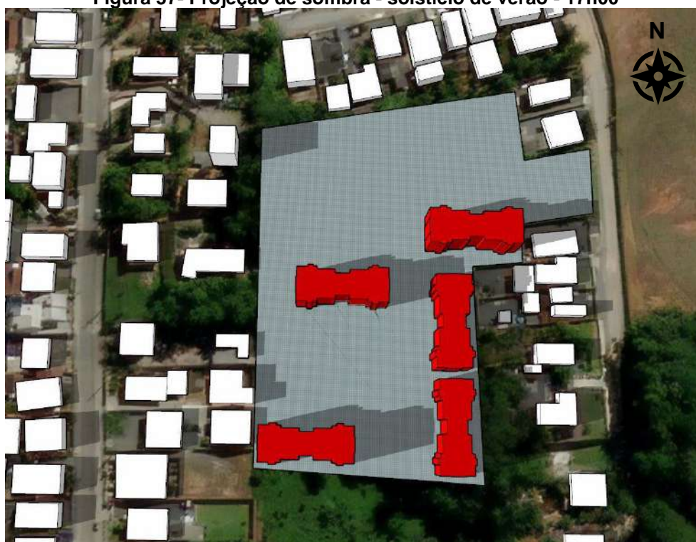
Figura 37- Projeção de sombra - solstício de verão - 17h00
