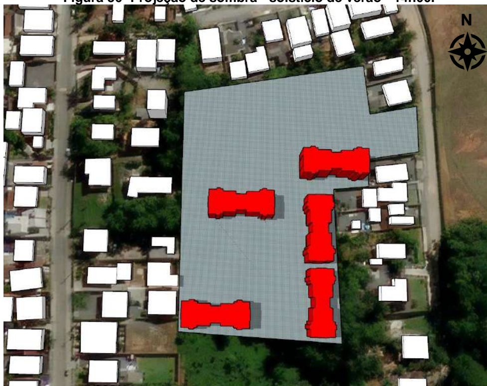
Figura 36- Projeção de sombra - solstício de verão - 14h00.
