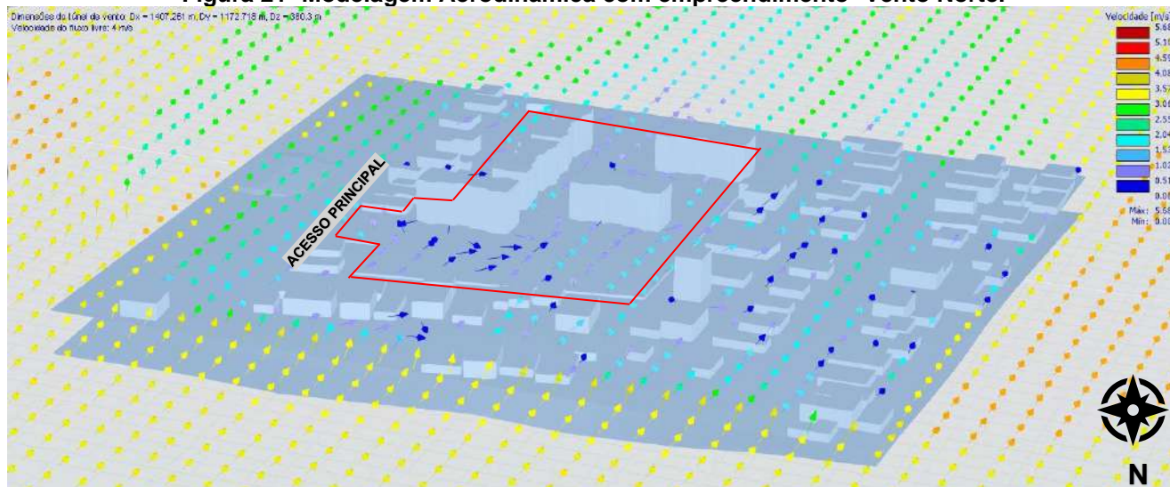
Figura 21- Modelagem Aerodinâmica com empreendimento- Vento Norte.
