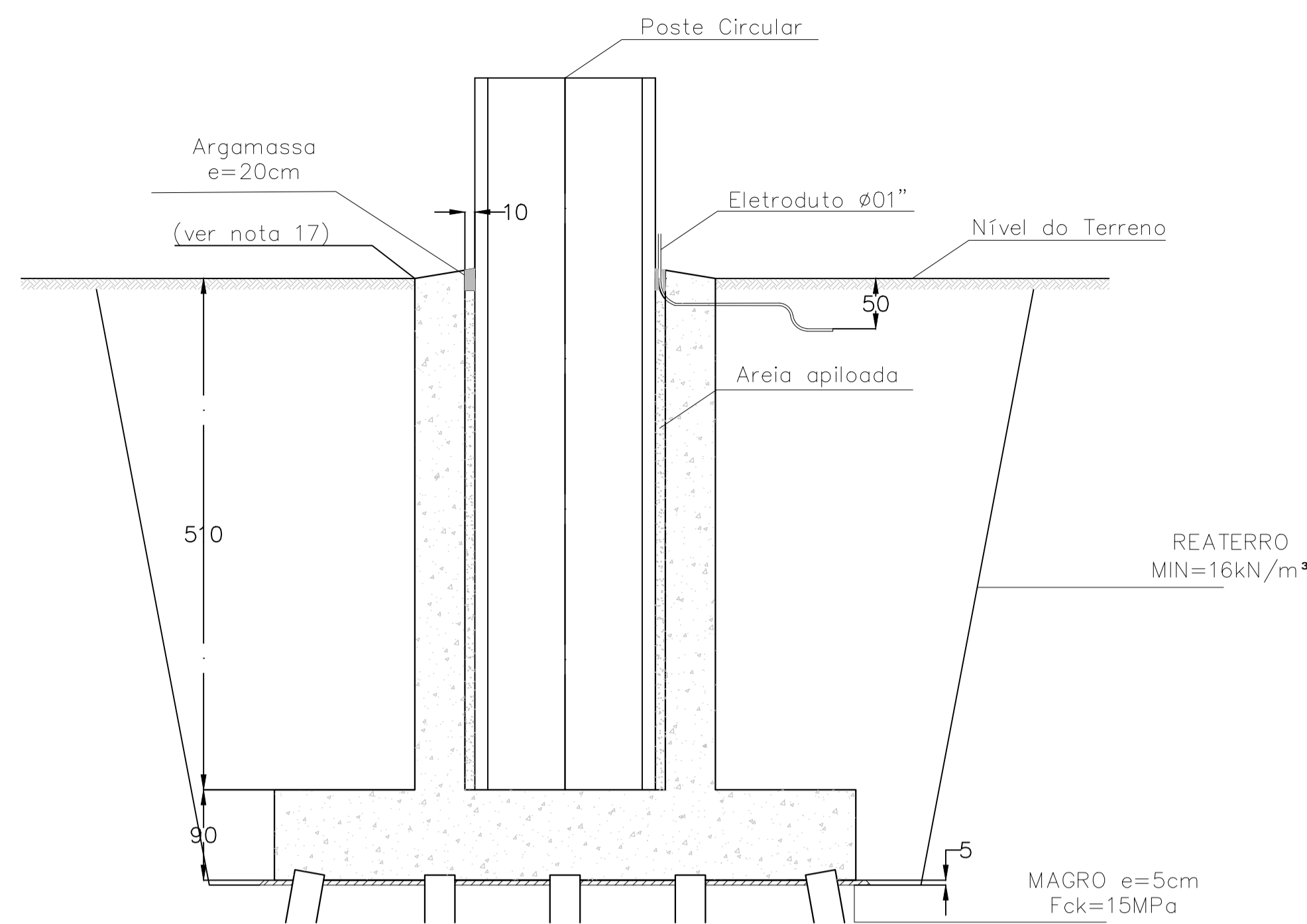
FORMA DO BLOCO - VISTA EM CORTE esc 1:50
