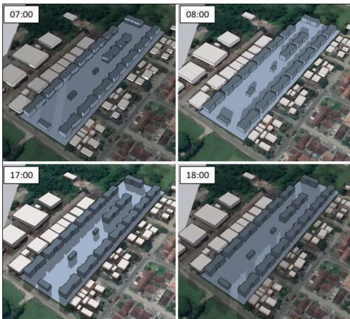
Figura 30. Compilado de imagens evidenciando o sombreamento projetado para o futuro empreendimento durante o Solstício de Inverno. Fonte: DBio, 2022.
