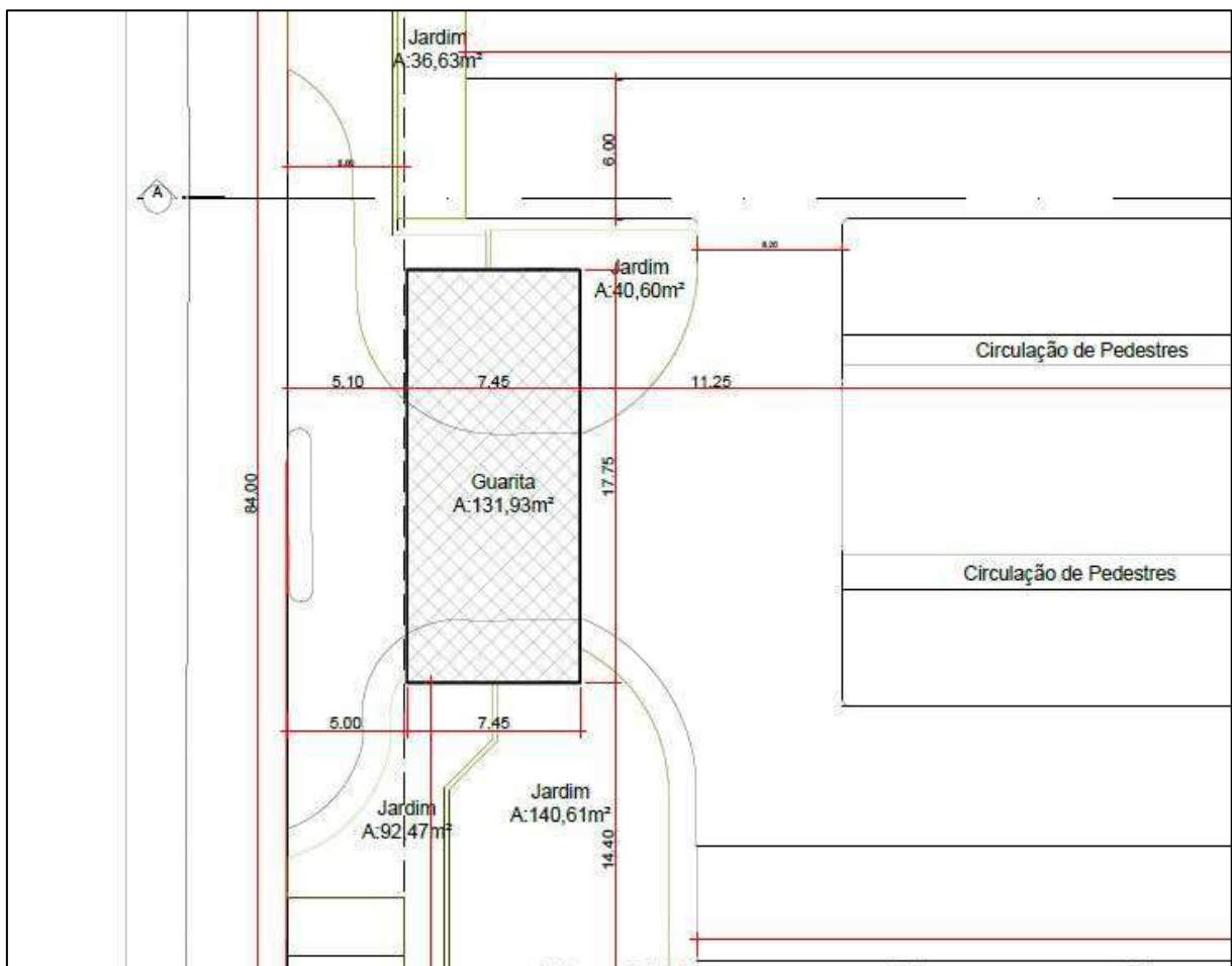
Figura 67. Recorte da planta baixa evidenciando o recuo a ser adotado para a guarita de acesso ao empreendimento. Fonte: DBio, 2022
