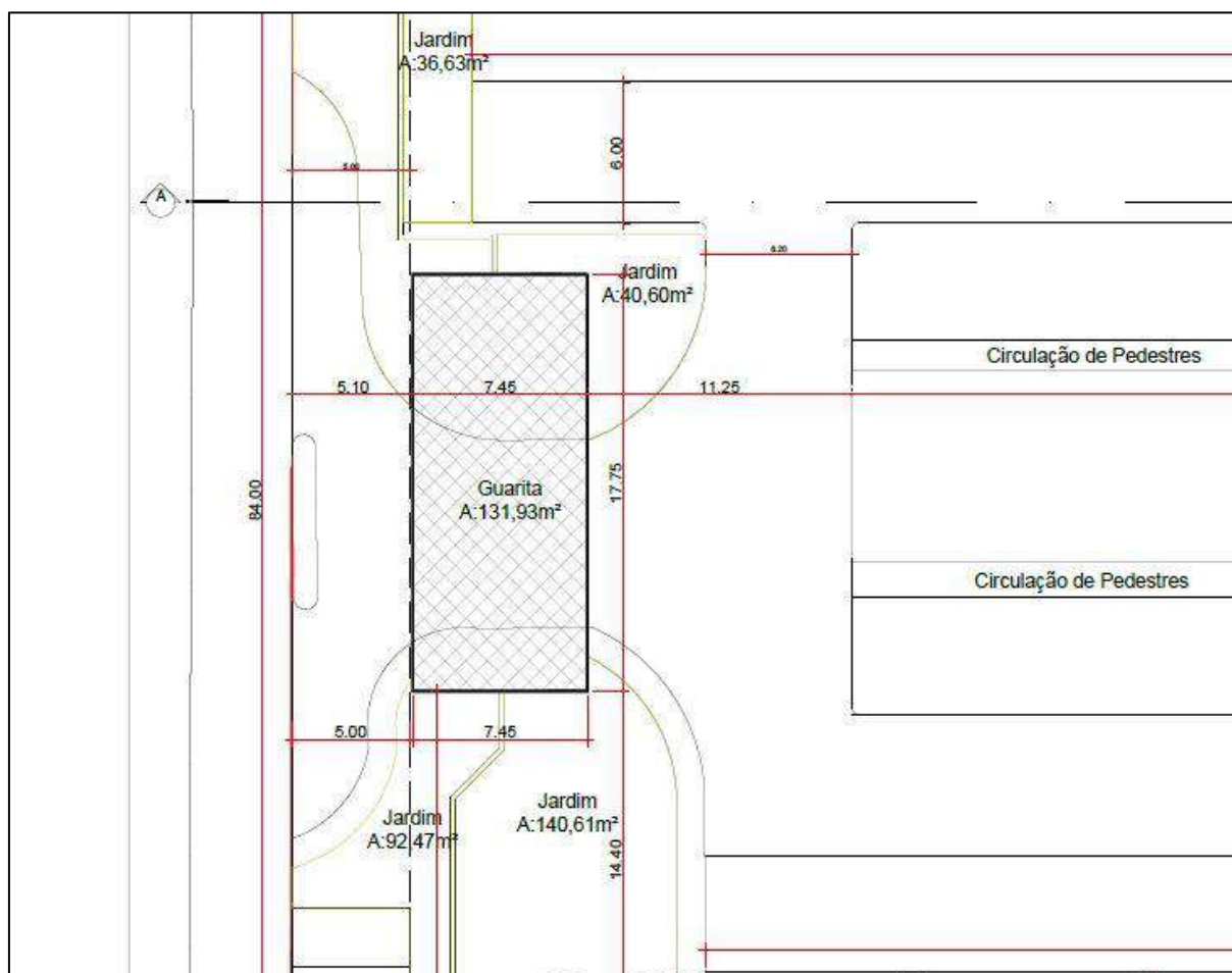
Figura 66. Recorte da planta baixa evidenciando o recuo a ser adotado para a guarita de acesso ao empreendimento. Fonte: DBio, 2022
