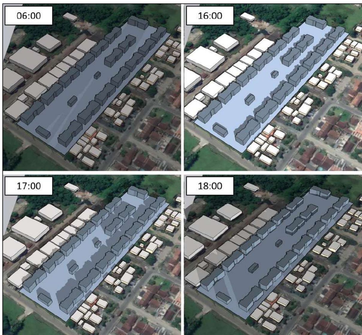
Figura 28. Compilado de imagens evidenciando o sombreamento projetado para o futuro empreendimento durante o Equinócio de Outono. Fonte: DBio, 2022.
