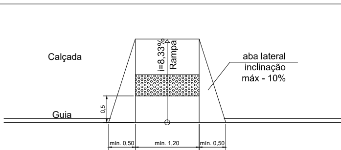
DETALHES REBAIXO CALÇADA
