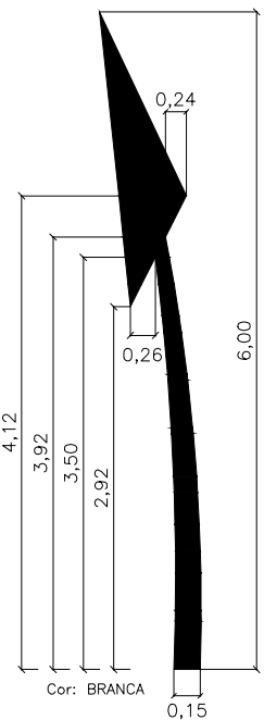
DETALHE SETA INDICATIVA DE MOVIMENTO EM CURVA
