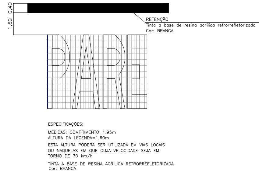
DETALHES LEGENDA "PARE"
