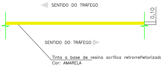
DETALHES LINHA AMARELA CONTÍNUA SIMPLES
