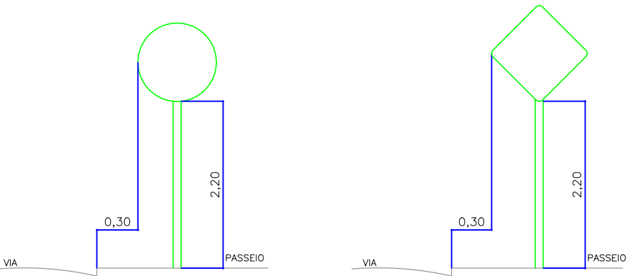
DETALHES INSTALAÇÃO DAS PLACAS
