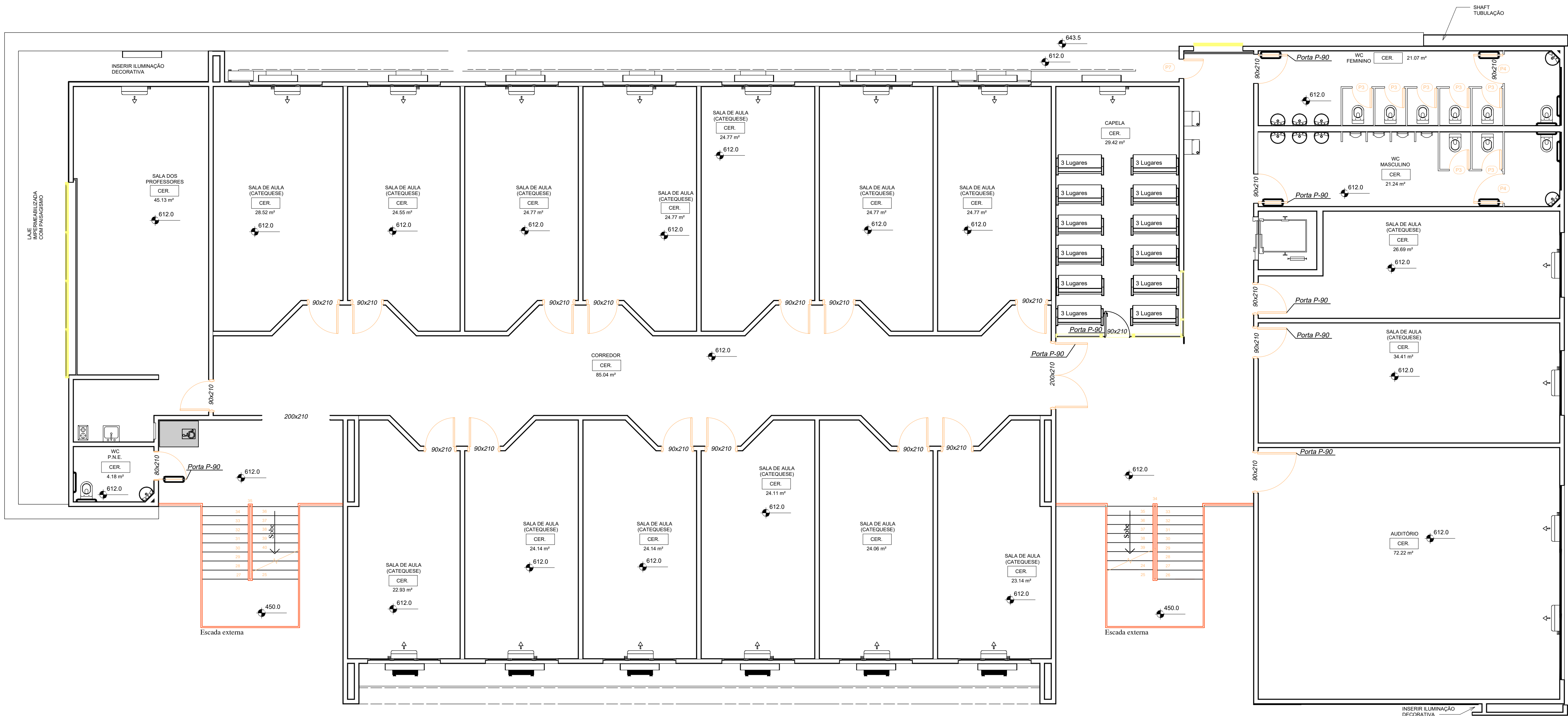
Planta Baixa - 2º Pavimento
