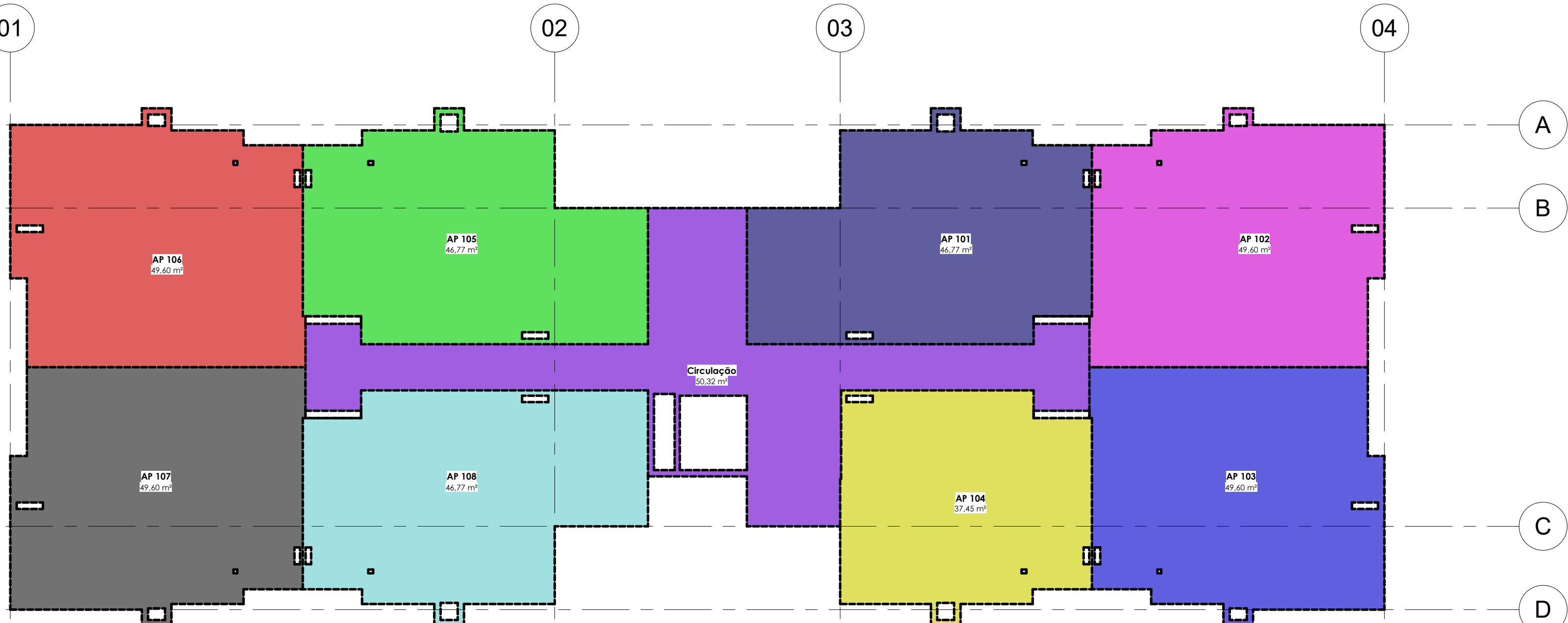
2 Planta de área térreo 1 : 100
