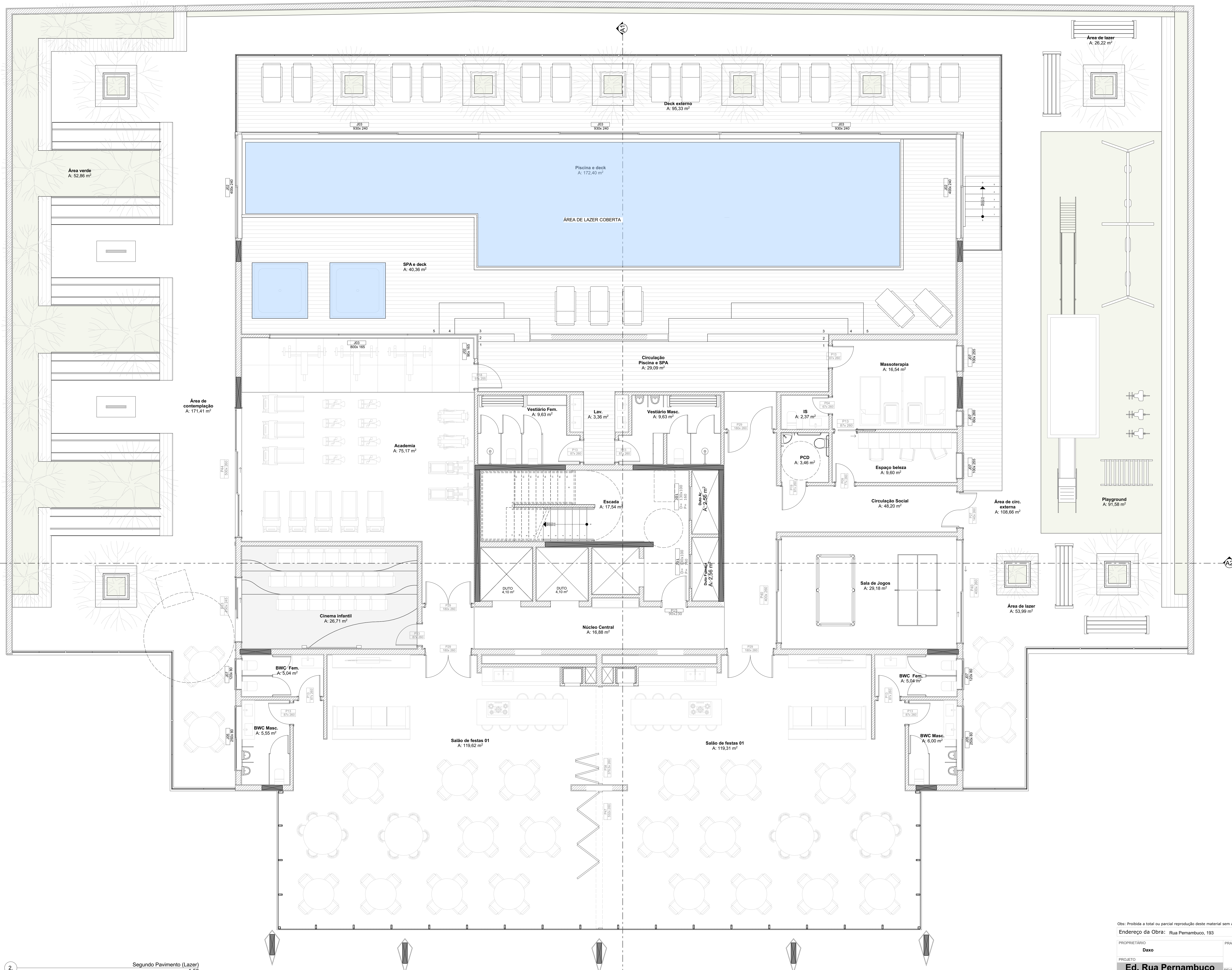
2. Segundo Pavimento (Lazer) 1:50
