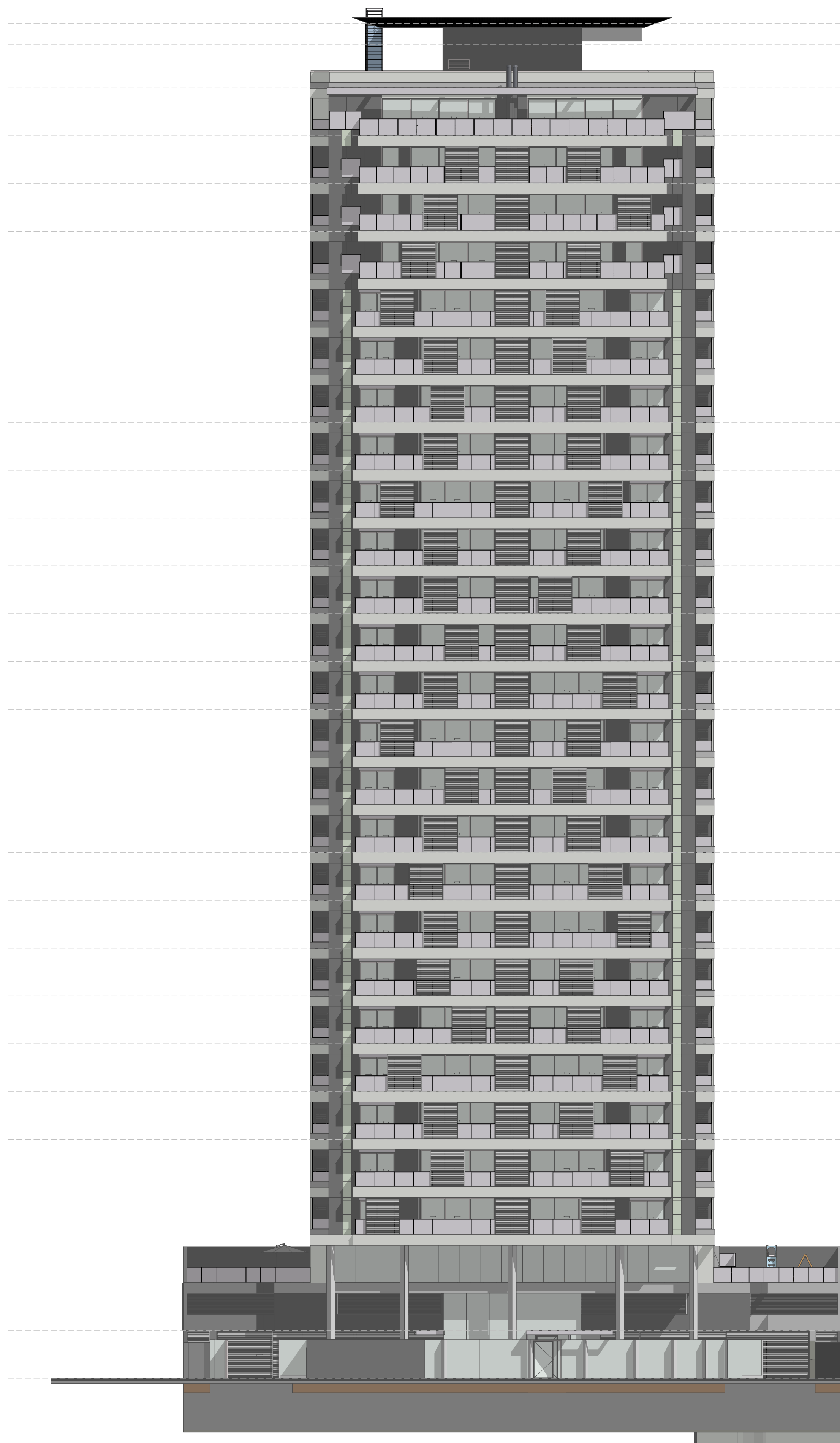
1 Elevação 1:200
