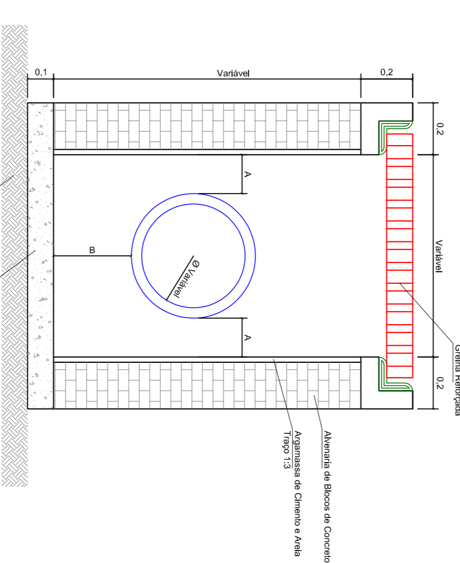
Corte AA'
