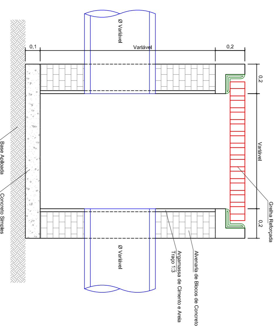
Corte BB'
