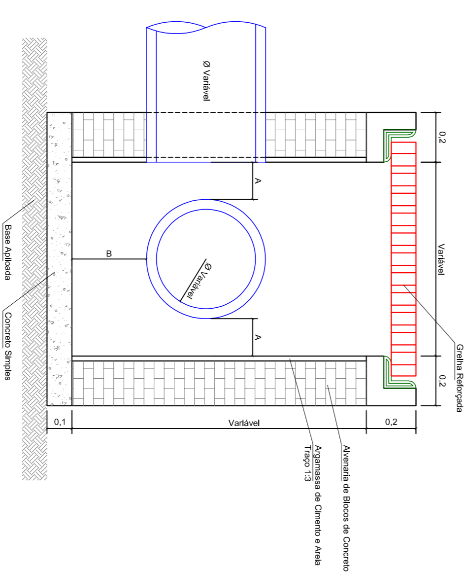
Corte BB'
