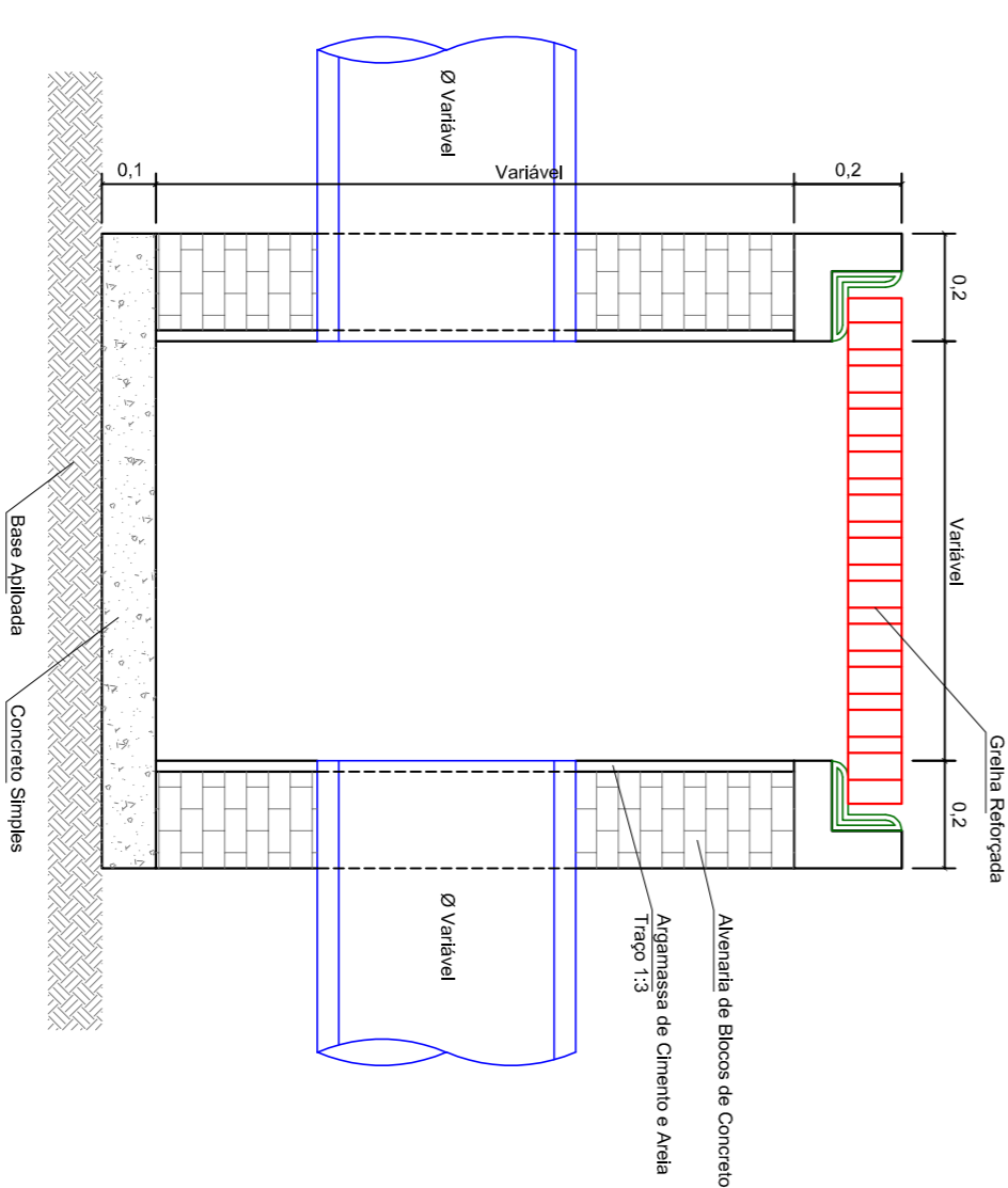
Corte BB'
