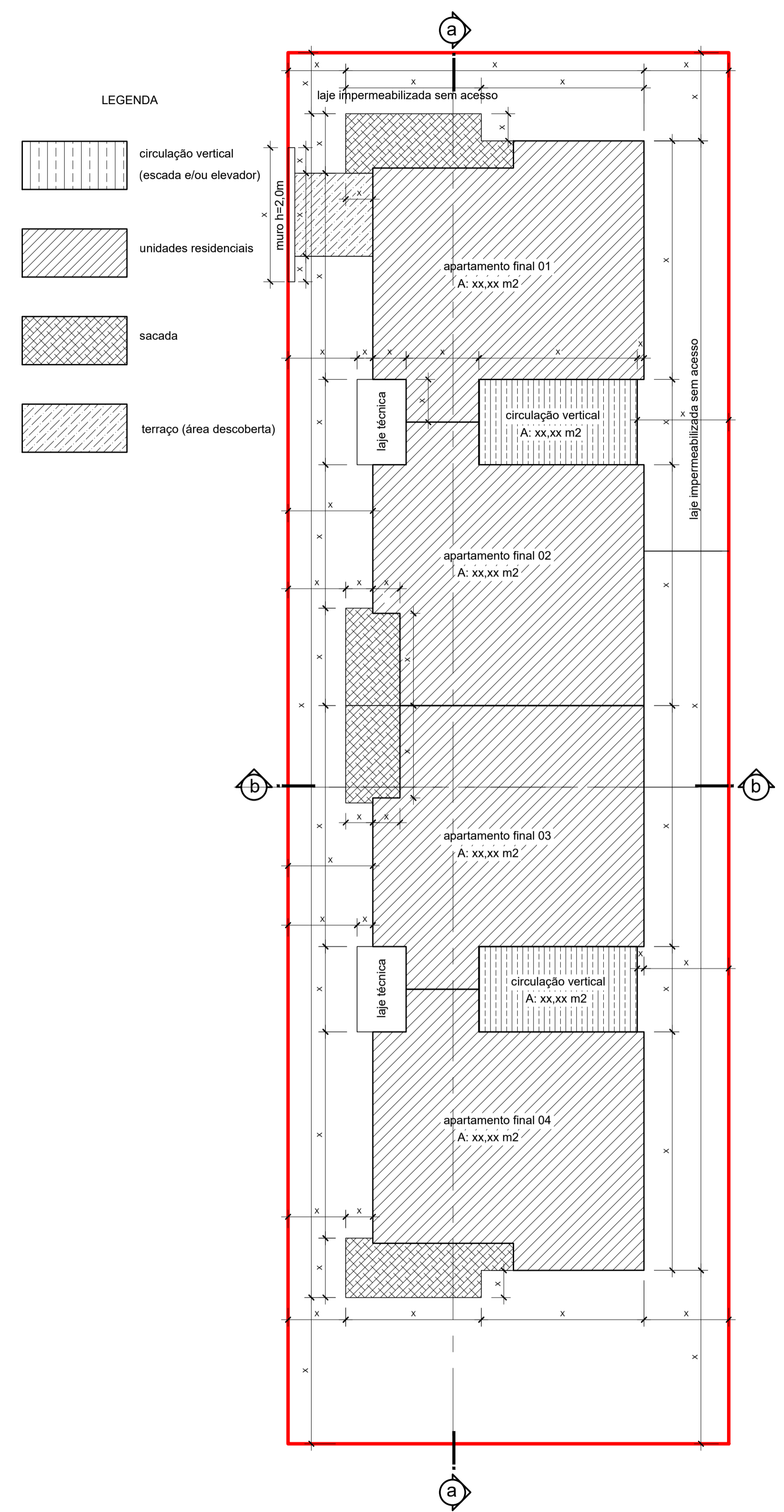
PLANTA ESQUEMÁTICA 1º PAVIMENTO ESCALA : 1/100
