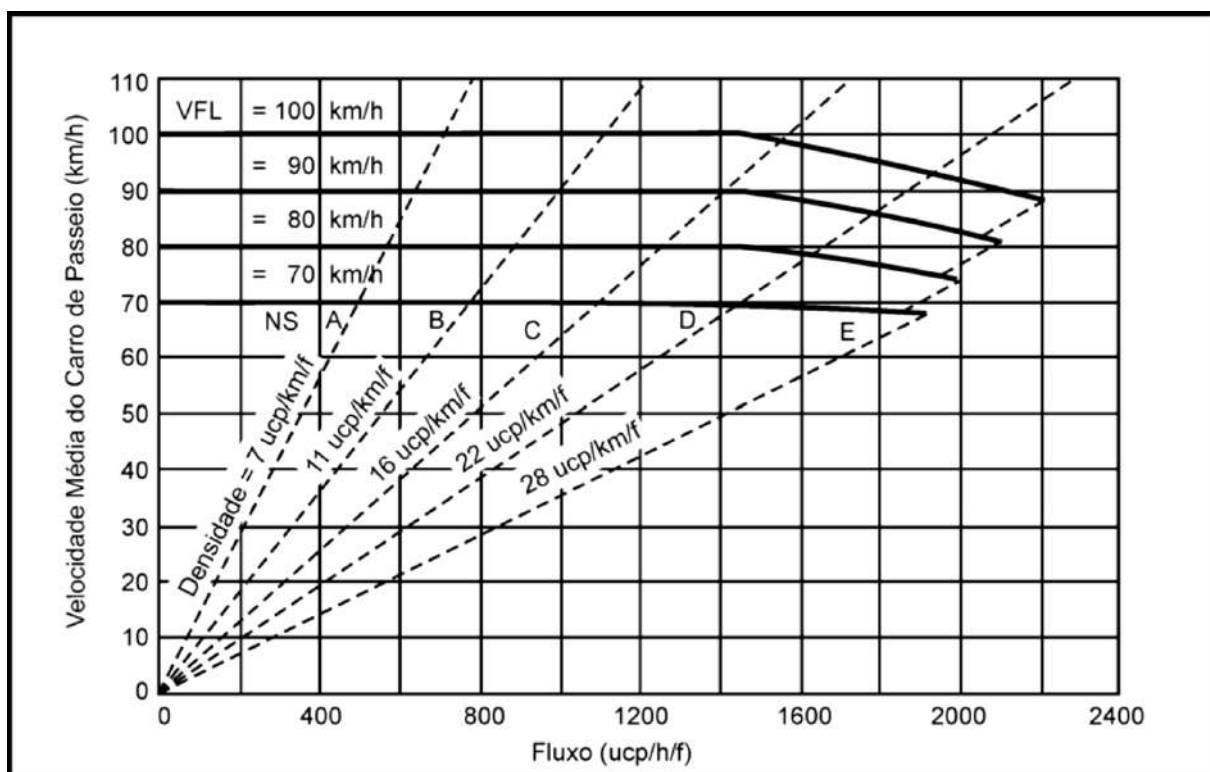
Figura 63. Âbaco de níveis de serviço. Fonte DNIT 2006.
