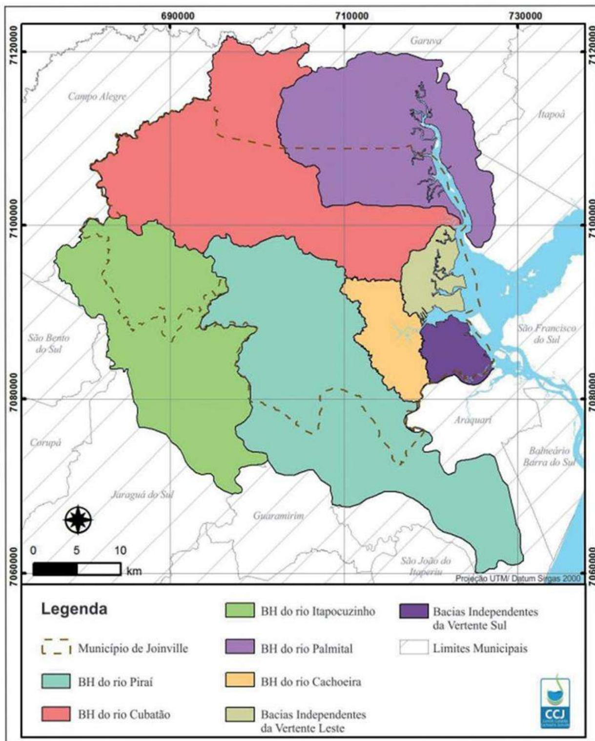
Figura 26. Bacias hidrográficas da região de Joinville. Fonte: Elaborado pelo CCJ (2016) com base em dados do IBGE, da Prefeitura de Joinville e SDS.
