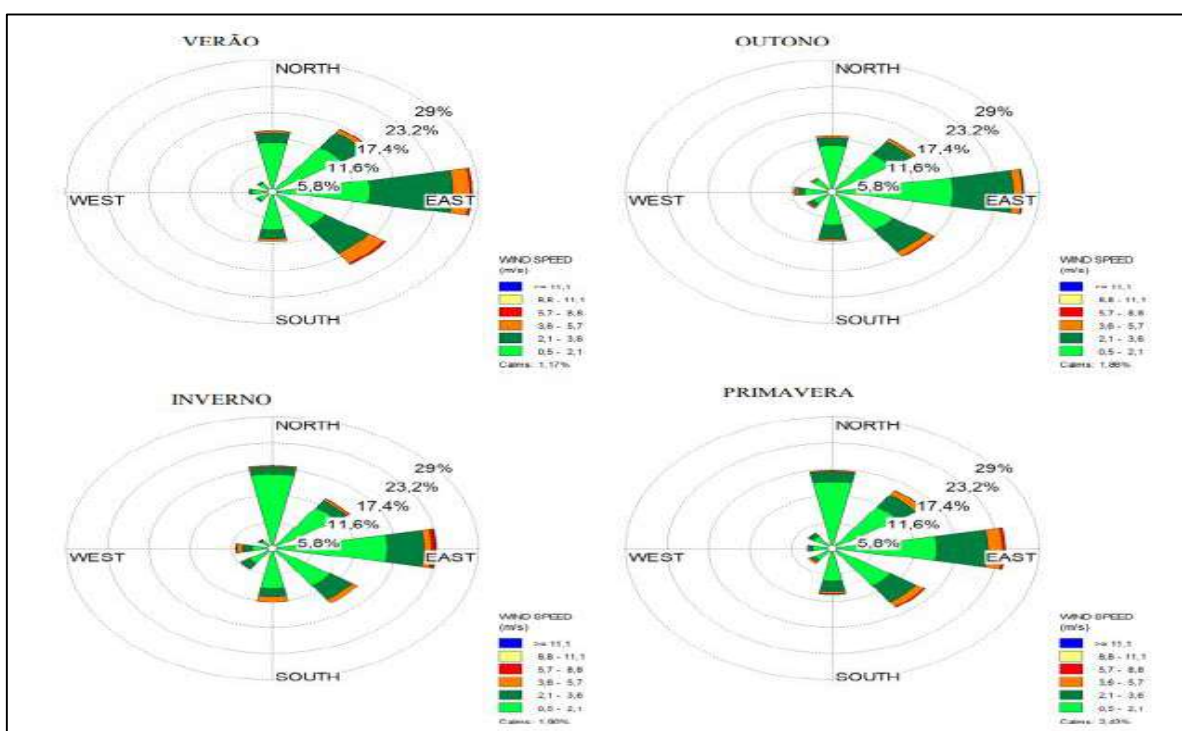
Figura 17. Rosa dos ventos das diferentes estações do ano para a estação meteorológica da Univille. Fonte: Yara de Mello, 2015.
