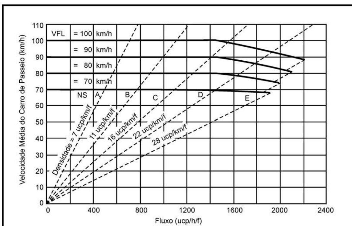
Figura 45. Ábaco de níveis de serviço. Fonte DNIT 2006.
