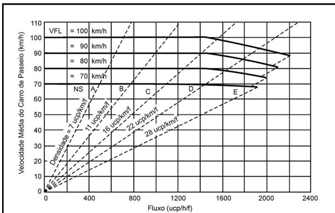
Figura 36. Ábaco de níveis de serviço. Fonte DNIT 2006.
