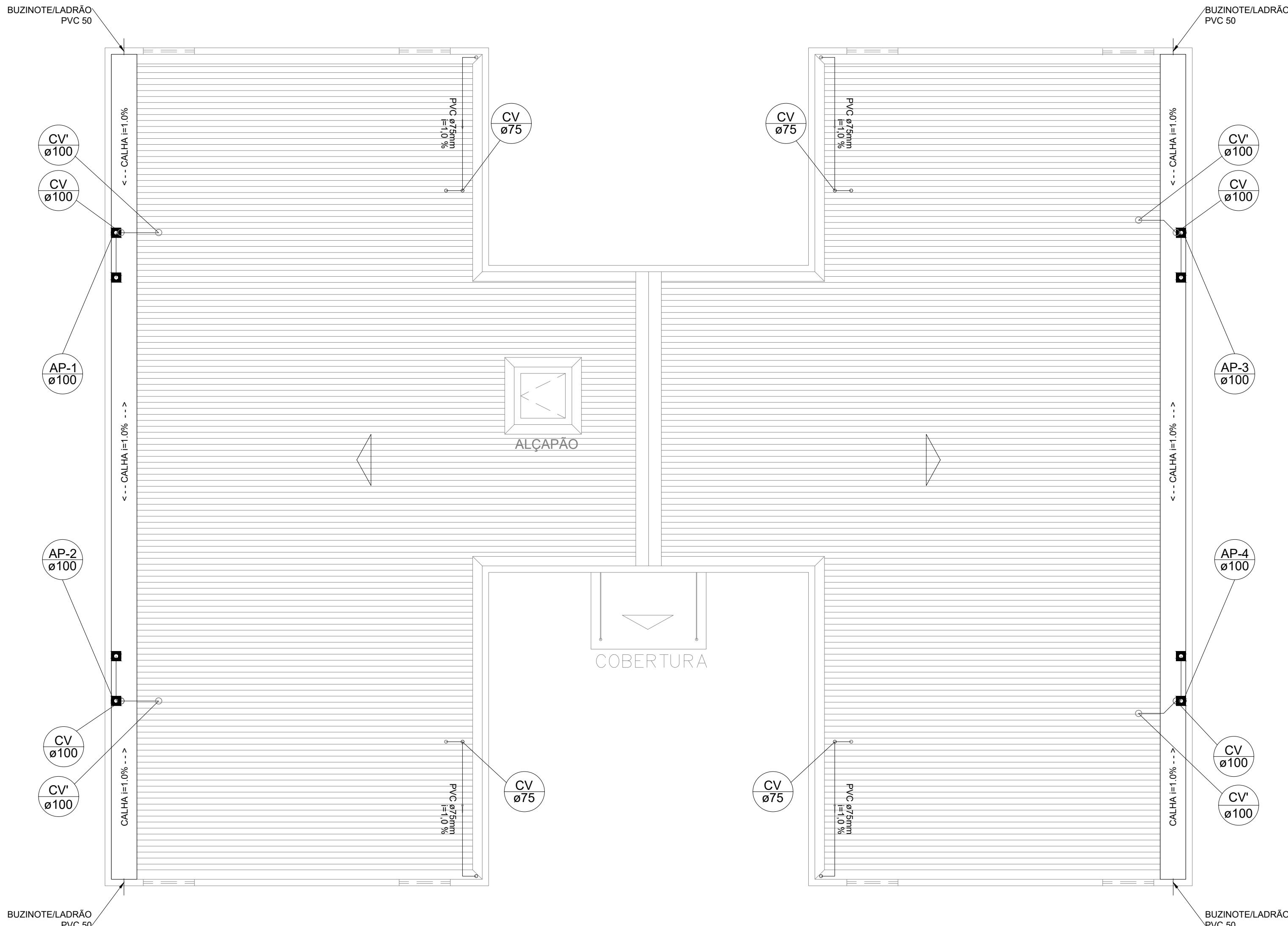
PLANTA COBERTURA - BLOCOS 01 AO 15 ESCALA 1:50
