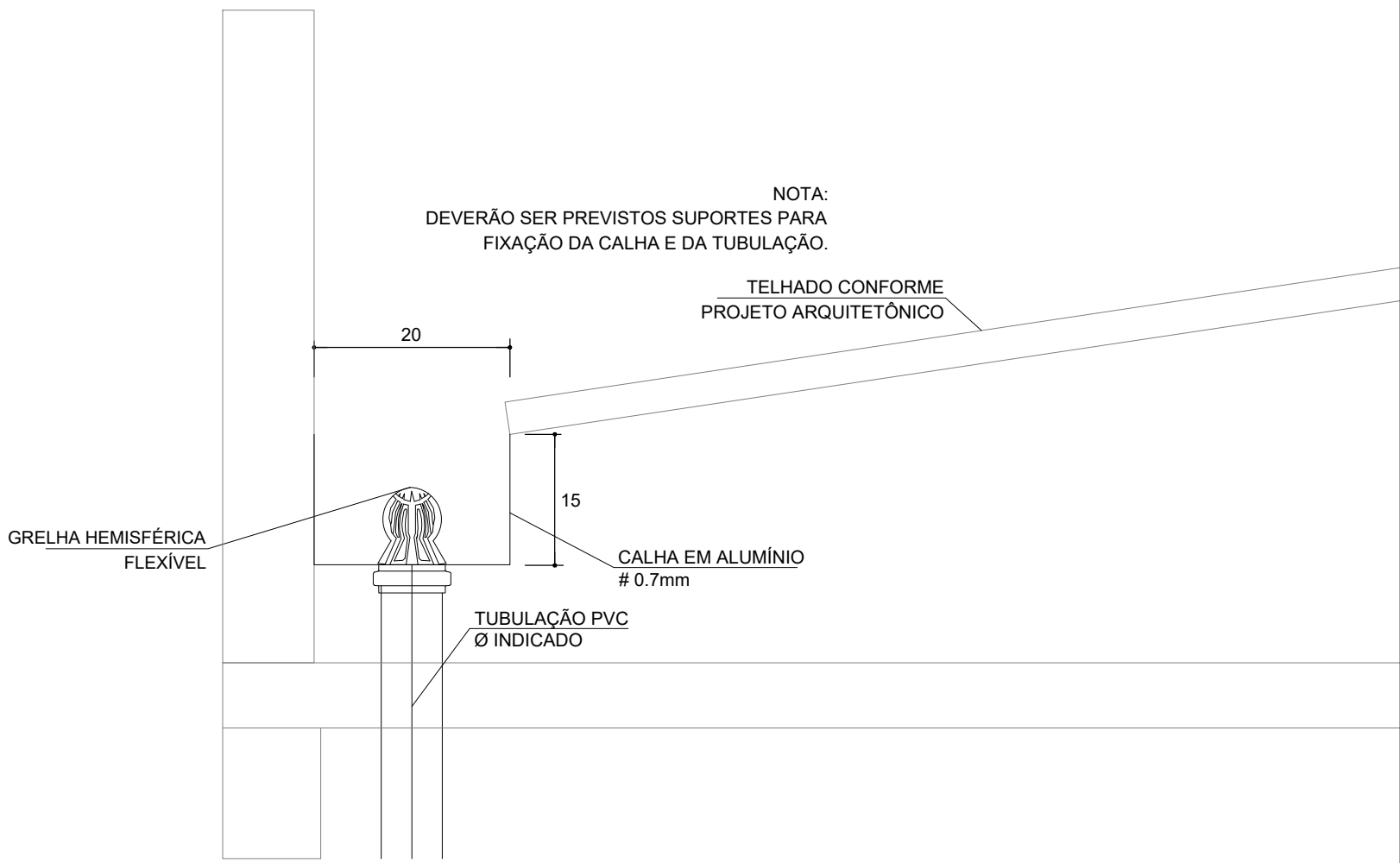
DETALHE GÊNÉRICO DE 02 PONTOS DE CAPTAÇÃO DE AGUAS PLUVIAIS NA CALHA
