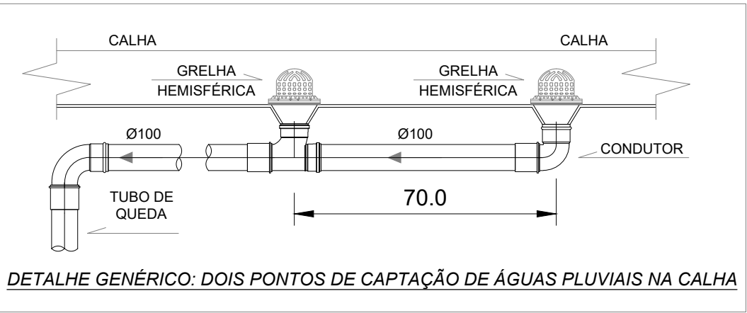
DETALHE GÊNÉRICO DE 02 PONTOS DE CAPTAÇÃO DE AGUAS PLUVIAIS NA CALHA
