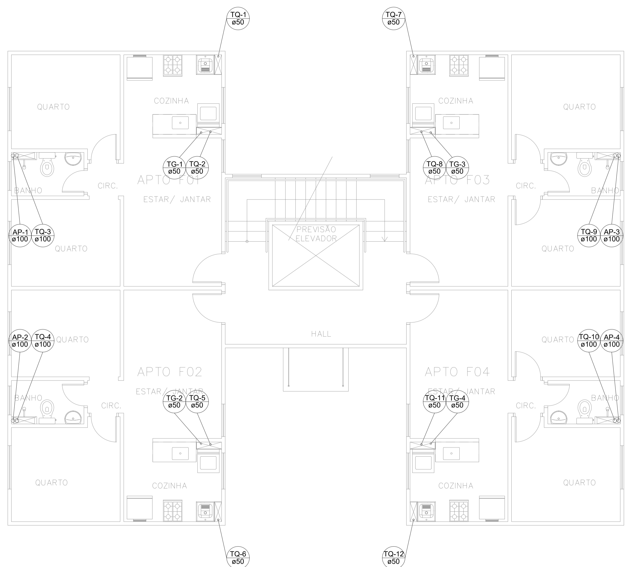
PLANTA DE CAPTAÇÃO DE ESGOTO E ÁGUAS PLUVIAIS - PAV. TIPO BLOCOS 01 AO 15 ESCALA 1:50
