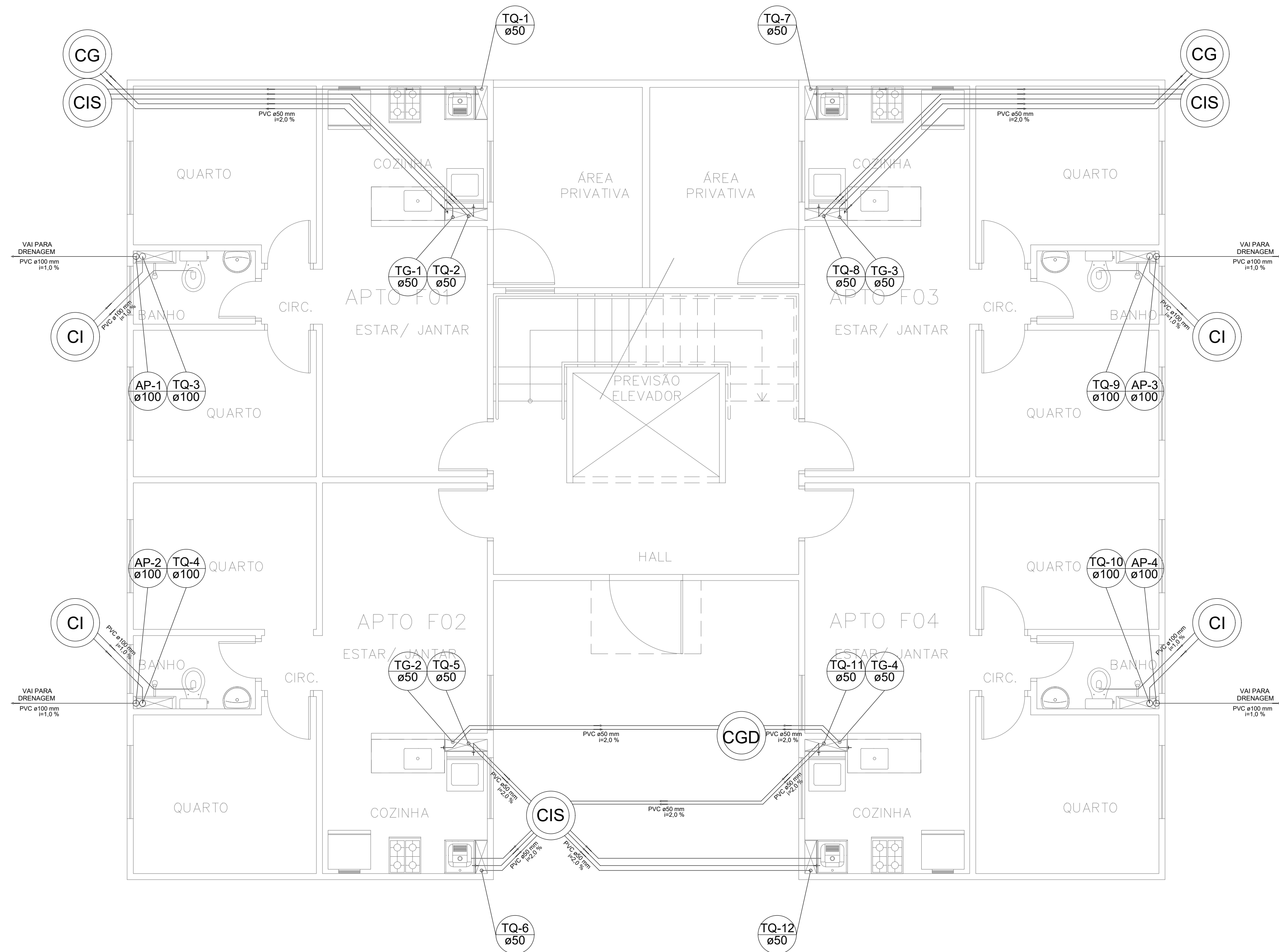
PLANTA DE CAPTAÇÃO DE ESGOTO E ÁGUAS PLUVIAS - PAV. TÉRREO BLOCO 01 ESCALA 1:50
